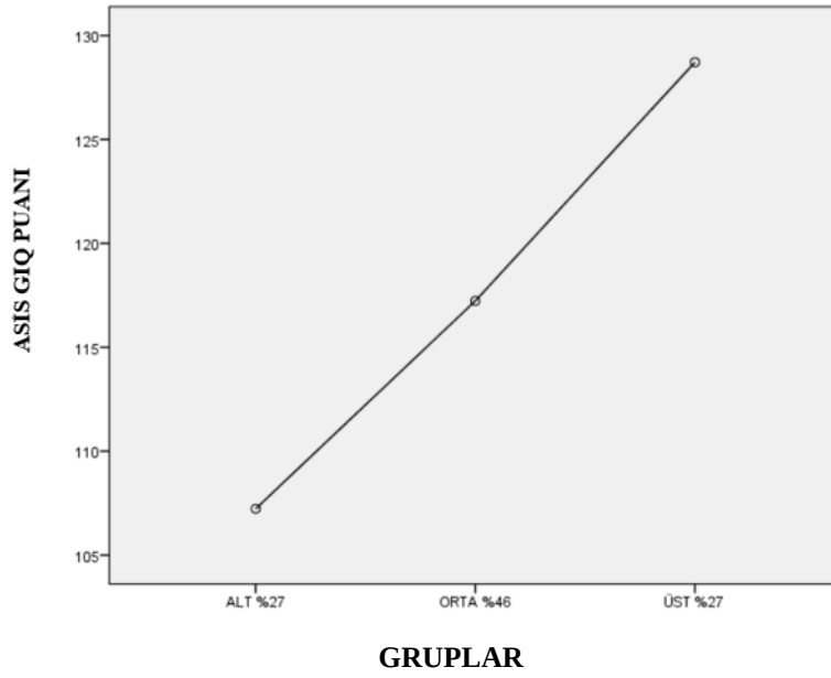
Şekil 4.1. Yüzdelik grupların genel zekâ puanları
