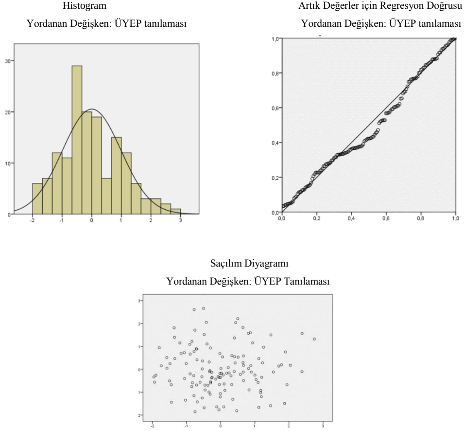
Şekil 4.1 Artık değerler için regresyon doğrusu, histogram ve saçılım diyagramı
