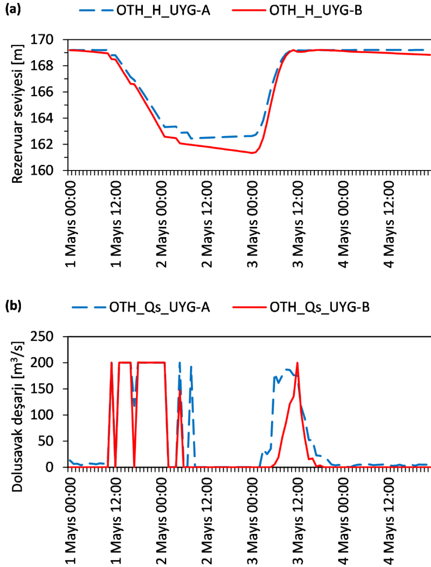
Şekil 5.4 OTH kapalı-döngü işletme sonuçlarının türbinsiz sistemle karşılaştırılması (a) Rezervuar seviye değişimi (m) (b) Dolusavak deşarjlar ( \text{m}^3/\text{s} )
