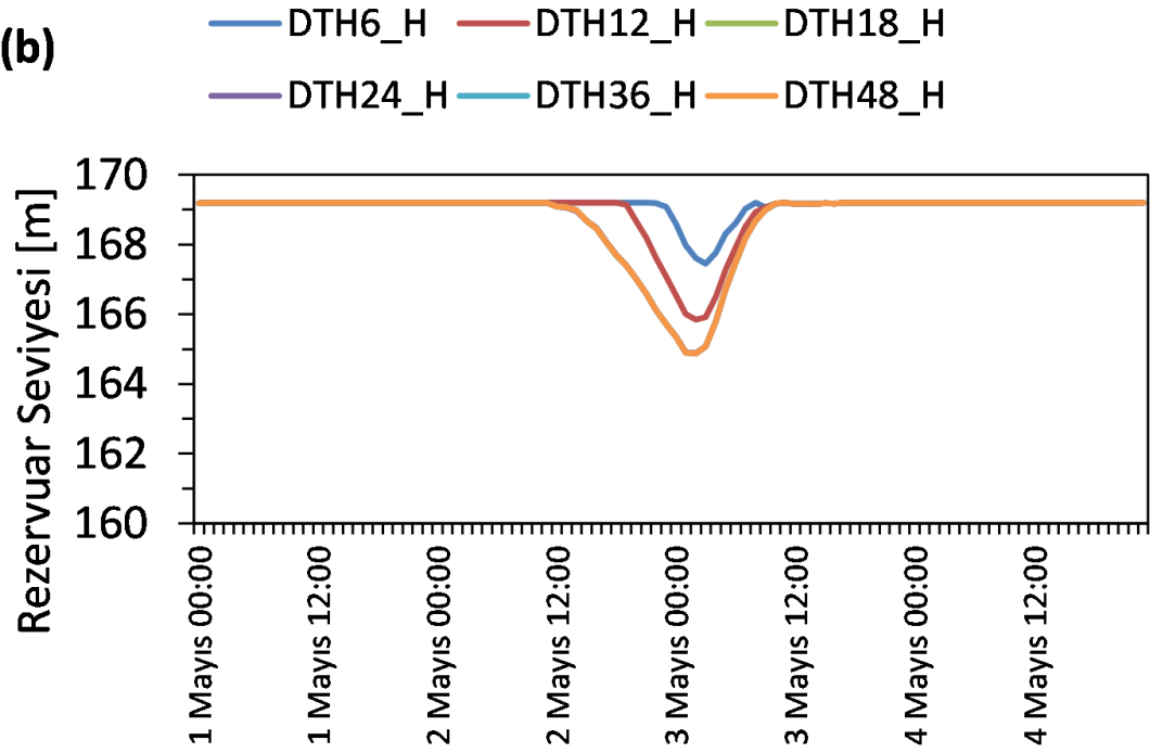
Şekil 4.19 DAT ile hindcast denemeleri tahmin ufku performansının karşılaştırılması (Senaryo-01) (a)
