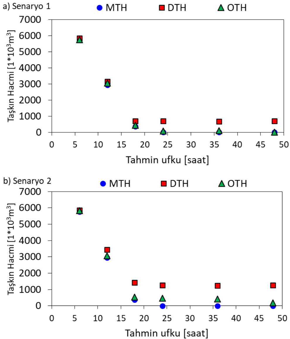
Şekil 4.26 Bağımsız 5 farklı senaryo için MTH, DTH ve OTH testlerine ait “mansap kanalından taşan hacim [ 1000 \text{ m}^3 ]” performans değerlendirme sonuçları
