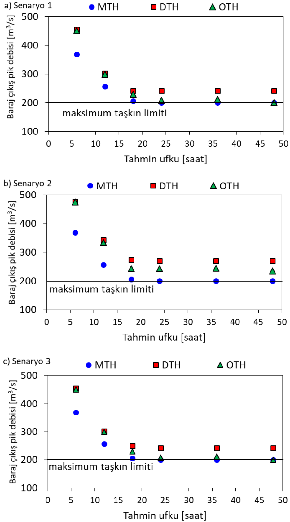
Şekil 4.25 Bağımsız 5 farklı senaryo için MTH, DTH ve OTH testlerine ait pik dolusavak deşarj [ m^3/s ] performans değerlendirme sonuçları
