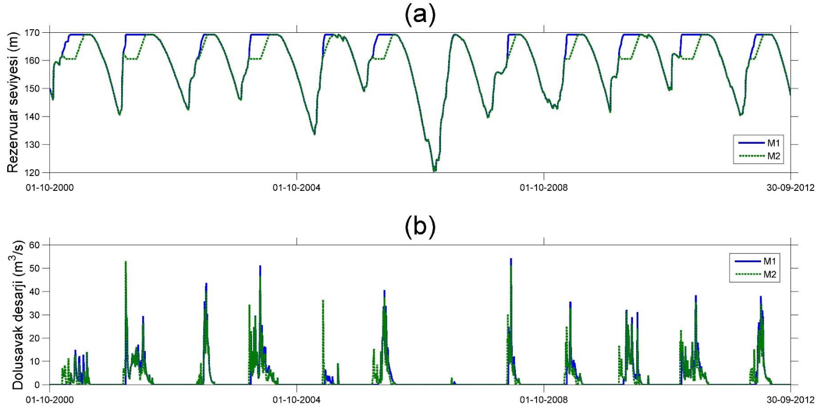
Şekil 4.10 M1 ve M2 modellerinin karşılaştırması (a) Rezervuar seviyesi [m] (b) Dolusavak deşarjı [ \text{m}^3/\text{s} ]
