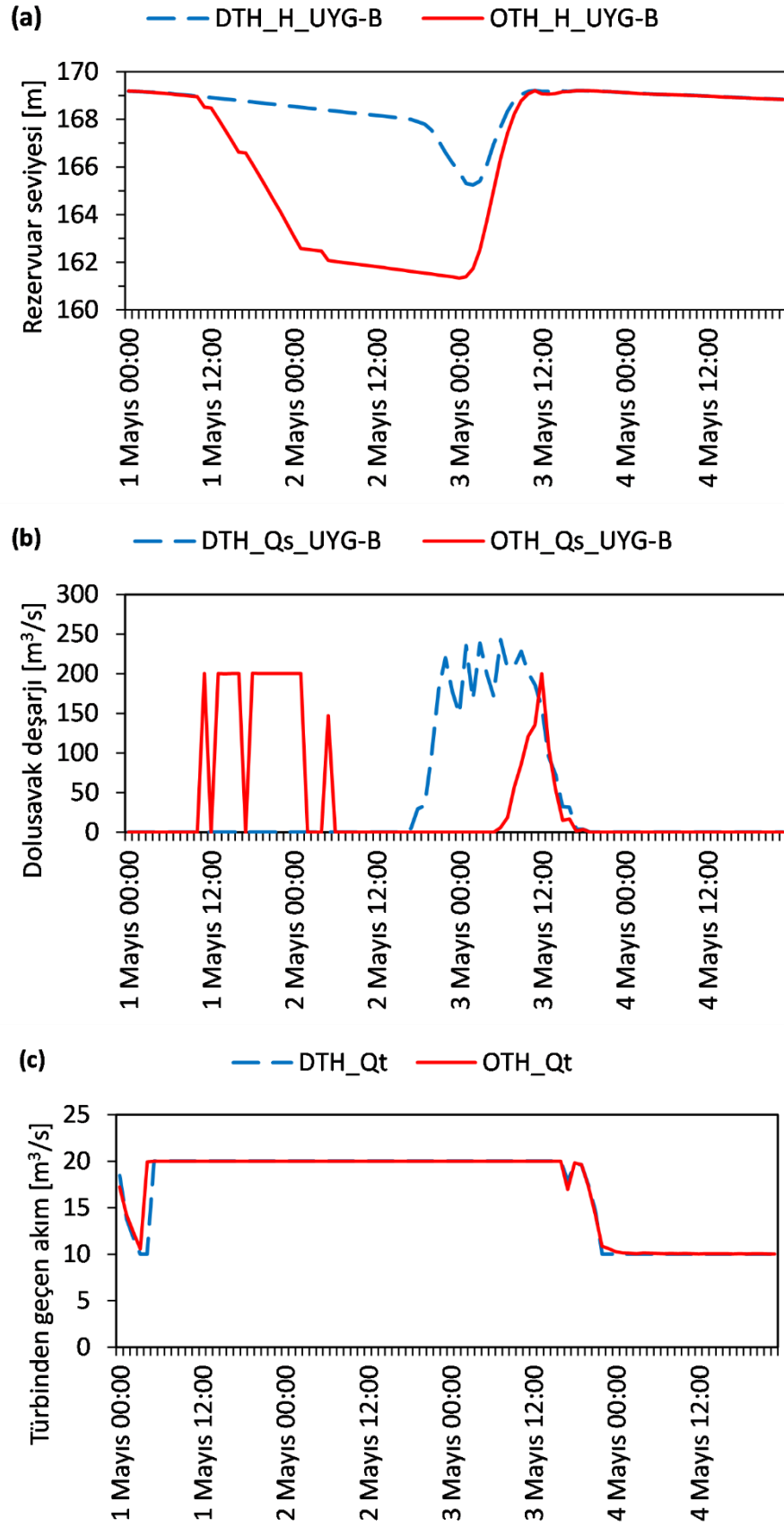
Şekil 5.2 UYG-A ve UYG-B karşılaştırmalı DTH ve OTH sonuçları (a) Rezervuar seviye değişimi (m) (b) Dolusavak deşarjları ( m^3/s ) (c) Türbinden bırakılan akım ( m^3/s )
