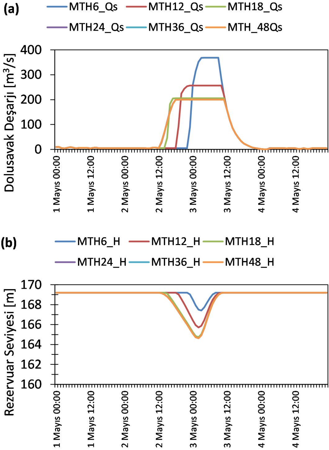
Şekil 4.18 MT ile hindcast testleri (MTH) tahmin ufku performanslarının karşılaştırılması a) Dolusavak deşarjı [ \text{m}^3/\text{s} ] b) Rezervuar seviyesi [m]
