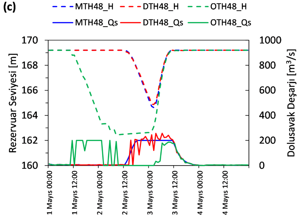
Şekil 4.24 Üç farklı kurulumda (MTH, DTH, OTH) ve farklı tahmin ufkuna göre rezervuar seviyesi [m] ve dolusavak deşarjlarının [ \text{m}^3/\text{s} ] karşılaştırılması (Senaryo 01) (a) 24 saat, (b) 36 saat, (c) 48 saat
