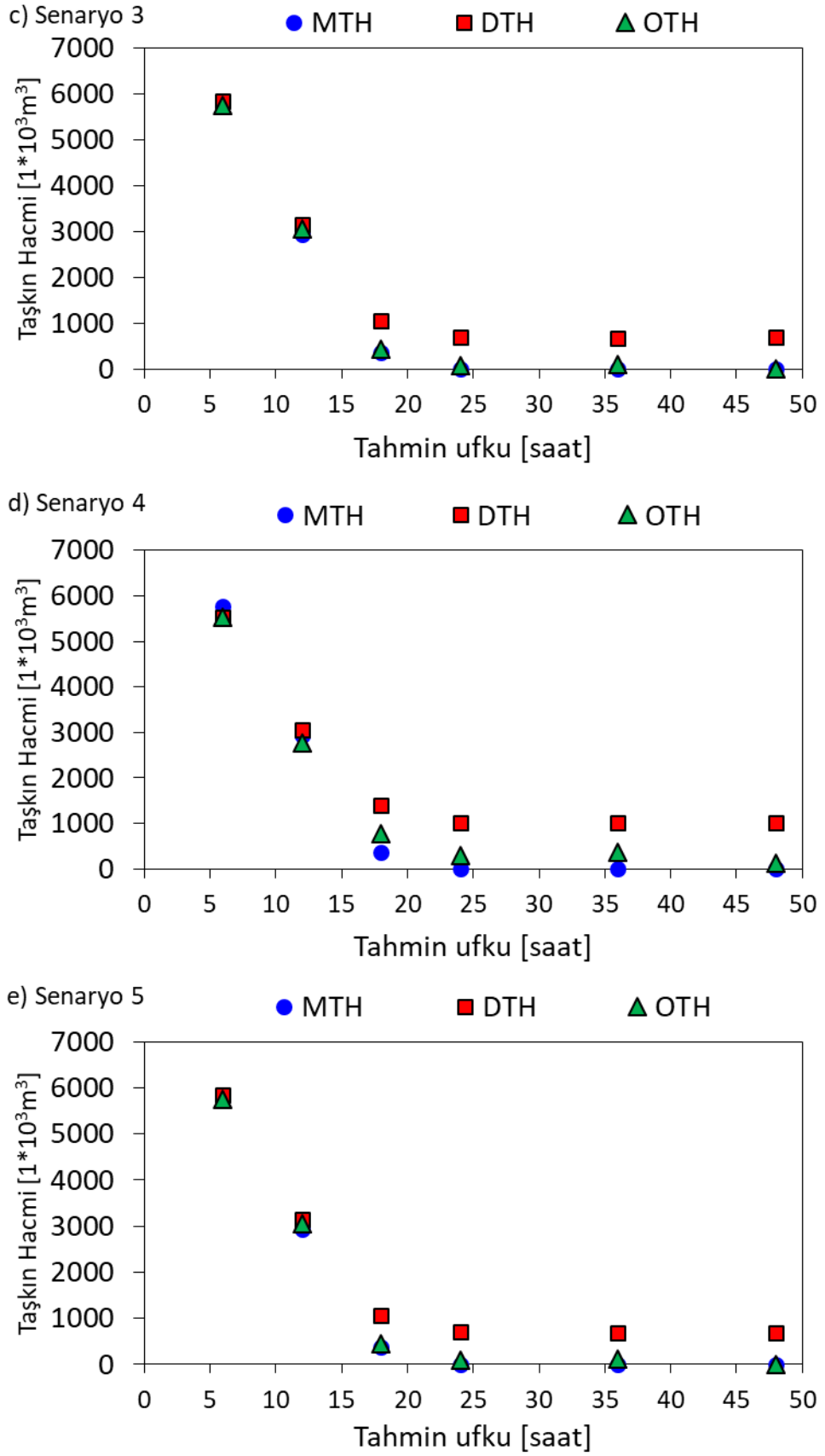
Şekil 4.26 (Devam) Bağımsız 5 farklı senaryo için MTH, DTH ve OTH testlerine ait “mansap kanalından taşan hacim [ 1000 m^3 ]” performans değerlendirme sonuçları
