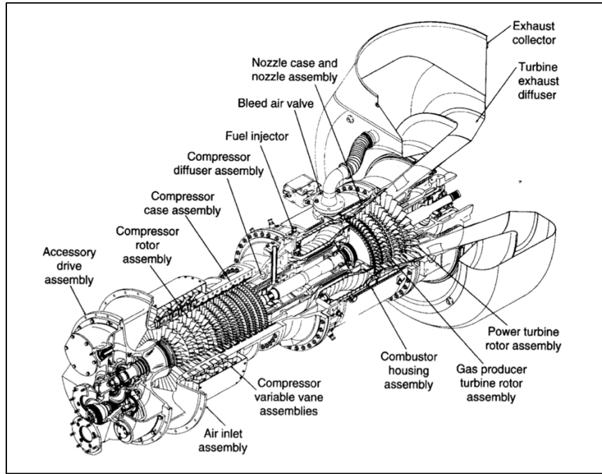
Görsel 3.14. Gemi gaz türbini (Hunt, 1999)
