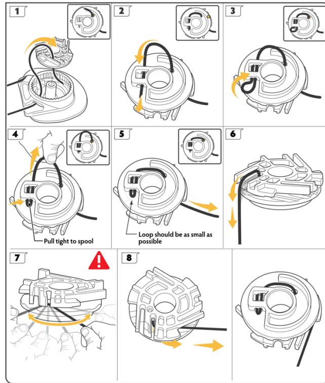
Görsel 3.15. Üretim Talimatı Bağcığın Bobine Eklenmesi ( https://fordillustration.com/Instructional-Illustration ) (Erişim Tarihi: 13.9.2018)
