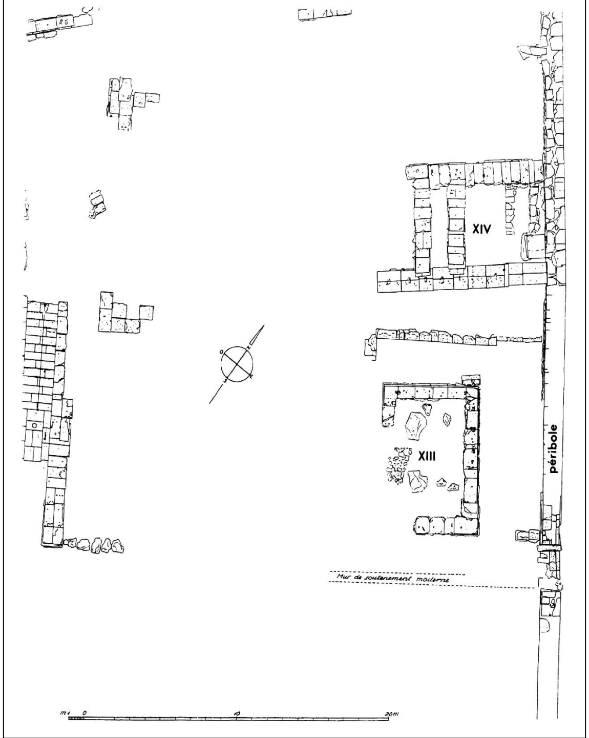
Görsel 76: XIII ve XIV numaralı thesauros lar ile doğu peribolos planı. Laroche, 1988, fig. 1.
