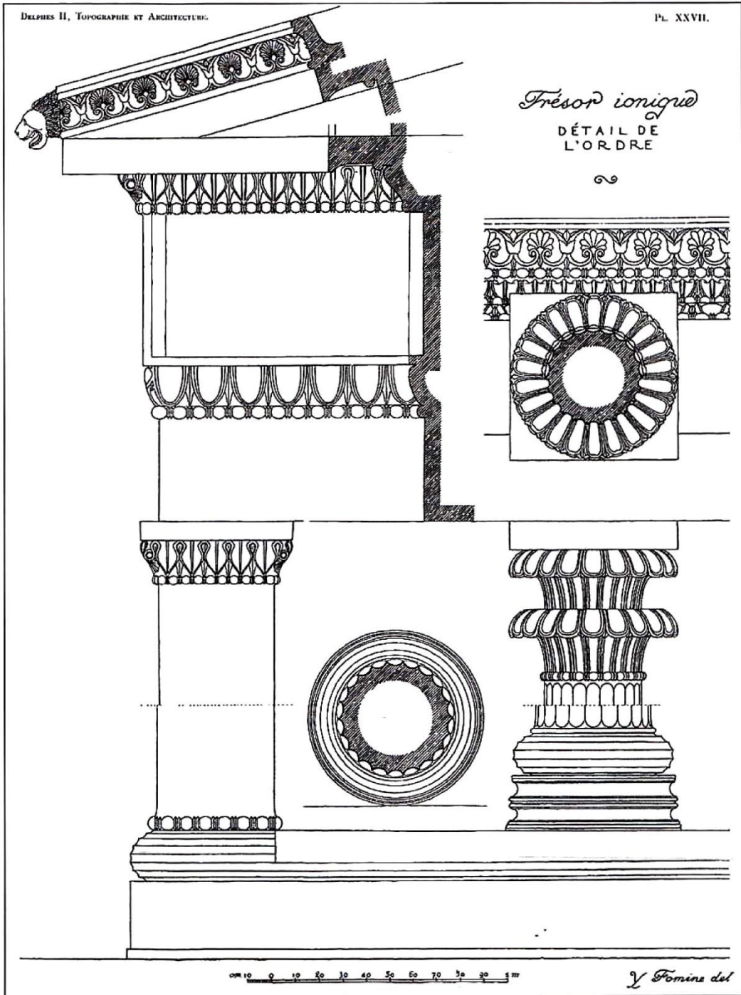
Görsel 78: Massalia thesaurosü detay çizimleri. Laroche, 2013; Çizimler: Youri Fomine.
