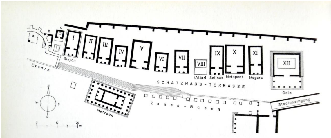
Görsel 16: Olympia thesaurosları planı. a-c: Kült yapıları.
