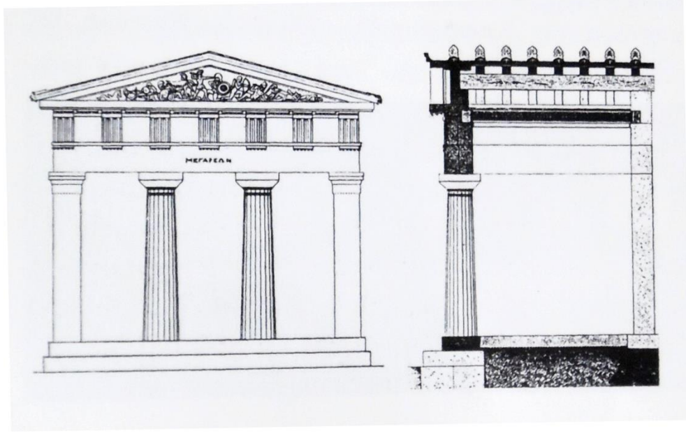
Görsel 42: Megara thesaurosü önden görünüm ve kesit çizimi.
