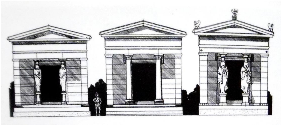
Görsel 61: Knidos, Massalia ve Siphnos thesauros ları ön cepheleri. Gruben, 2001, fig. 59. Ölçü yaklaşık olarak: 1:300.
