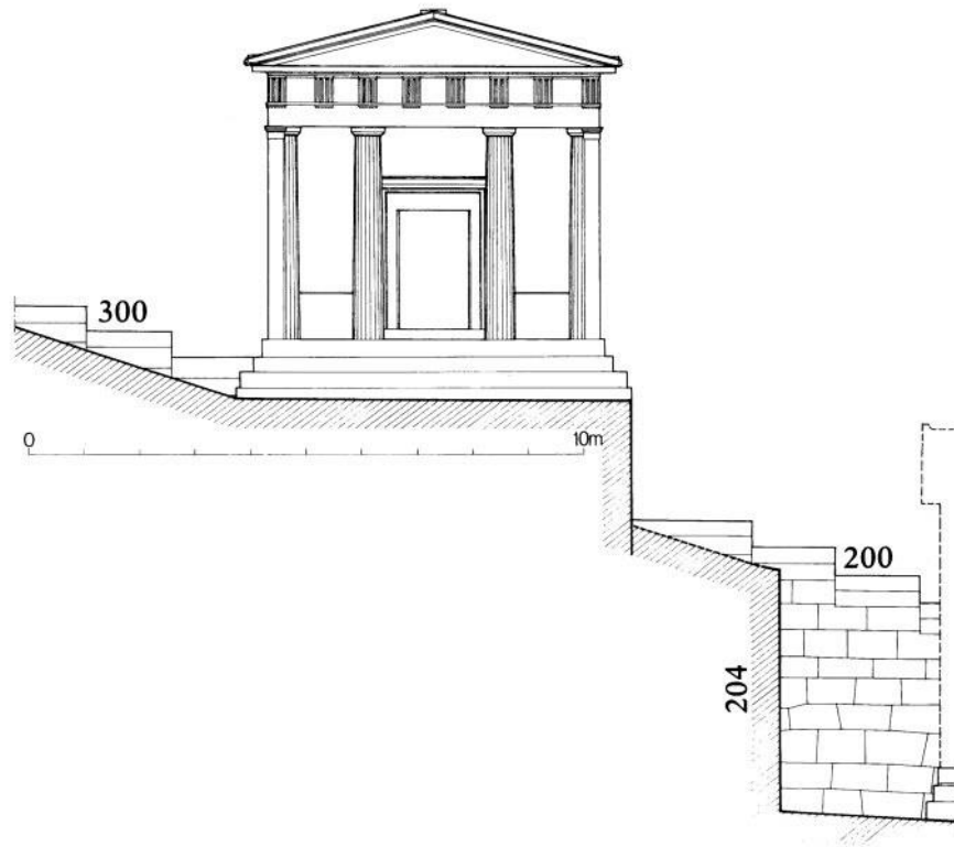
Görsel 77: Kyrene (XIV) thesauros. Bommelaer and Laroche, 1991, s. 156, fig. 62.
