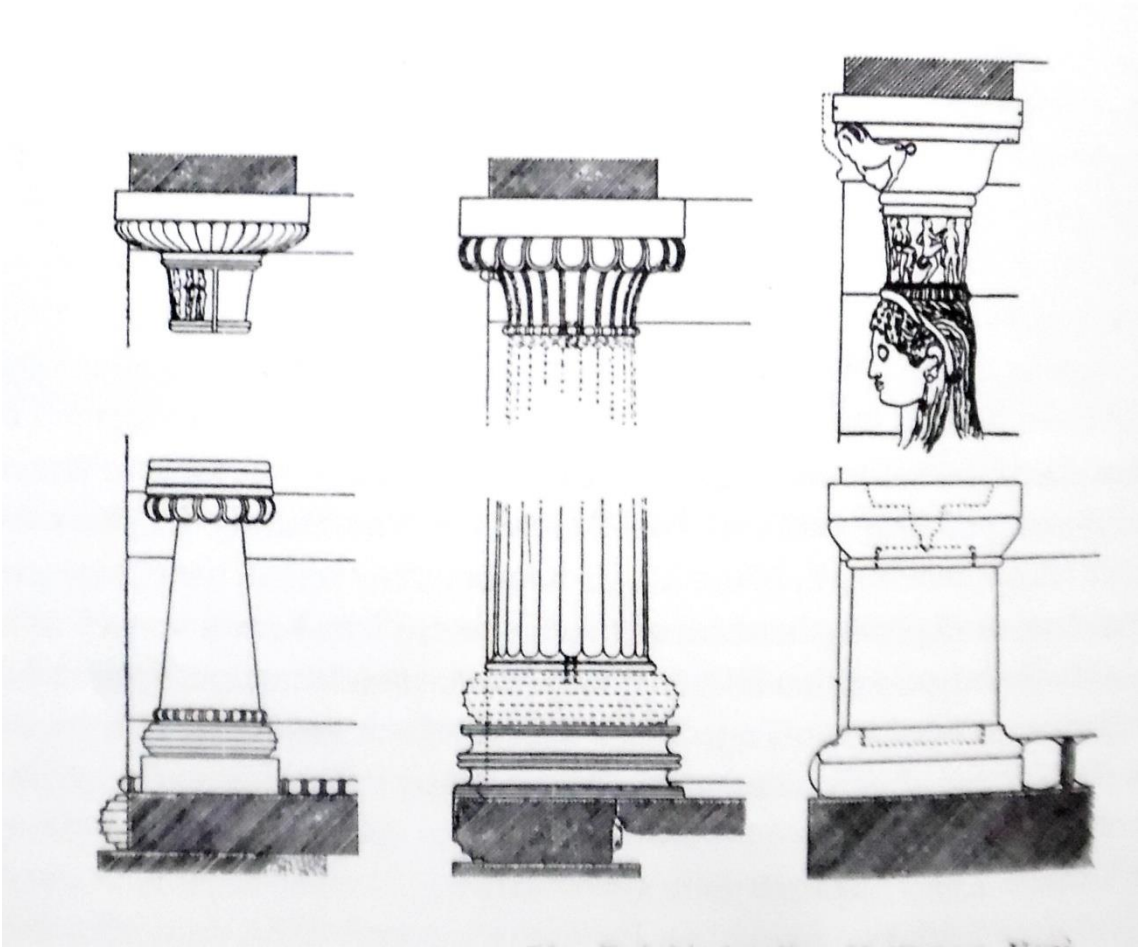
Görsel 62: Knidos, Massalia ve Siphnos thesauros ları sütun ları. Gruben, 2001, fig. 61.
