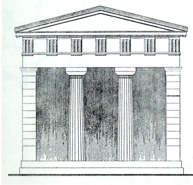
Görsel 24: Sikyon thesauros'u rekonstrüksiyonu.
