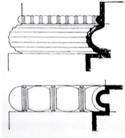
Görsel 63: Knidos ve Siphnos thesauros larının temel profilleri. Gruben, 2001, fig. 62.
