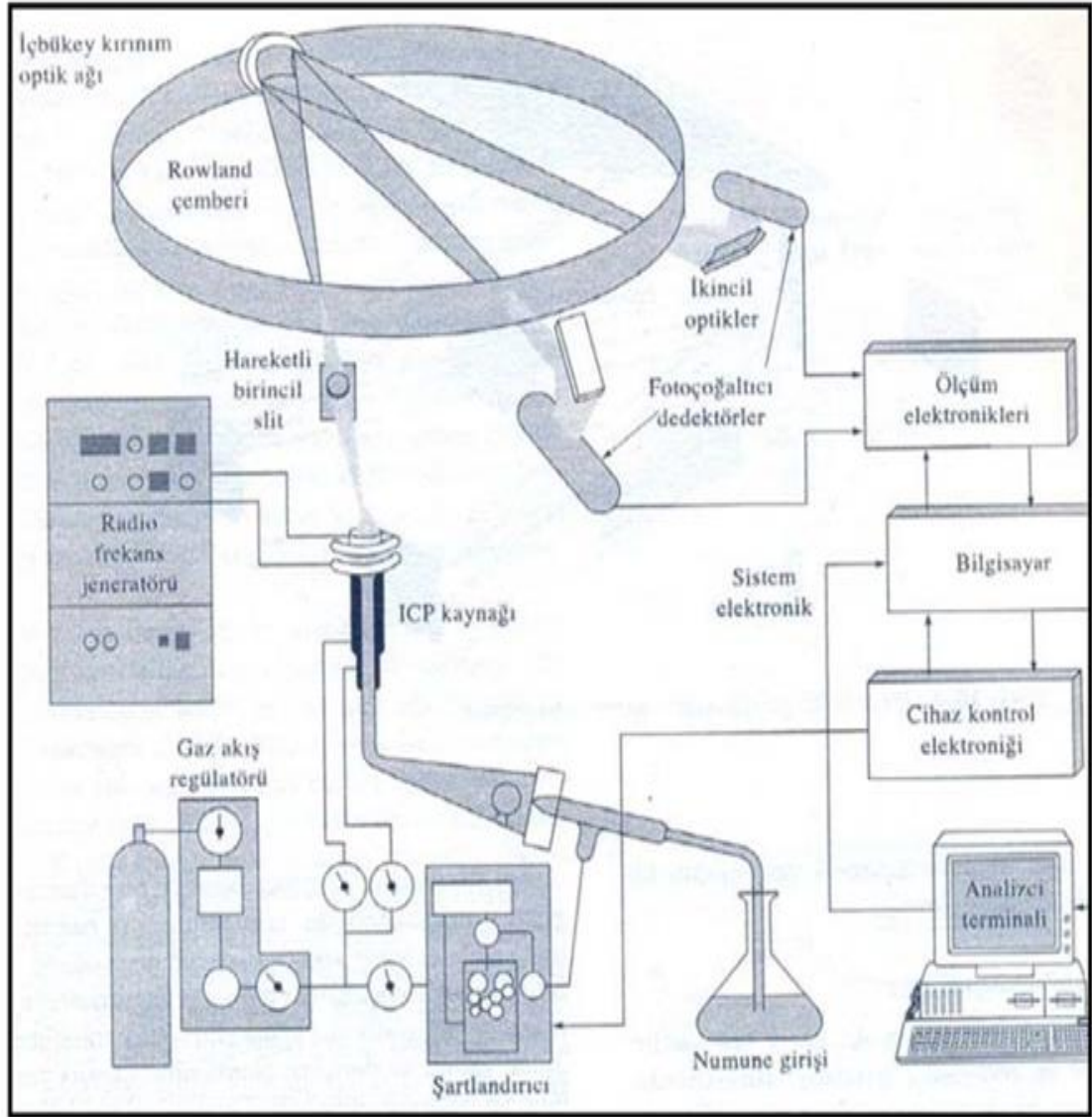
Şekil 5.1. ICP-OES Cihazının Yapısı
