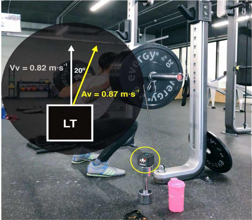
Şekil 2.1. 20^\circ sapmayla yapılan vertikal skuat kaldırışı sırasında, sapmayı hesaba (dikey hız / kosinüs açısı) katmadan yapılan ölçümle 0.82 \text{ m}\cdot\text{s}^{-1} hesaba katılarak elde edilen 0.87 \text{ m}\cdot\text{s}^{-1} ortalama hız verisi arasında fark vardır.
