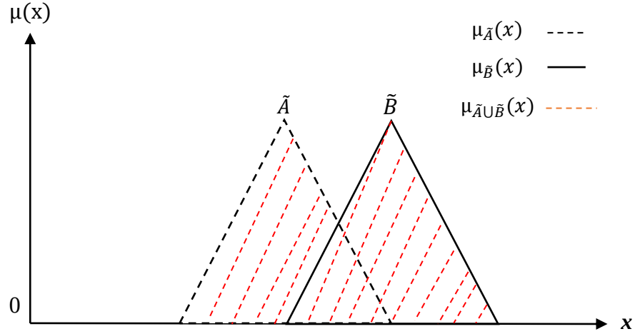
Şekil 1.7. Bulanık Kümelerde Birleşim İşlemi
