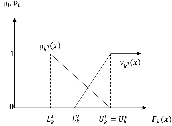
Şekil 2.4. Minimizasyon Yapılı Sezgisel Bulanık Kümelerde Üyelik Fonksiyonları
