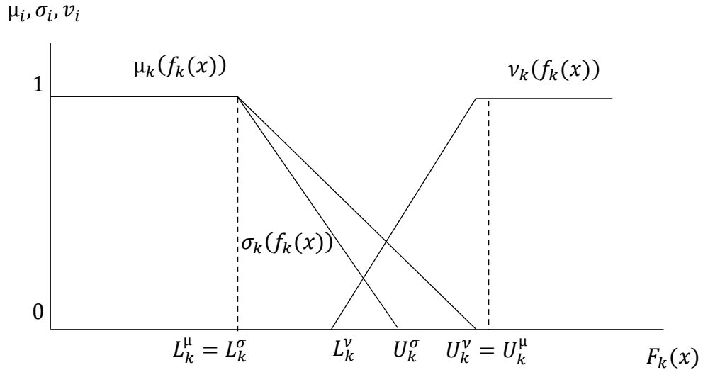
Şekil 2.6. Minimizasyon Yapılı Nötrosifik Bulanık Kümelerde Üyelik Fonksiyonları
