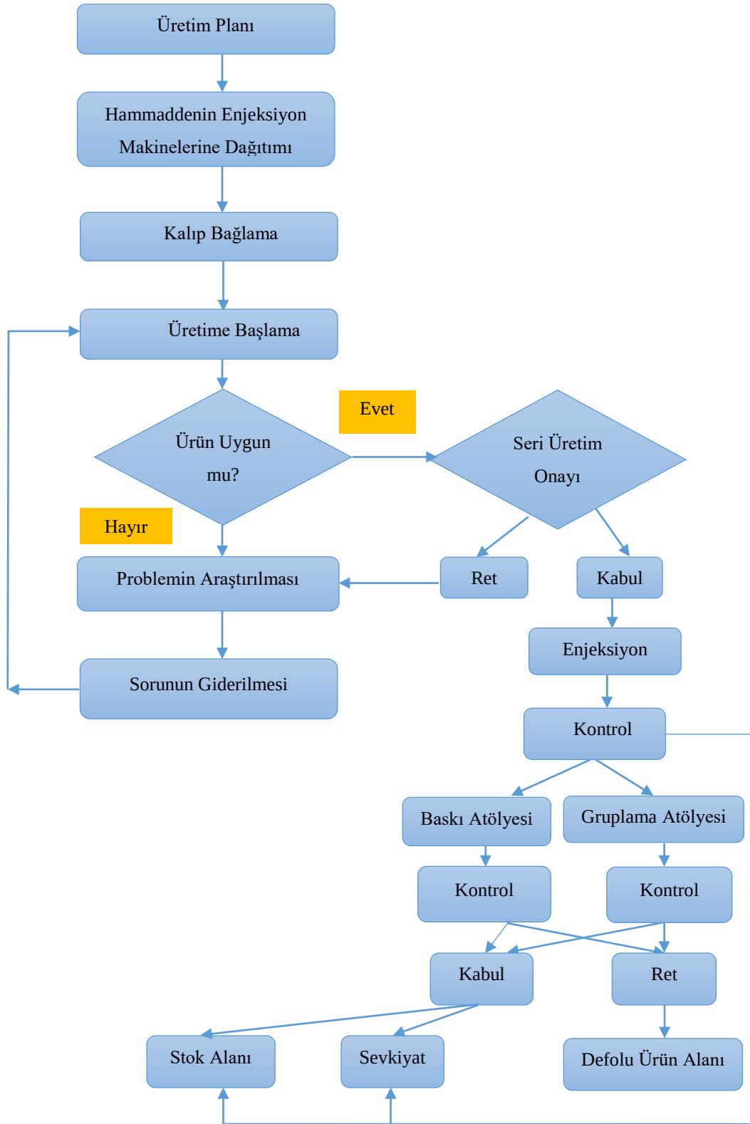
Şekil 3.1. Beyaz Eşya Plastik Ürünleri Üretim İşletmesinde İş Akış Diyagramı
