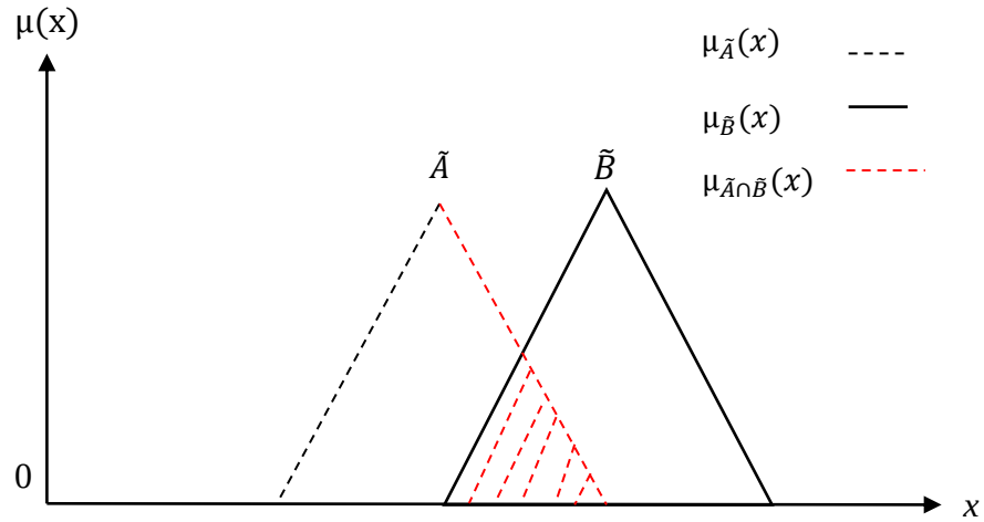
Şekil 1.8. Bulanık Kümelerde Kesişim İşlemi
