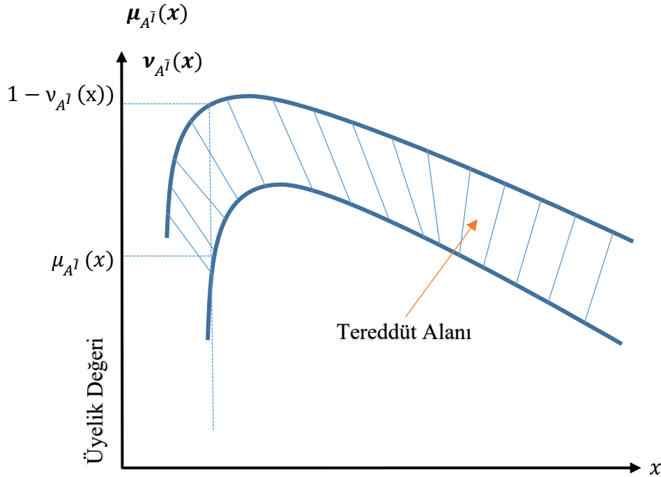
Şekil 1.11. Sezgisel Bulanık Küme Tereddüt Düzeyi (Garg, Rani & Sharma, 2013, s. 3)
