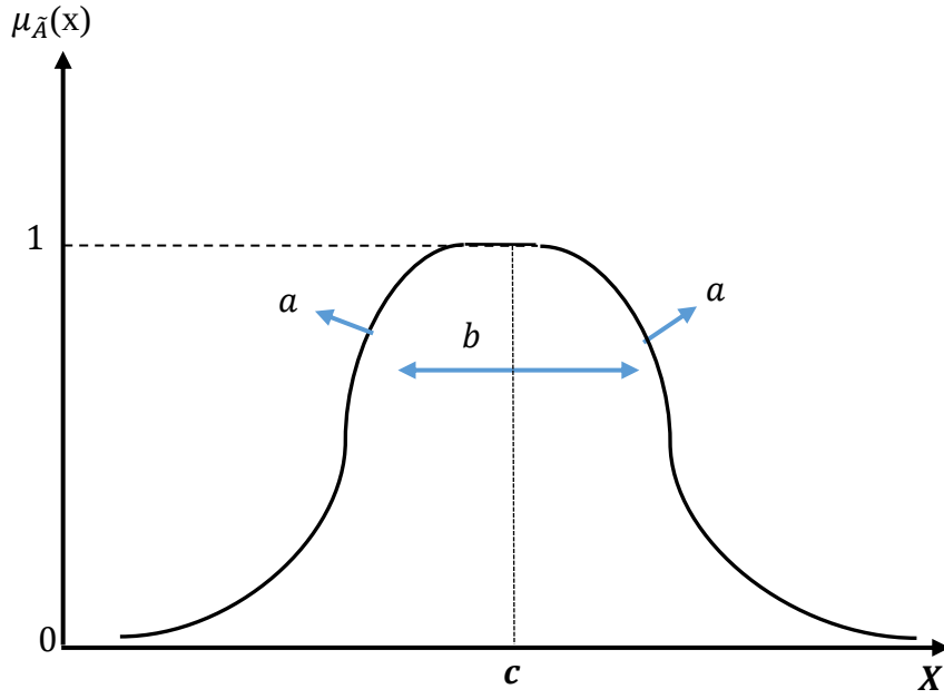
Şekil 1.6. Çan Eğrisi Üyelik Fonksiyonu (Aytaç, 2011, s. 81)
