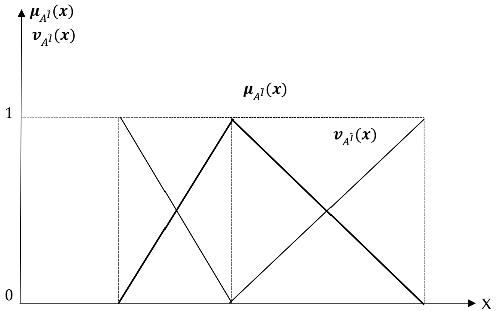
Şekil 1.10. Sezgisel Bulanık Kümelerde Üyelik Fonksiyonları (Naim & Hagrass, 2014, s. 1308)
