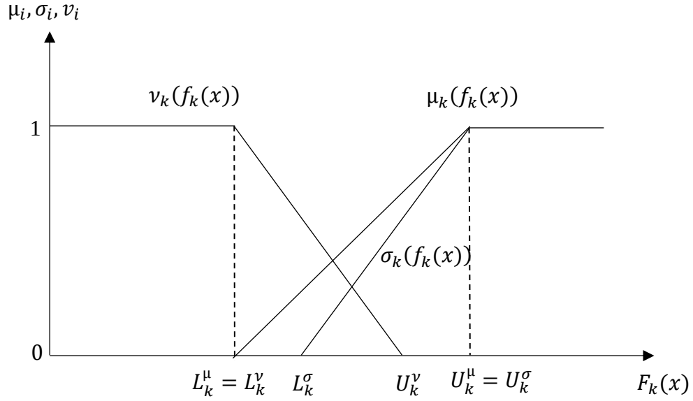
Şekil 2.5. Maksimizasyon Yapılı Nötrosofik Bulanık Kümelerde Üyelik Fonksiyonları
