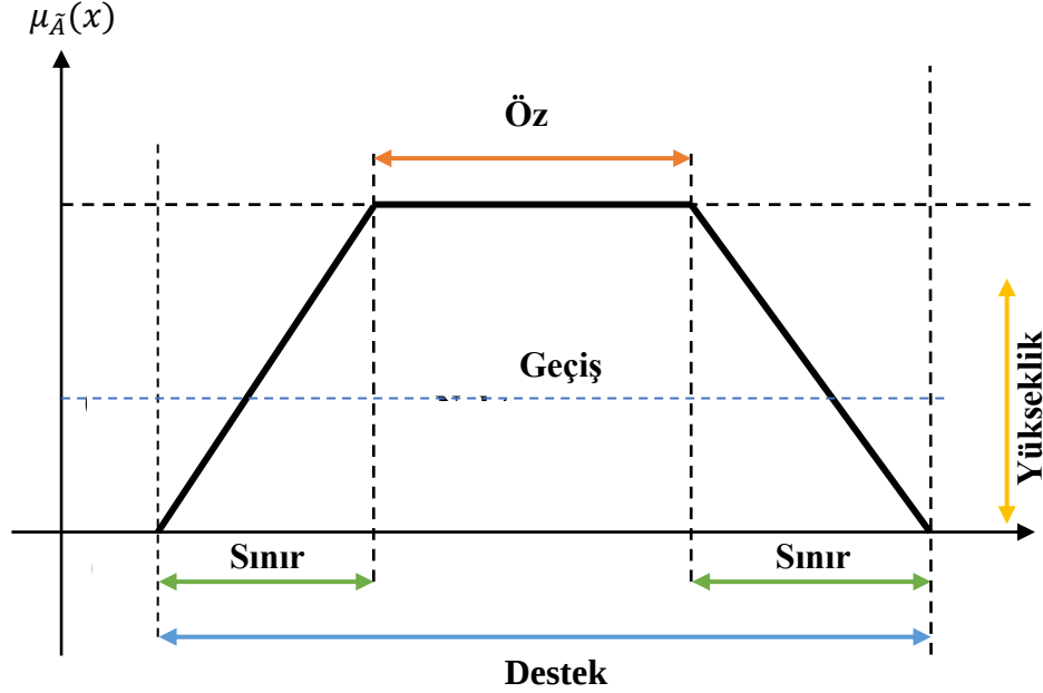
Şekil 1.1. Üyelik Fonksiyonunun Kısımları (Şen, 2009, s. 33)
