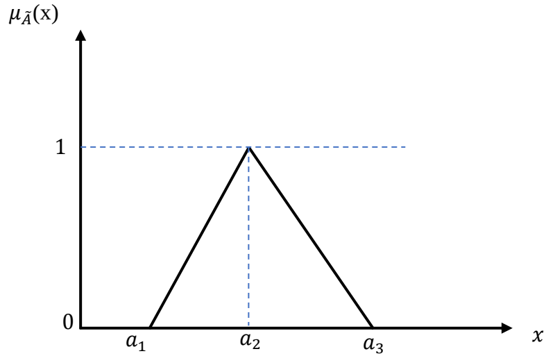
Şekil 1.3. Üçgen Üyelik Fonksiyonu (Zhang & Liu, 2006, s. 8)
