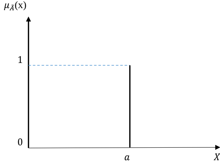
Şekil 1.2. Tekil Üyelik Fonksiyonu (Hanss, 2005, s. 50)
