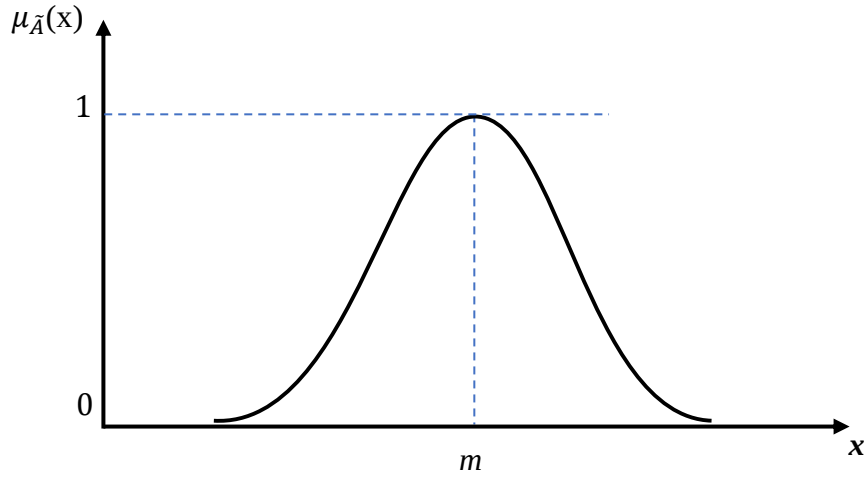
Şekil 1.5. Gaussian Üyelik Fonksiyonu (Massad, Ortega, & Carcalho de Barros, 2008, s. 24)
