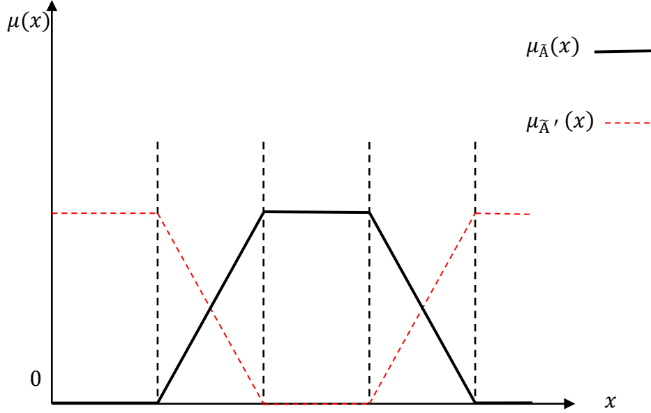
Şekil 1.9. Bulanık Kümelerde Tümleme İşlemi
