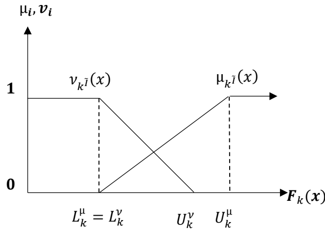
Şekil 2.3. Maksimizasyon Yapılı Sezgisel Bulanık Kümelerde Üyelik Fonksiyonları
