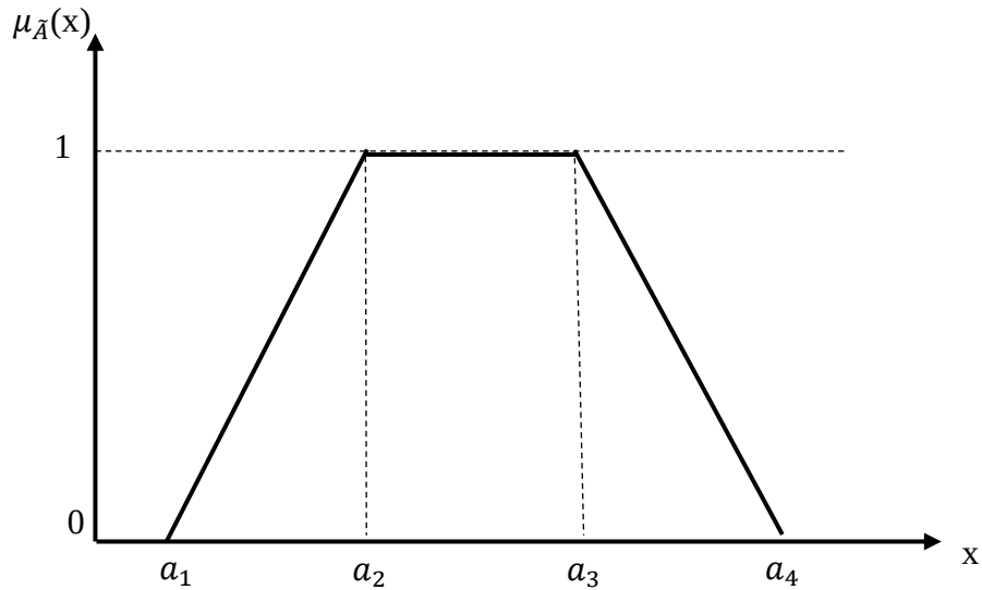
Şekil 1.4. Yamuk Üyelik Fonksiyonu (Akan, 2017, s. 110)
