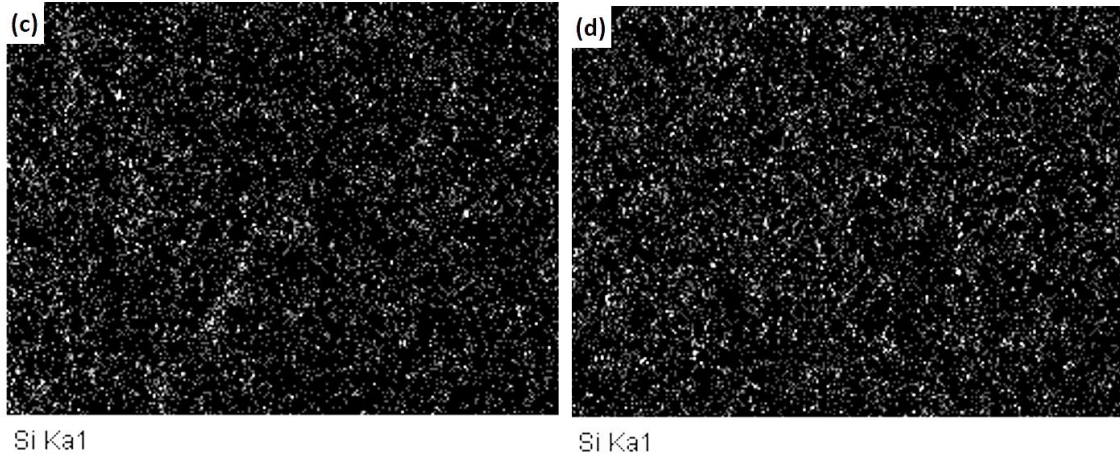
Şekil 1.106. (Devam). Düşük boyutlu Al_2O_3-ZrO_2 granülleri ile (a) hacimce %5, (b) hacimce %10 ve siklonlarla (c) hacimce %5, (d) hacimce %10 UBE Si_3N_4-ZrO_2 olacak şekilde dondurarak kurutma yöntemiyle yapılan denemelere ait numunelerin EDX haritalama tekniği ile elde edilen Si elementel haritaları
