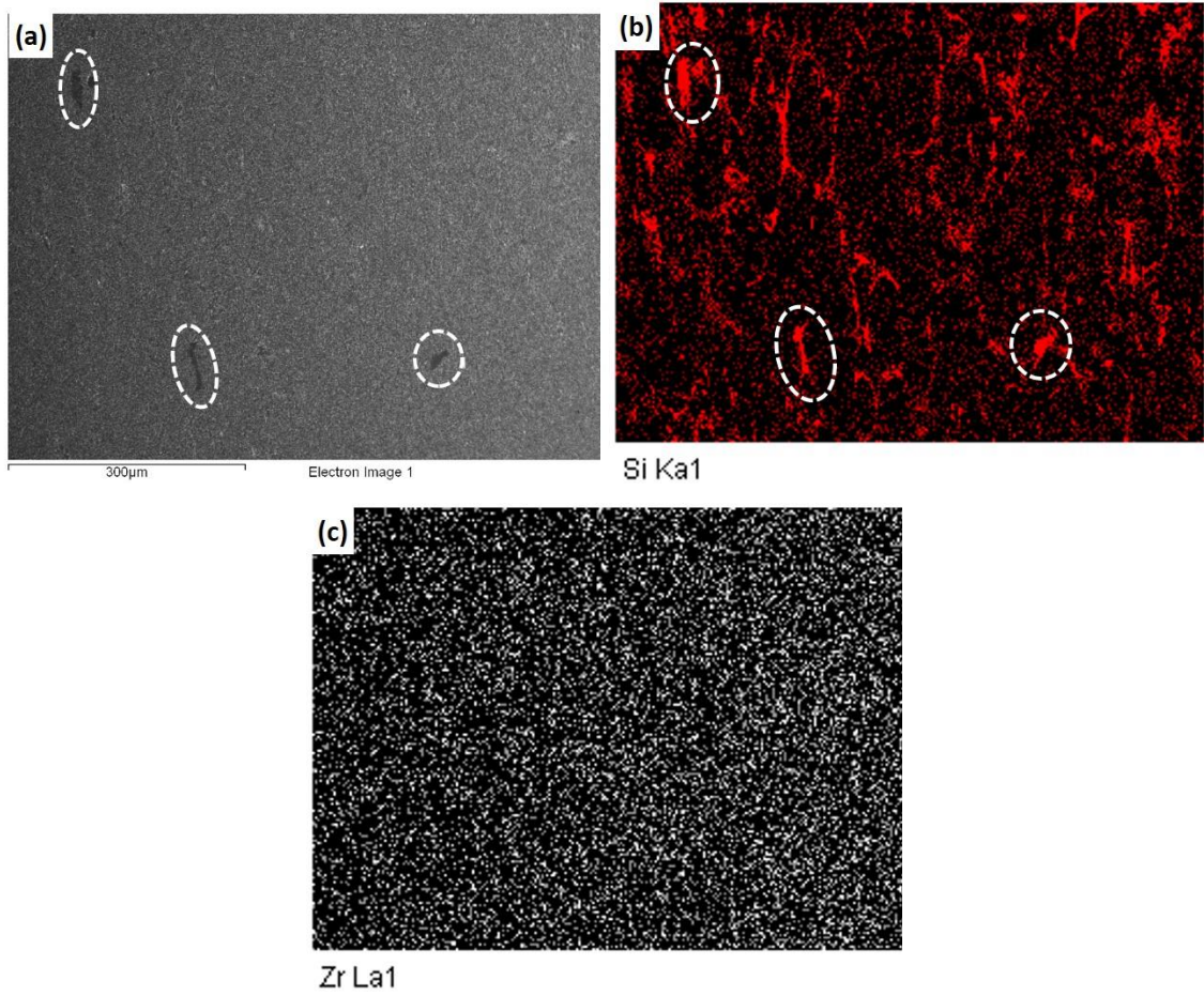
Şekil 1.94. 1000 dev/dk dönme hızında 10 dk süreyle karıştırılan AlZr-%10 uZeZr numunesine ait (a) BSE-SEM görüntüsü ile aynı yerden yapılan EDX haritalama analizi ile elde edilen (b) Si elementel haritası, (c) Zr elementel haritası. Si bölgeleri dairelerle gösterilmiştir.
