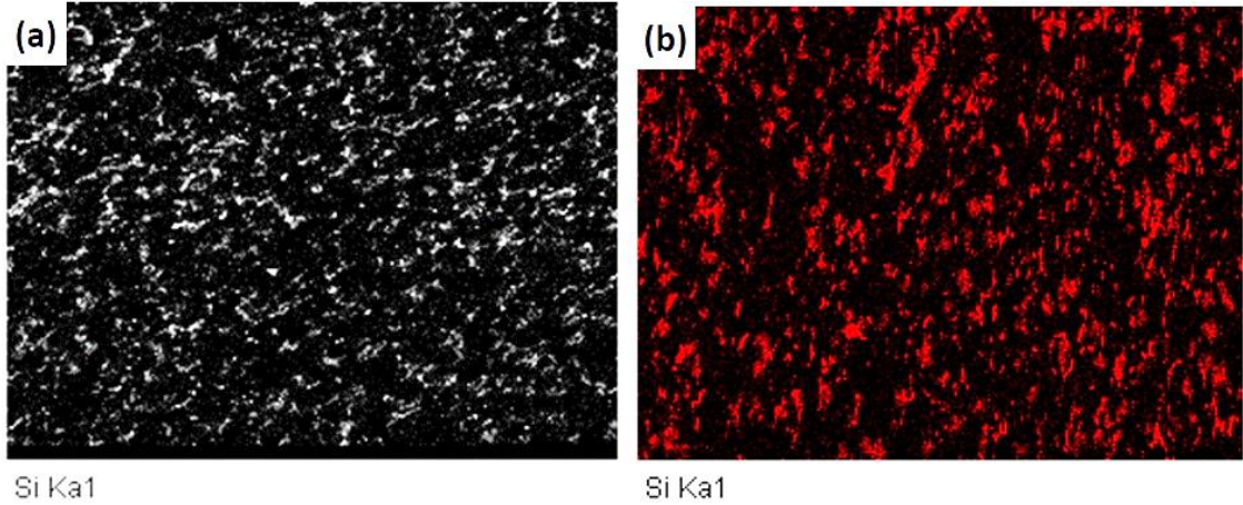
Şekil 1.104. (a) Yeni üretilen düşük boyutlu granüller, (b) eski granüller kullanılarak dondurarak kurutma yöntemiyle üretilen AlZr-%10 ubeZr numunelerine ait Si elementel haritaları
