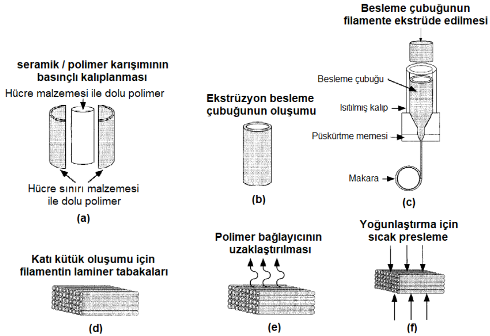
Şekil 1.18. Fibröz monolitlerin üretimi için ortak ekstrüzyon sürecinin şematik gösterimi: (a) başlangıç besleme çubuğunun şekillendirilmesi, (b) ekstrüzyon besleme çubuğunun oluşumu, (c) ortak ekstrüzyon, (d) katı kütük oluşumu laminasyon işlemi, (e) bağlayıcı uzaklaştırma ve (f) sıcak presleme [25]
