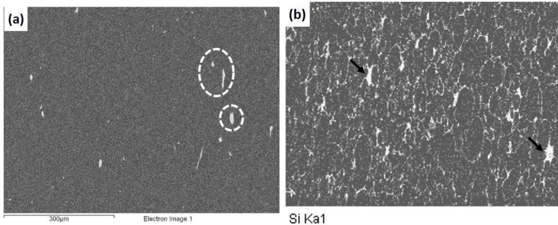
Şekil 1.84. Toz ağırlığının 1,5 katı kadar bilye ile karıştırılmış Si_3N_4-ZrO_2 tozunun Al_2O_3-ZrO_2 granülleri etrafına kaplanmasıyla elde edilen numunenin (a) BSE-SEM görüntüsü ve aynı yerden yapılan EDX haritalama analizi ile elde edilen (b) Si, (c) Zr, (d) Al elementel haritaları. Si bölgeleri oklarla, Zr bölgeleri dairelerle gösterilmiştir.
