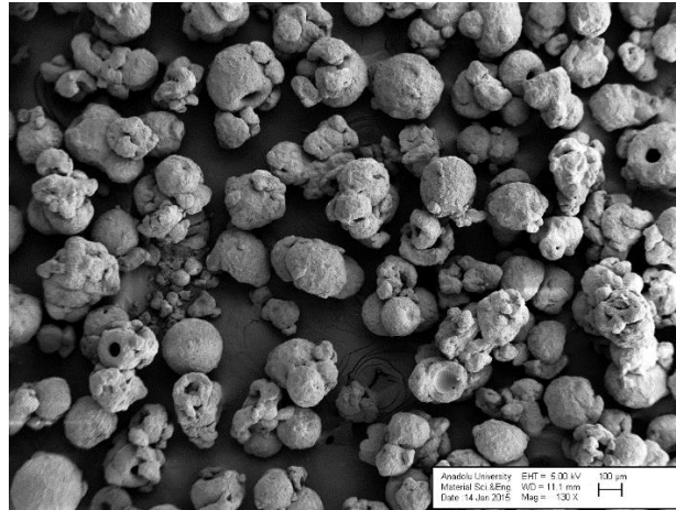
Şekil 1.92. 1000 dev/dk dönme hızında 10 dk süreyle karıştırılan AlZr-%10 ubeZr granüllerinin SE-SEM görüntüsü
