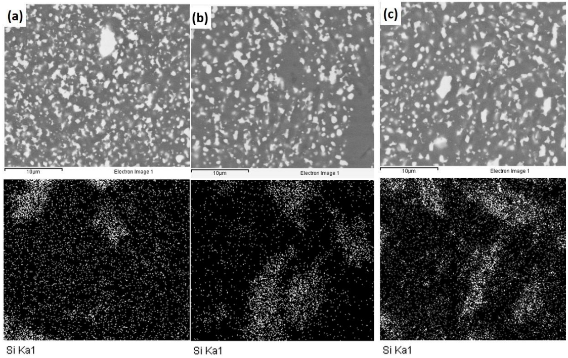
Şekil 2.4. Hacimce (a) %1, (b) %3, (c) %5 nano \text{Si}_3\text{N}_4 içeren numunelere ait BSE-SEM görüntüleri ile aynı yerden yerden yapılan EDX haritalama analizi ile edilen Si elementel haritaları
