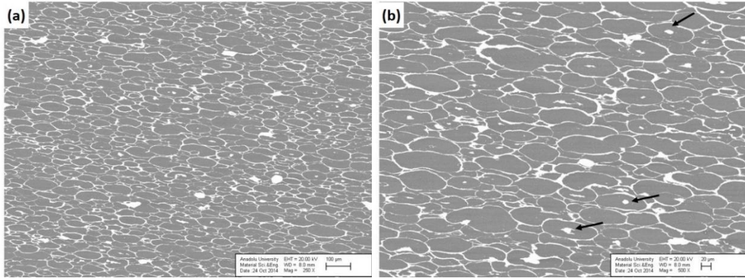
Şekil 1.63. Yalnızca su kullanılarak üretilen SL500 - %15 Zr numunesinin kesitten alınmış BSE-SEM görüntüleri (a) 250x, (b) 500x. Heterojen ZrO_2 bölgeleri oklarla gösterilmiştir.
