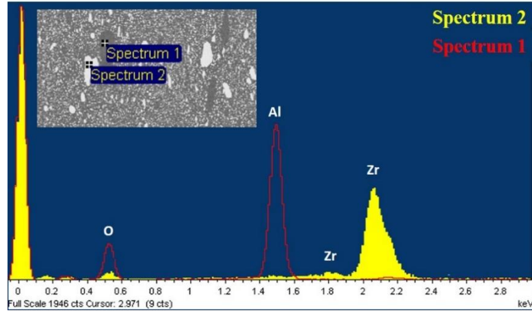
Şekil 2.3. Hacimce %3 nano \text{Si}_3\text{N}_4 içeren numuneye ait EDX analizi sonuçları
