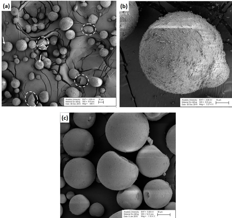
Şekil 1.75. \text{AlZr--}\%10 \text{ ubeZr} numunesine ait granüllerin (a) 426x, (b) 3270x büyütmedeki SE-SEM görüntüleri ile (c) kaplanmamış \text{Al}_2\text{O}_3\text{--ZrO}_2 granüllerinin SE-SEM görüntüsü. Parçalanmış granüller dairelerle, donat şeklindeki granüllere dolan tozlar oklarla gösterilmiştir.
