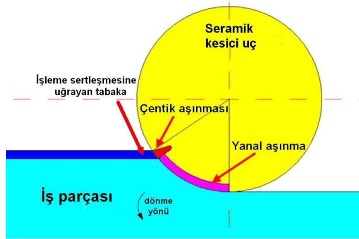
Şekil 1.2. Aşınma mekanizmasının şematik gösterimi. Yüzey sertleşmesine uğrayan tabaka koyu renk ile gösterilmiştir [12].
