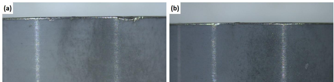
Şekil 2.9. Test edilen (a) hacimce %1, (b) hacimce %3, (c) hacimce %5 nano \text{Si}_3\text{N}_4 içeren nano kompozitlerin ve (d) \text{AlZr} matris, (e) \text{Al}_2\text{O}_3\text{--SiC}_v kesici uçların aşınma profilleri
