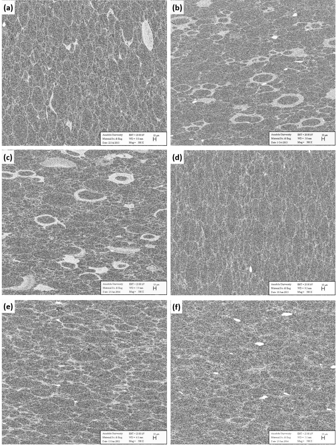
Şekil 1.52. Bilyalı değirmende yapılan (a) yağ ilavesiz, (b) 1 sa yağ ile karıştırılan, (c) 2 sa yağ ile karıştırılan SN80-%15 ubeZr numunelerinin ve (d) yağ ilavesiz, (e) 1 sa yağ ile karıştırılan, (f) 2 sa yağ ile karıştırılan SN80-%15 nanoZr numunelerinin BSE-SEM görüntüleri
