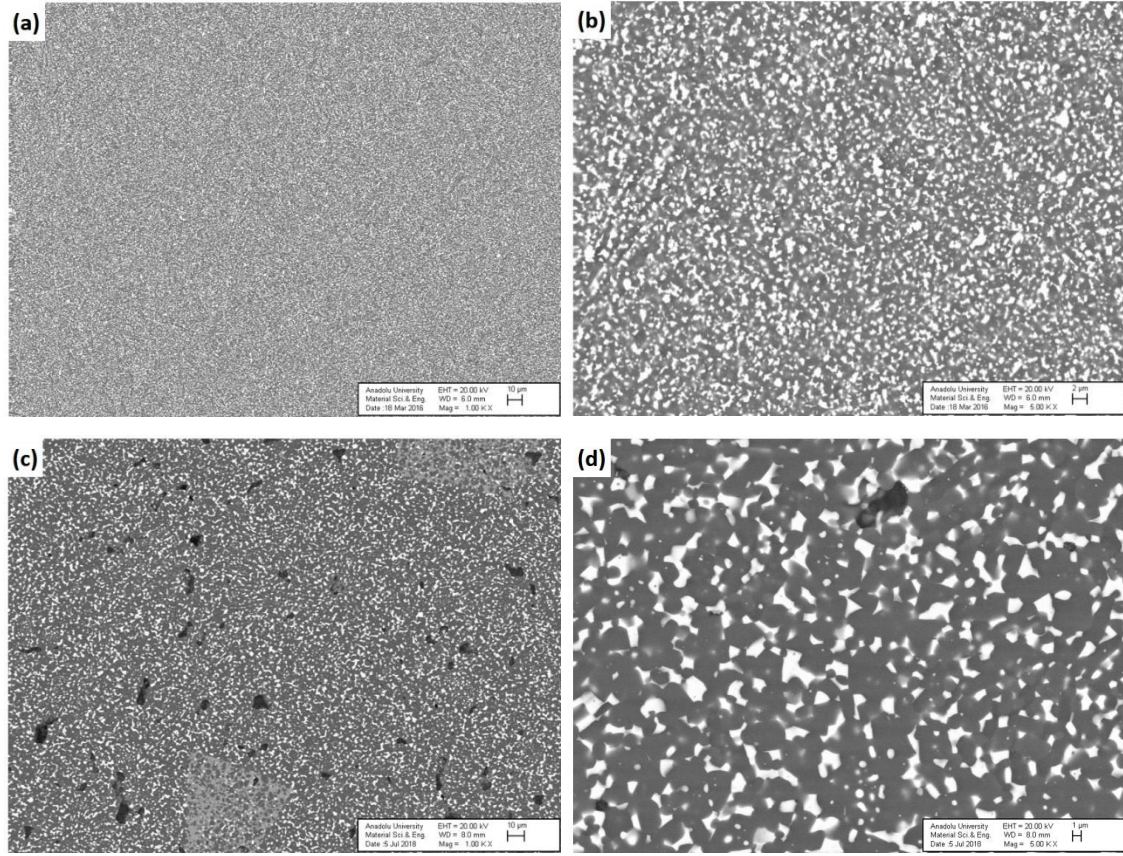
Şekil 3.11. Düşük boyutlu \text{Al}_2\text{O}_3\text{--ZrO}_2 granüllerine hacimce %5 \text{Si}_3\text{N}_4\text{--ZrO}_2 kaplanarak SPS ile üretilen numunenin (a) 1000x büyütmede, (b) 5000x büyütmede alınan BSE-SEM görüntüleri ile GPS ile üretilen numunelerin (c) 1000x büyütmede, (d) 500x büyütmede alınan BSE-SEM görüntüleri
