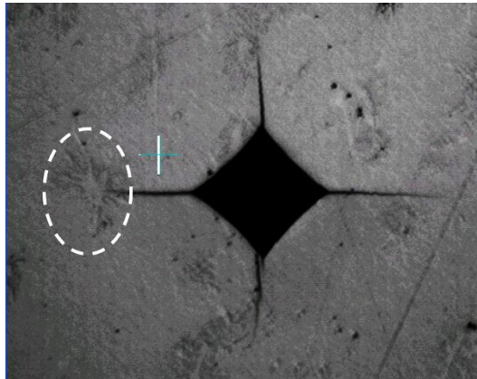
Şekil 1.89. \text{AlZr--}\%10 \text{ ubeZr} numunesine ait Vickers indent izi ve oluşan çatlaklar. Çatlağın heterojen bölgeyle etkileşimi daire ile gösterilmiştir.
