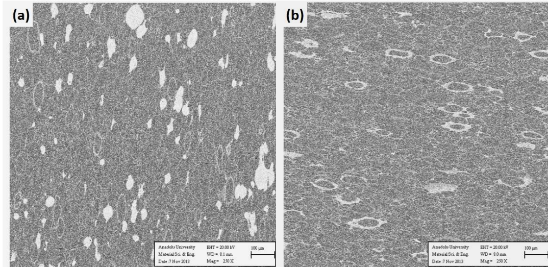
Şekil 1.54. UBE \text{Si}_3\text{N}_4 - \text{ZrO}_2 kaplama tozunun eksenel değirmende (a) kuru ortamda, (b) yaş ortamda karıştırılması ile elde edilen numunelerin BSE-SEM görüntüleri
