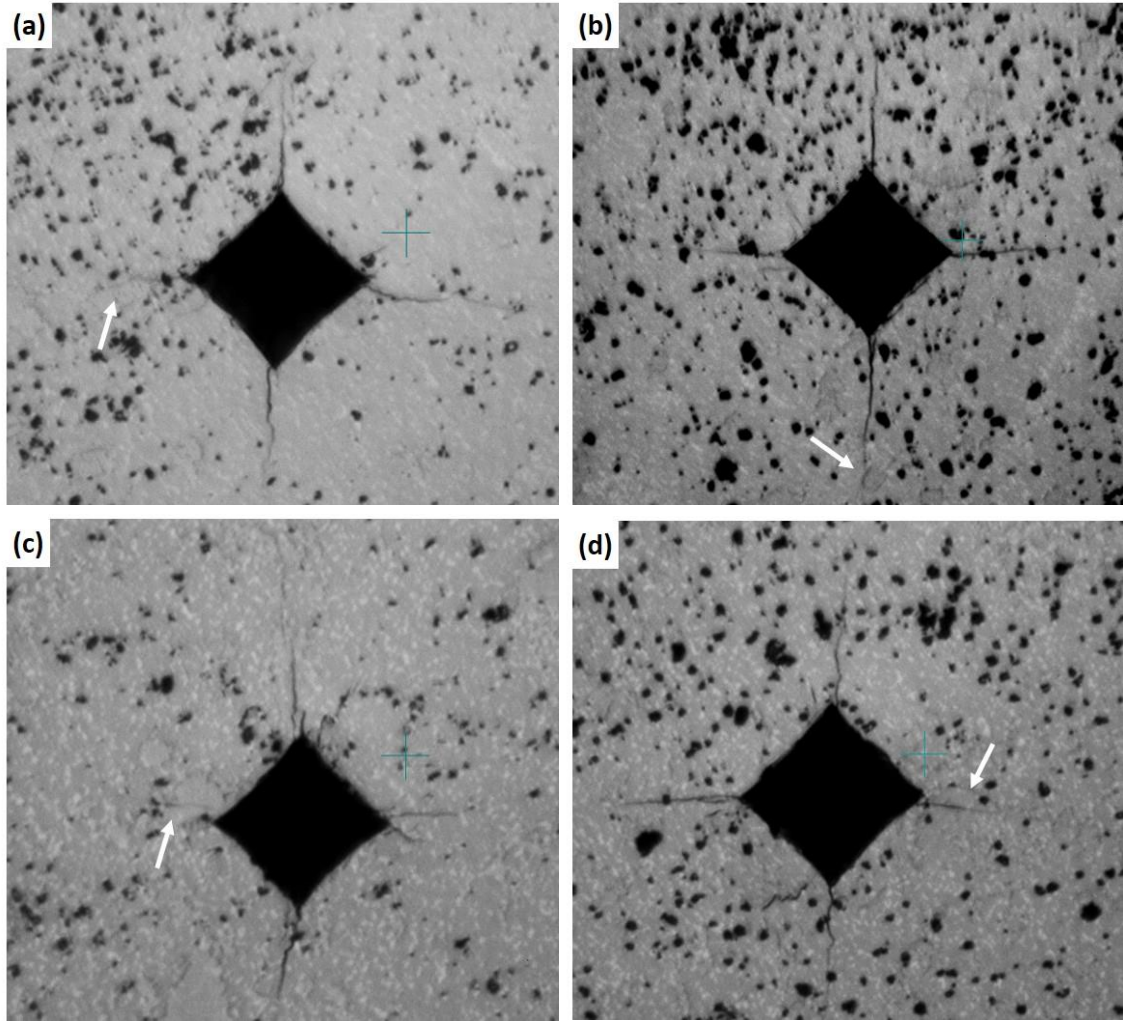
Şekil 3.6. Hacimce %1 nano \text{Si}_3\text{N}_4 içerip (a) GPS ile üretilen, (b) PLS ile üretilen, hacimce %3 nano \text{Si}_3\text{N}_4 içerip (c) GPS ile üretilen, (d) PLS ile üretilen numunelere ait Vickers indent izi ve oluşan çatlakların optik mikroskop görüntüsü. Çatlakların \text{Si}_3\text{N}_4 bölgeleriyle etkileşimi ok ile gösterilmiştir.
