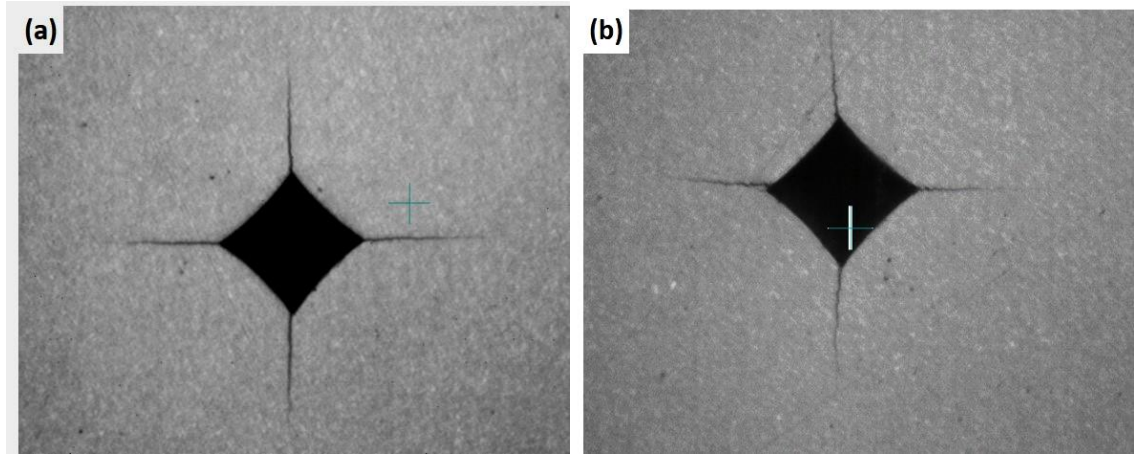
Şekil 2.7. (a) 500 dev/dk dönme hızıyla üretilen ve hacimce %3 nano Si 3 N 4 içeren numuneye, (b) AlZr matrise ait Vickers indent izi ve oluşan çatlaklar
