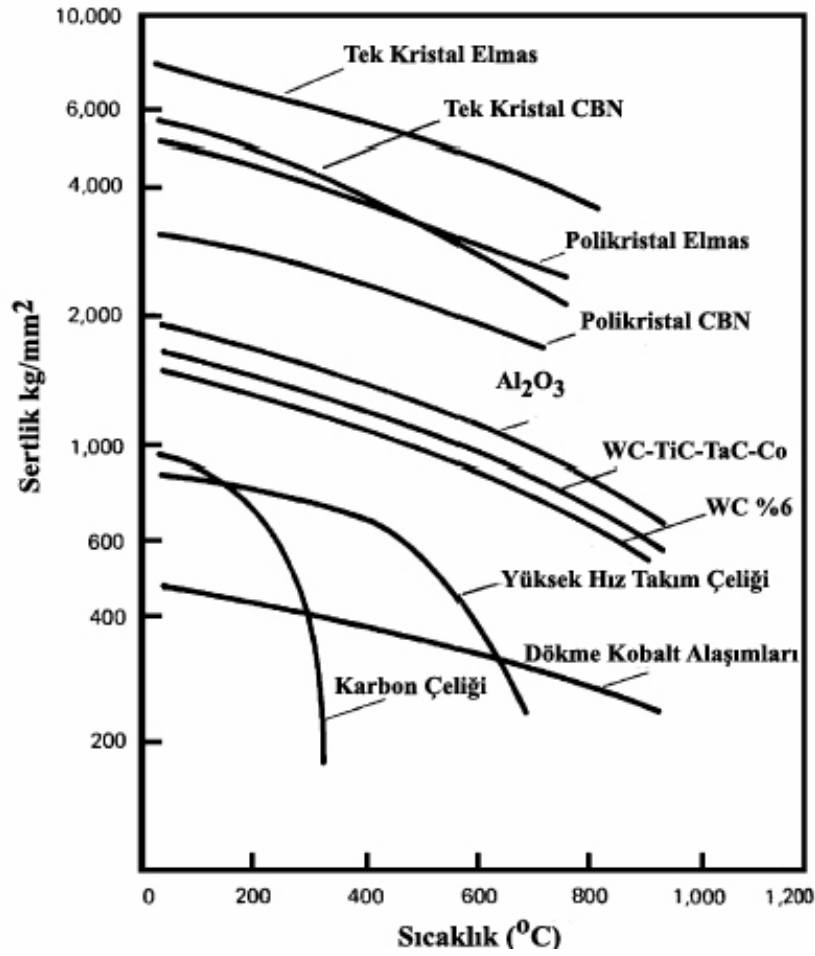
Şekil 1.9. Bazı kesici uç malzemelerinin sıcaklığa bağlı sertlik değişimleri [8]
