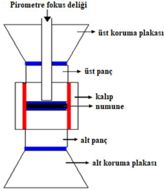
Şekil 1.39. SPS'te kullanılan kalıp sisteminin şematik gösterimi
