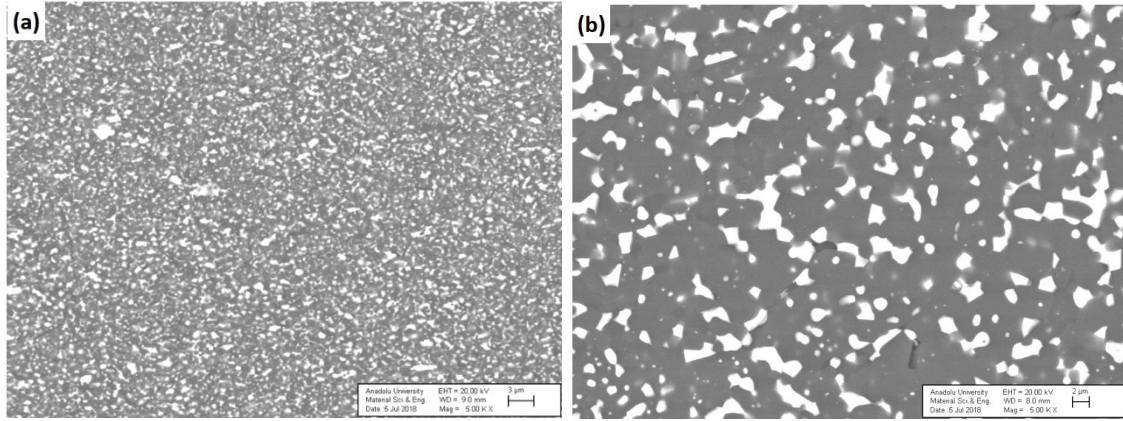
Şekil 3.14. Hacimce %3 nano \text{Si}_3\text{N}_4 içeren ve (a) SPS ile, (b) GPS ile üretilen numunelerin 5000x büyütmede alınmış BSE-SEM görüntüleri
