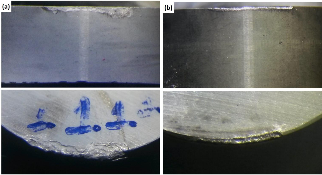
Şekil 1.87. (a) \text{AlZr--}\%10 nanoSN test numunesinin, (b) \text{Al}_2\text{O}_3\text{--SiC}_v kesici ucun alınma profilleri
