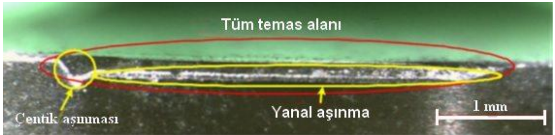
Şekil 1.1. Inconel 718'in yüksek hızda kaba işlenmesinde kullanılan SiAlON kesici uca görülen yanıl aşınma ve çentik aşınması [12]
