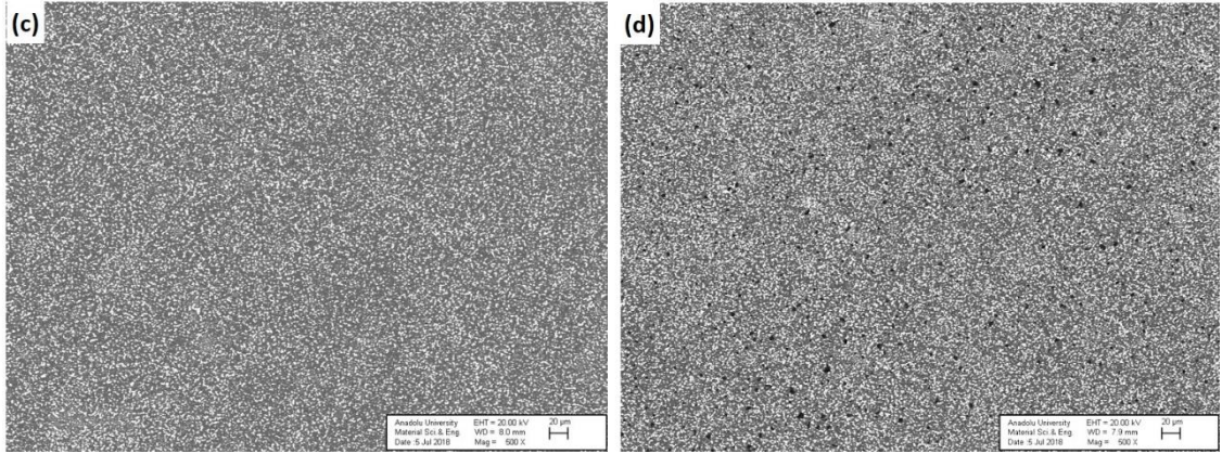
Şekil 3.12. (Devam) Hacimce %1 nano \text{Si}_3\text{N}_4 içerip (a) GPS ile üretilen, (b) PLS ile üretilen, hacimce %3 nano \text{Si}_3\text{N}_4 içerip (c) GPS ile üretilen, (d) PLS ile üretilen numunelere ait BSE-SEM görüntüleri
