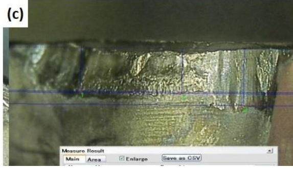
Şekil 1.60. (Devam) GGG 40 malzemesinin işlenmesi sonucu oluşan aşınma profilleri (a) AlZr-%15 nanoZr, (b) SN80E, (c) SL550C
