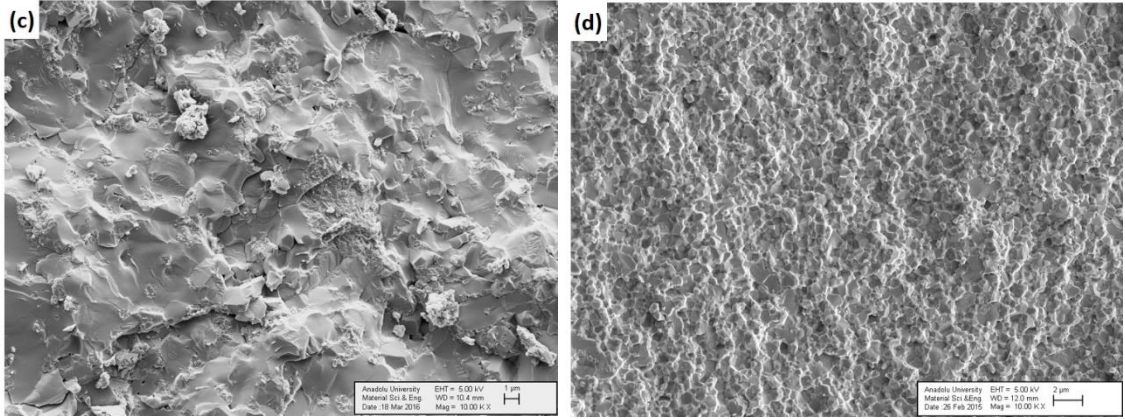
Şekil 2.5. (Devam) Hacimce (a) %1, (b) %3, (c) %5 nano \text{Si}_3\text{N}_4 içeren numunelerle (d) \text{AlZr} matrise ait SE-SEM görüntüleri
