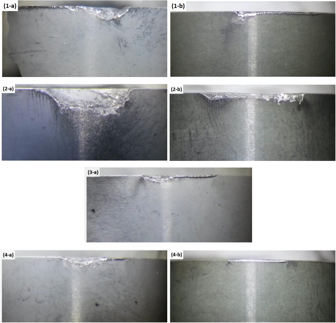
Şekil 1.109. Farklı kesme koşullarında test edilen kesici uçların aşınma profilleri. Baştaki rakam Tablo 1.23’de verilen kesme koşulunu ifade ederken (a) AlZr-%10 ubeZr numunesini, (b) Al 2 O 3 -SiC v kesici ucu ifade etmektedir.
