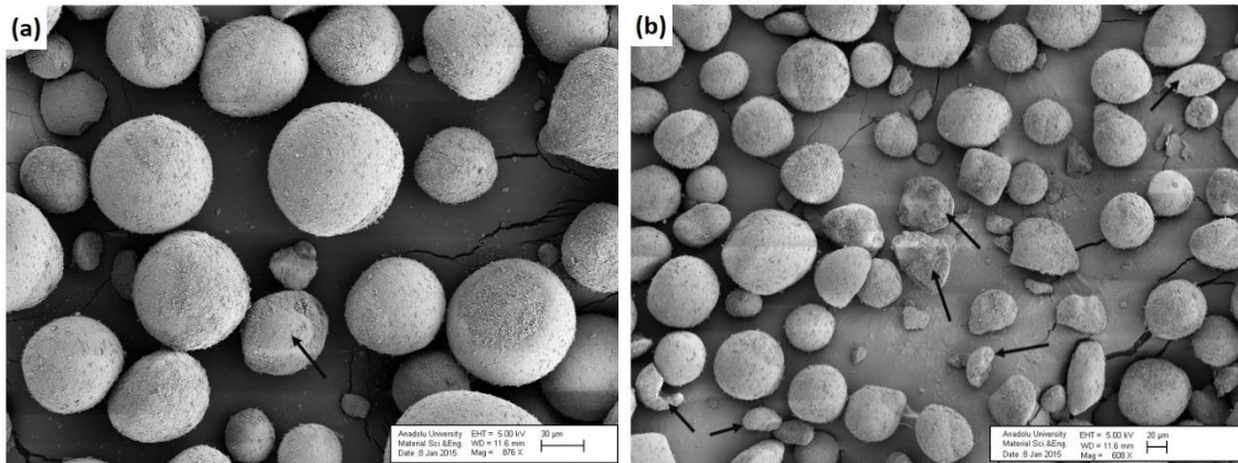
Şekil 1.78. Şiddetli karıştırıcıda 30 dk süreyle (a) 700 dev/dk, (b) 1000 dev/dk dönme hızlarında yapılan AlZr-%12 NbZr numunesine ait granüllerin SE-SEM görüntüleri. Granüllerden kopan parçalar oklarla gösterilmiştir.
