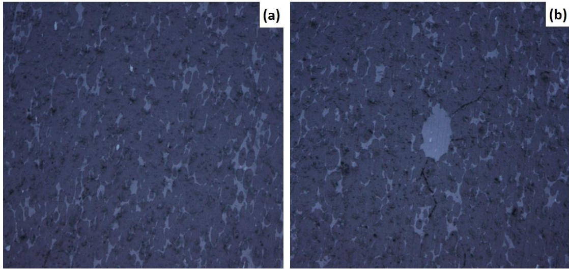
Şekil 1.79. Şiddetli karıştırıcıda 30 dk süreyle (a) 700 dev/dk, (b) 1000 dev/dk dönme hızlarında yapılan AlZr -%12 ubeZr numunelerine ait BSE-SEM görüntüleri
