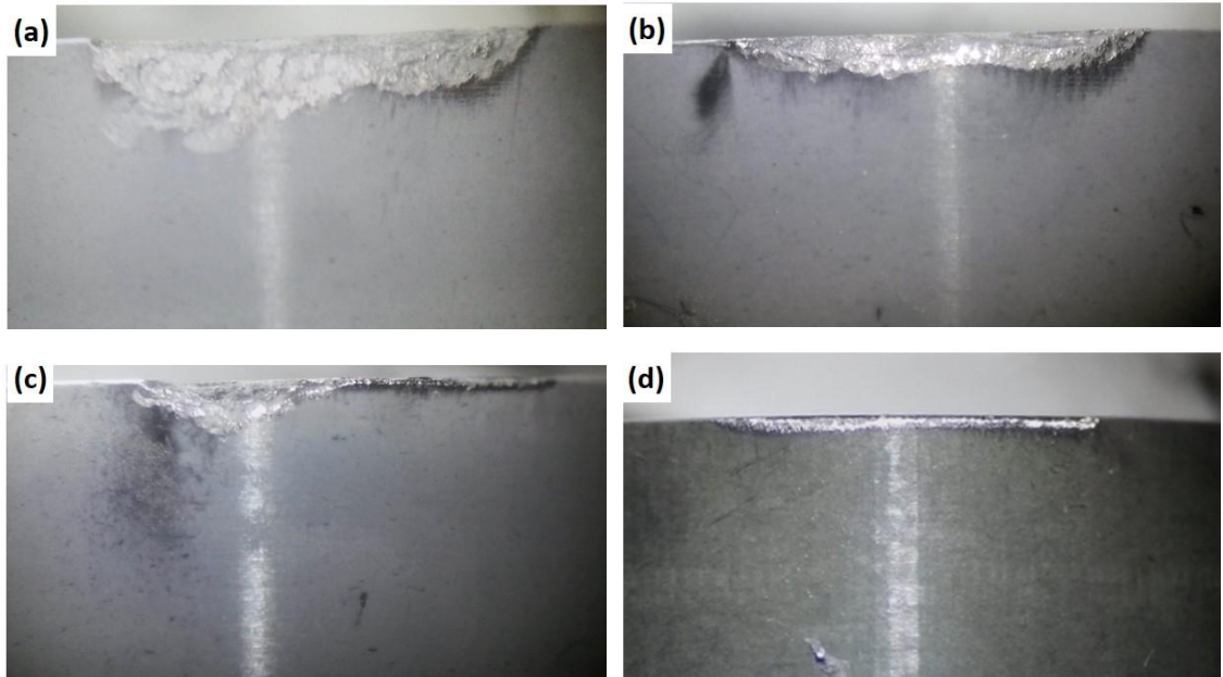
Şekil 1.88. 300 m/dk kesme hızıyla yapılan testlerde kullanılan (a) \text{AlZr} -%10 ubeZr, (b) \text{AlZr} -%10 nanoZr numunesinin, (c) 400 m/dk kesme hızıyla yapılan testte kullanılan \text{AlZr} -%10 nanoZr numunesinin, (d) referans olarak alınan \text{Al}_2\text{O}_3 - \text{SiC}_v kesici ucun aşınma profilleri
