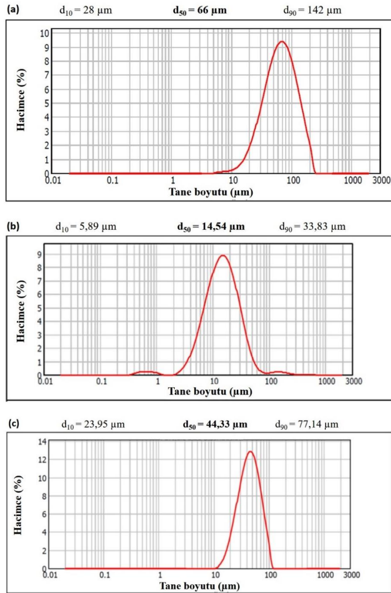
Şekil 1.103. (a) \text{Al}_2\text{O}_3\text{-ZrO}_2 granüllerinin (b) siklonların, (c) 75 \mu\text{m} 'lik elekten elenen granüllerin tane boyut dağılım grafikleri
