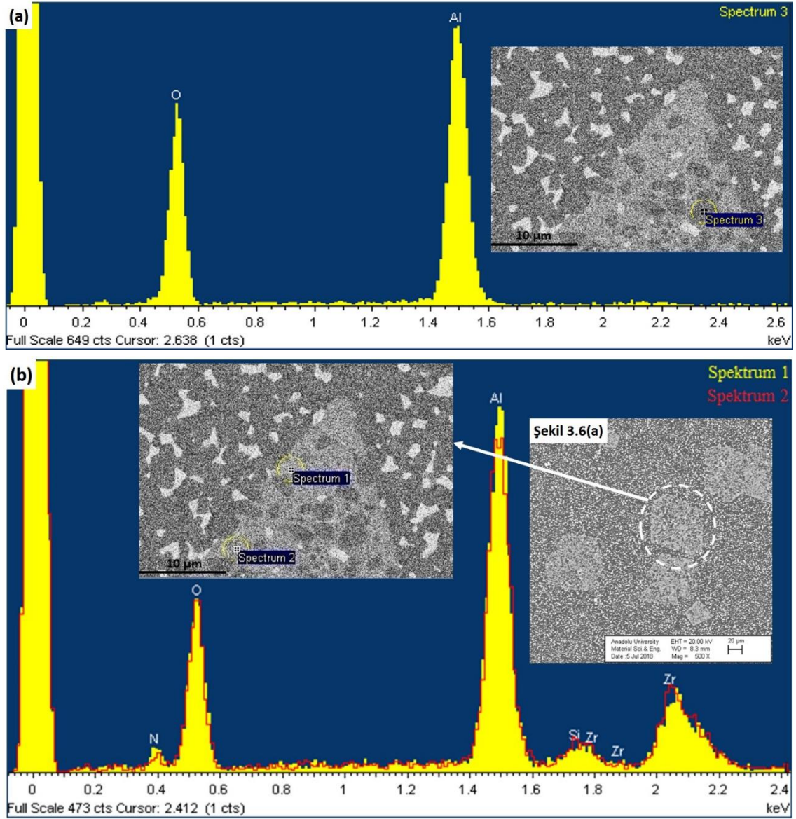
Şekil 3.9. Granüllere hacimce %5 UBE \text{Si}_3\text{N}_4\text{-ZrO}_2 kaplanarak yapılan ve GPS ile üretilen numuneye yüksek büyütmede (8730x) yapılan EDX nokta analizleri
