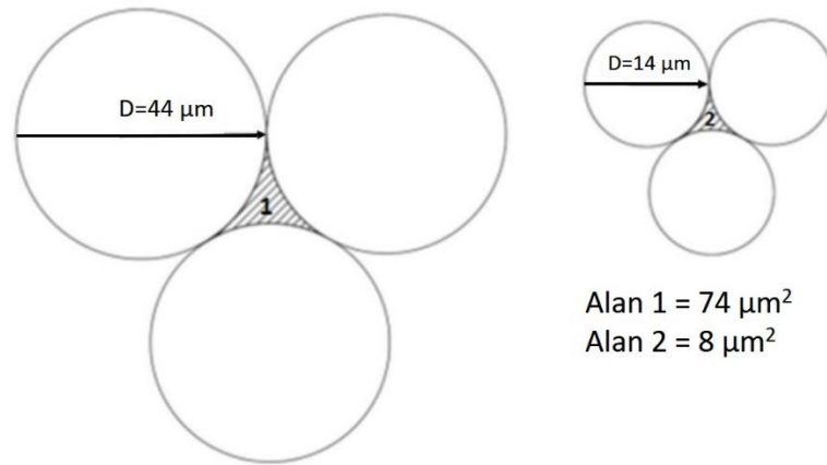
Şekil 1.102. Düşük boyutlu \text{Al}_2\text{O}_3\text{-ZrO}_2 granülleri ile siklonların arasında kalan üçlü bölgenin alanının şematik gösterimi
