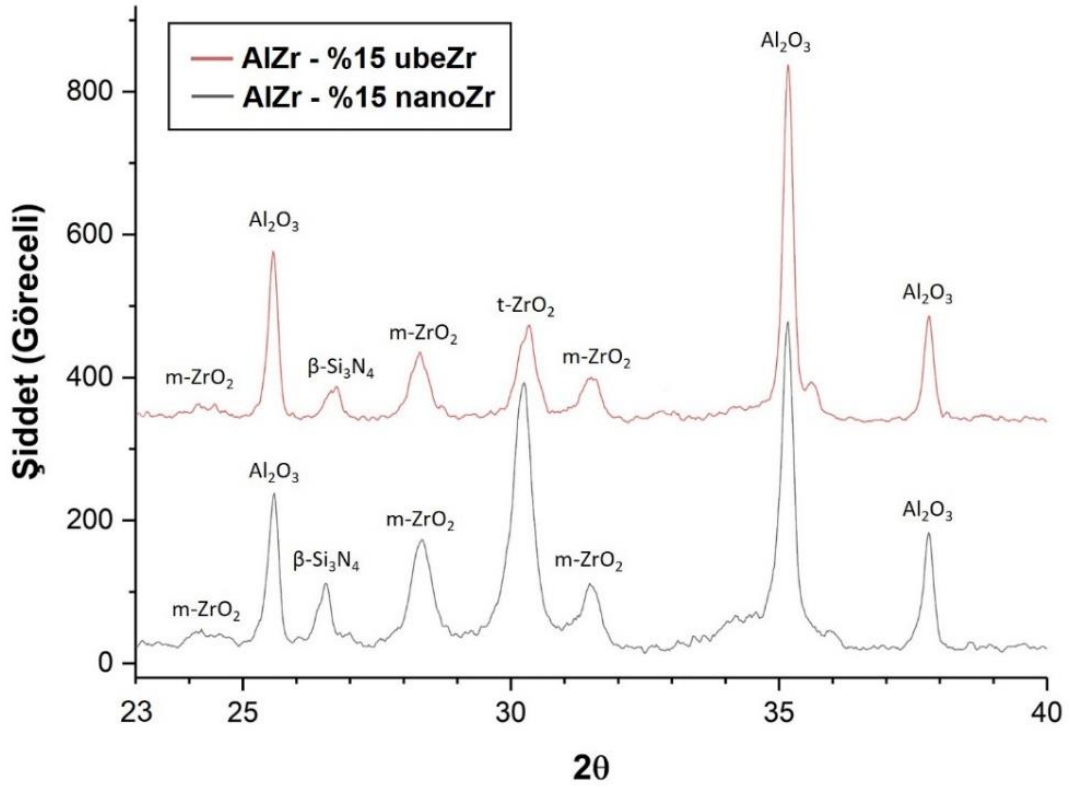
Şekil 1.43. AlZr-%15 ubeZr ve AlZr-%15 nanoZr numunelerine ait XRD paternleri
