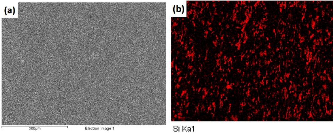
Şekil 1.100. Dondurarak kurutma yöntemiyle üretilen \text{AlZr-}\%10 \text{ uBeZr} numunesine ait (a) BSE-SEM görüntüsü ile aynı yerden yapılan EDX haritalama analizi ile elde edilen (b) Si elementel haritası
