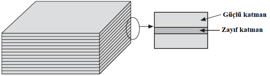
Şekil 1.16. Güçlü ve zayıf katmanlara sahip laminar kompozitin şematik gösterimi [54].
