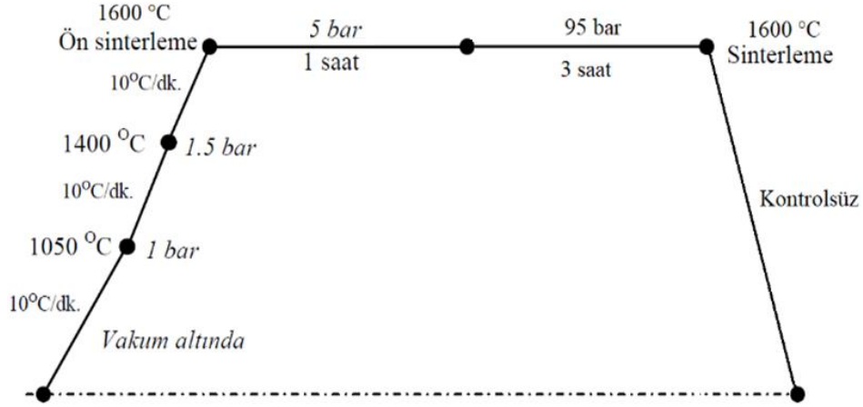
Şekil 3.2. GPS sinterleme rejiminin şematik gösterimi
