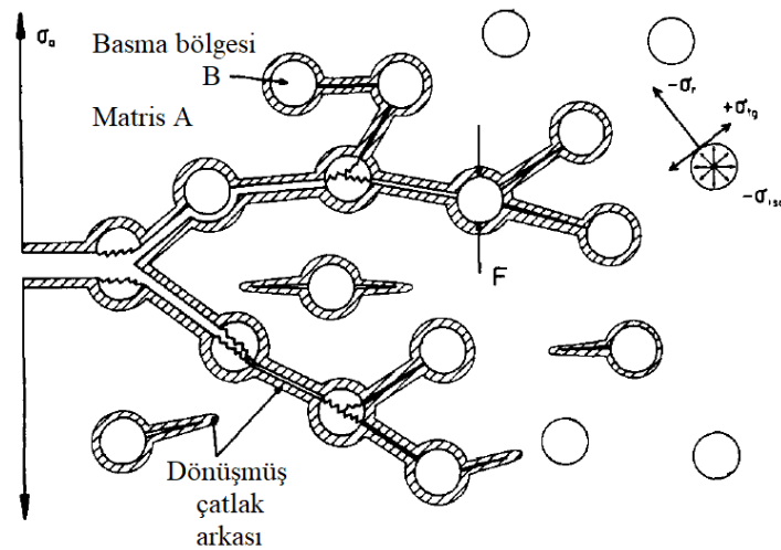
Şekil 1.11. TZP (Tetragonal Zirkonya Polikristal) matrisli dubleks seramikte çatlak ilerlemesinin şematik gösterimi [52]
