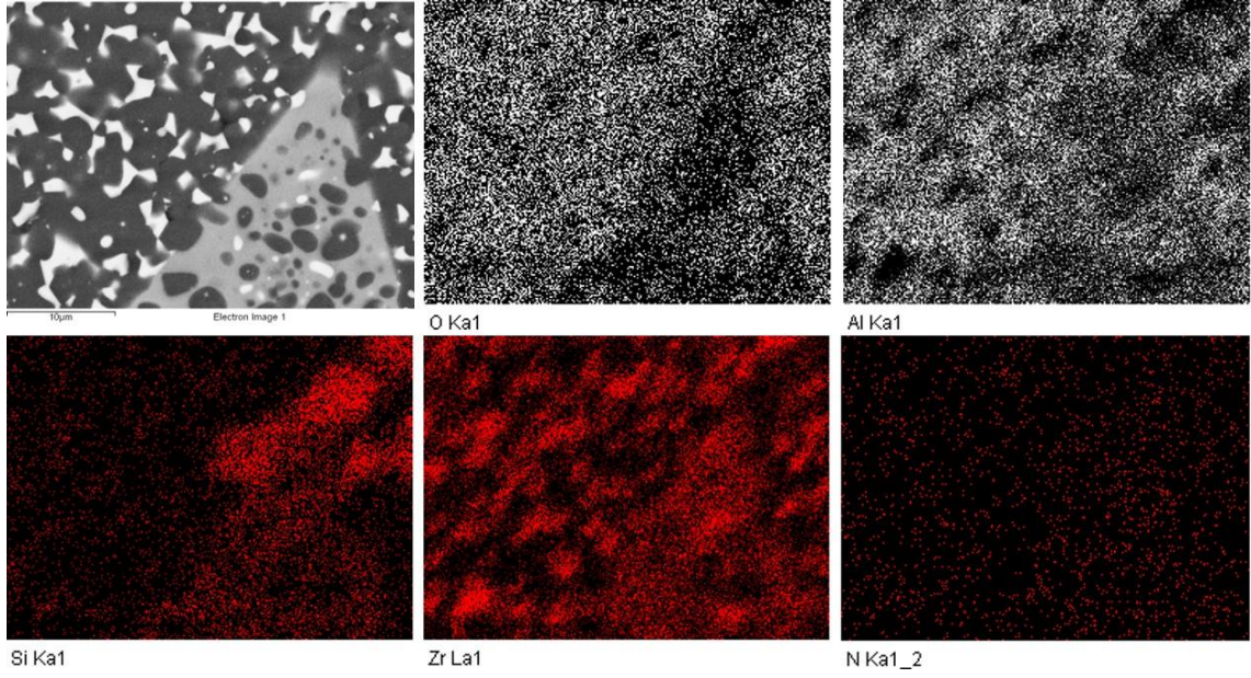
Şekil 3.10. Granüllere hacimce %5 UBE \text{Si}_3\text{N}_4\text{-ZrO}_2 kaplanarak yapılan ve GPS ile üretilen numuneye yüksek büyütmede (8730x) yapılan EDX haritalama analizi
