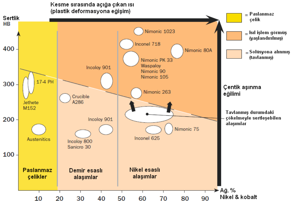
Şekil 1.5. Farklı alaşımların kompozisyona bağlı sertlikleri ve aşınma eğilimleri [37]
