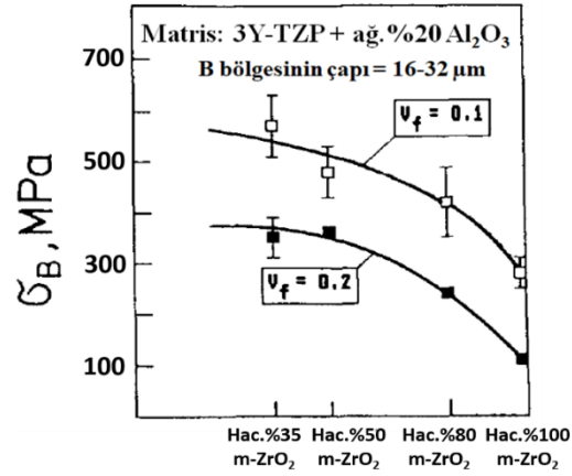
Şekil 1.13. Farklı basınç bölgesi miktarlarına sahip dubleks seramiklerin mukavemeti. Hacim fraksiyonu ve m-ZrO 2 miktarı arttıkça mukavemet azalır [53]
