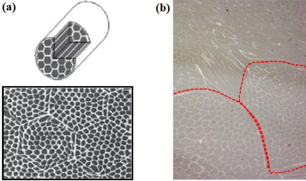
Şekil 1.27. CF1 kodlu fibröz monolit kesici uca ait (a) katalogda yer alan şematik gösterimi, (b) kesit optik mikroskop görüntüsü. Kırmızı çizgiyle gösterilen hücreler ikincil filamenti temsil etmektedir [23].
