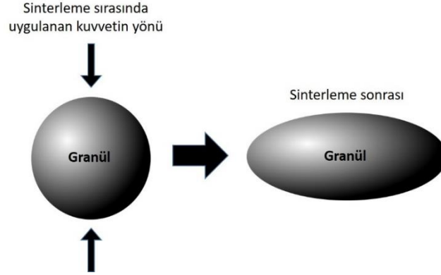
Şekil 1.67. Granüllerin, sinterleme sırasında uygulanan kuvvetin yönüne bağlı olarak yönlennesinin şematik gösterimi
