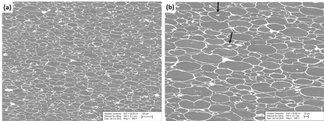
Şekil 1.64. Su-PEG karışımı kullanılarak üretilen SL500 - %15 Zr numunesinin kesitten alınmış BSE-SEM görüntüleri (a) 250x, (b) 500x. Heterojen ZrO_2 bölgeleri oklarla gösterilmiştir.
