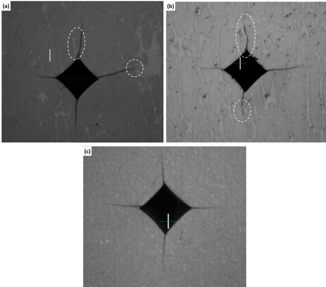
Şekil 1.61. (a) AlZr-%10 ubeZr, (b) AlZr-%10 nanoZr, (c) AlZr matris numunelerine ait Vickers indent izleri ve oluşan çatlaklar. Çatlakların heterojen bölgelerle etkileşimi dairelerle gösterilmiştir.
