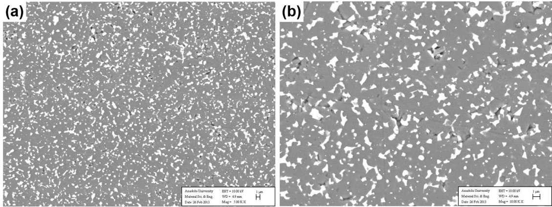
Şekil 1.31. CF1 kodlu fibröz monolit kesici ucun hücre içerisinde alınmış (a) 5kx büyütme, (b) 10kx büyütme BSE-SEM görüntüleri
