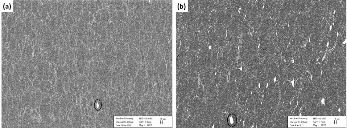
Şekil 1.49. SN80 granüllerinin (a) hacimce %10, (b) hacimce %20 \text{Si}_3\text{N}_4\text{-ZrO}_2 kaplanmasıyla üretilen numunelerin BSE-SEM görüntüleri. Heterojen \text{ZrO}_2 dairelerle gösterilmiştir.
