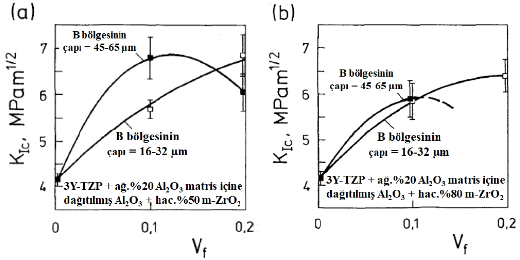
Şekil 1.14. 3Y-TZP + ağırlıkça %20 Al 2 O 3 matris içine dağıtılmış (a) Al 2 O 3 + hac.%50 m-ZrO 2 , (b) Al 2 O 3 + hac.%80 m-ZrO 2 dubleks seramiklerin kırılma tokluğu [53]
