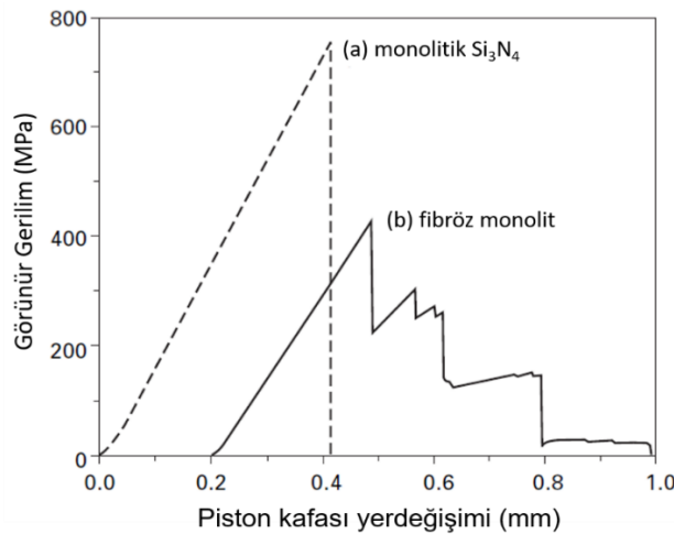
Şekil 1.21. (a) monolitik \text{Si}_3\text{N}_4 , (b) fibröz monolit seramiğin eğilme tepkisi [68]
