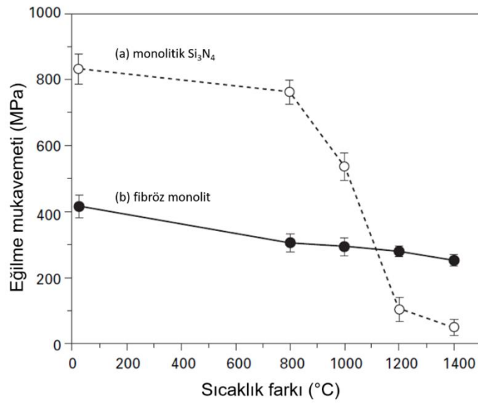
Şekil 1.22. (a) Monolitik \text{Si}_3\text{N}_4 , (b) fibröz monolit seramiğin ısı şok testi sonrası eğilme tepkisi. monolitik \text{Si}_3\text{N}_4 gevrek kırılma gösterirken fibröz monolitte gevrek olmayan hasar görülmektedir [68].
