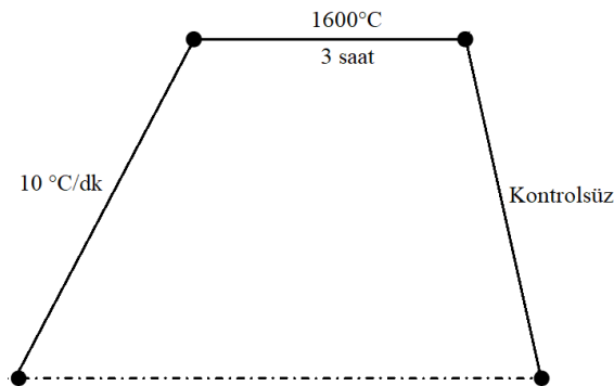
Şekil 3.3. PLS sinterleme rejiminin şematik gösterimi
