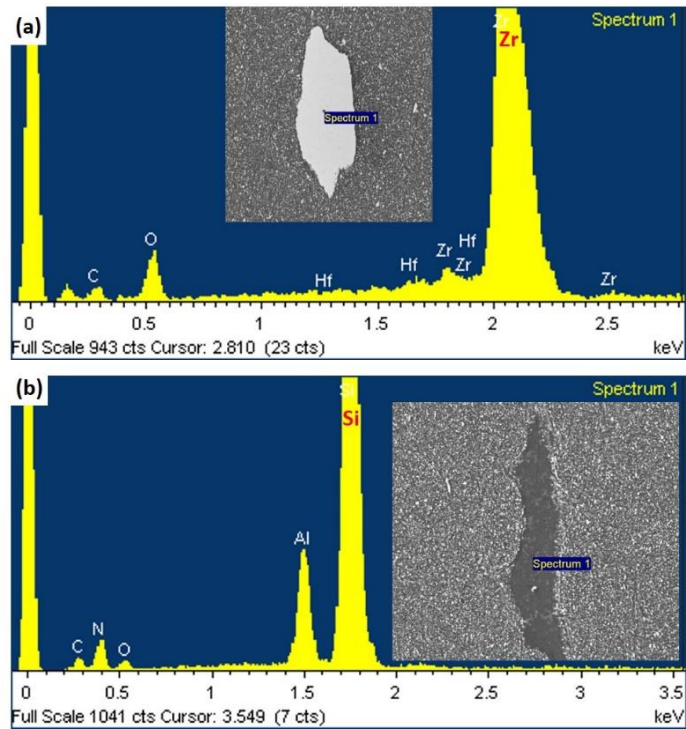
Şekil 1.83. Şekil 1.80(a)'da (a) siyah ok ile, (b) beyaz ok ile gösterilen bölgelerin EDX nokta analizi
