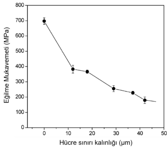
Şekil 1.26. Eğilme mukavemetinin hücre sınırı kalınlığına göre değişimi [66]
