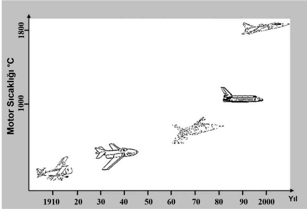
Şekil 1.4. Son yüzyılda jet motorlarında kullanılan malzemelerin yüksek sıcaklık mukavemetinin değerlendirilmesi [26]
