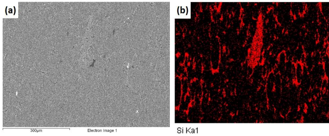
Şekil 1.76. (a) AlZr-%10 uBeZr numunesinin kesitinden alınan BSE-SEM görüntüsü, (b) aynı yerden yapılan EDX haritalama analizi ile elde edilen Si elementel haritası
