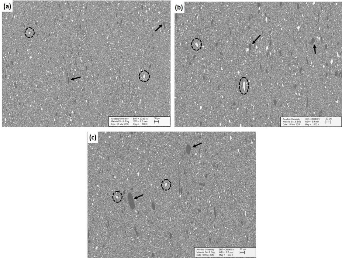
Şekil 2.2. Hacimce (a) %1, (b) %3, (c) %5 nano \text{Si}_3\text{N}_4 içeren numunelere ait BSE-SEM görüntüleri. Beyaz renkli \text{ZrO}_2 ve gri renkli \text{Al}_2\text{O}_3 toprakları sırasıyla daire ve oklarla gösterilmiştir.
