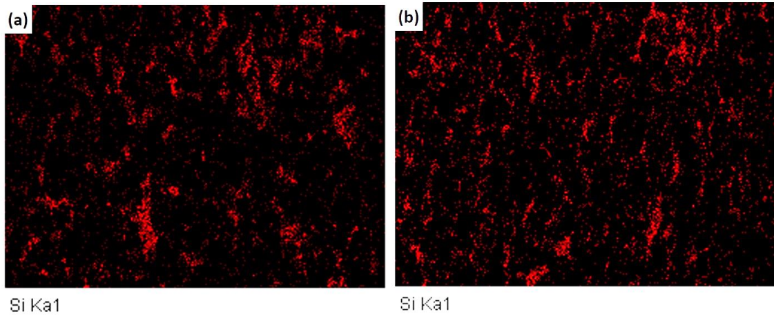
Şekil 1.81. Kaplama tozlarının dondurarak kurutma yöntemiyle üretildiği (a) AlZr-%10 ubeZr, (b) AlZr-%10 nanoZr numunelerine ait Si elementel haritaları
