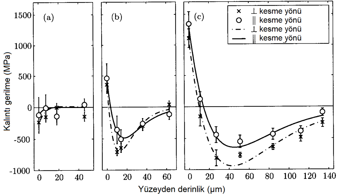
Şekil 1.8. Inconel 718'in SiC visker takviyeli alümina kesici uç ile tornalanması. 0,06 mm/dev ilerleme hızı ve (a) 10 m/dk, (b) 410 m/dk, (c) 810 m/dk kesme hızları için kalıntı gerilme derinlik profilleri [39]
