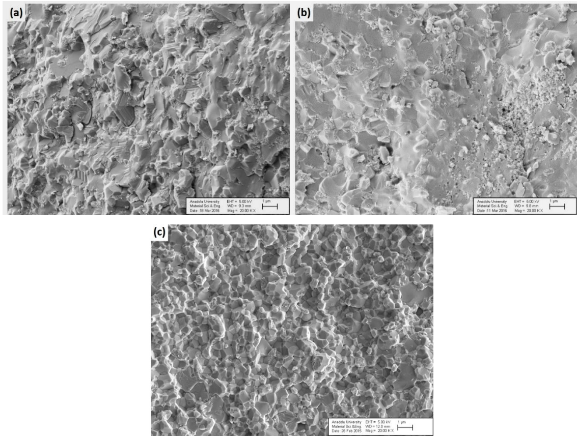
Şekil 1.108. Düşük boyutlu \text{Al}_2\text{O}_3\text{--ZrO}_2 granülleri ile (a) hacimce %5 ve (b) hacimce %10 olacak şekilde dondurarak kurutma yöntemiyle yapılan denemelere ve (c) AlZr matrise ait numunelerin kırık yüzeyinden 20000x büyütmede alınan SE-SEM görüntüleri
