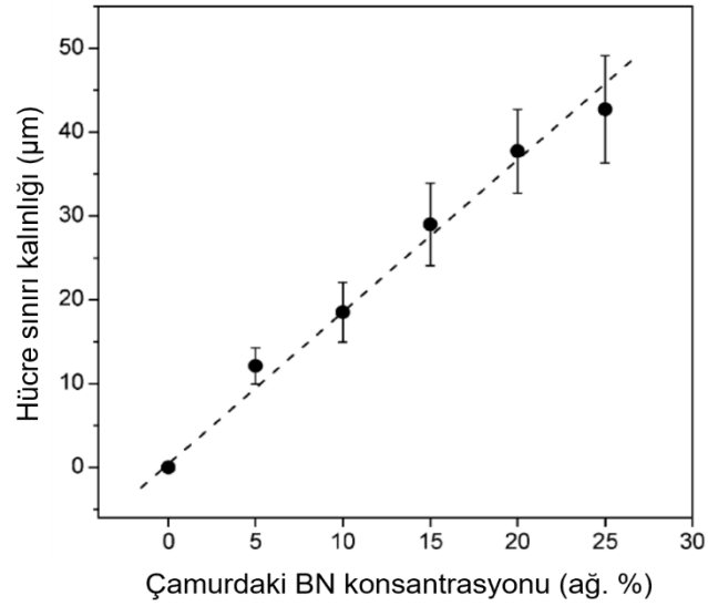
Şekil 1.23. Hücre sınırı kalınlığının çamurdaki BN konsantrasyonuna bağlı değişimi [66]
