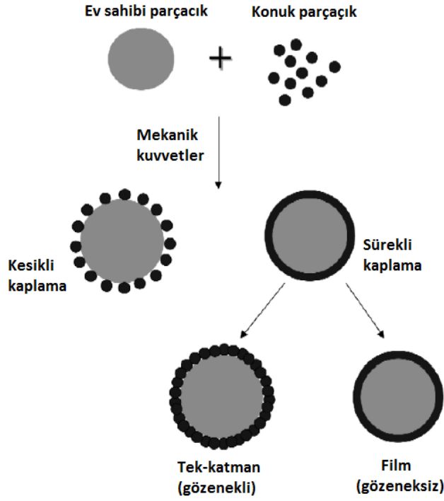
Şekil 1.37. Kuru parçacık kaplama yönteminin şematik gösterimi
