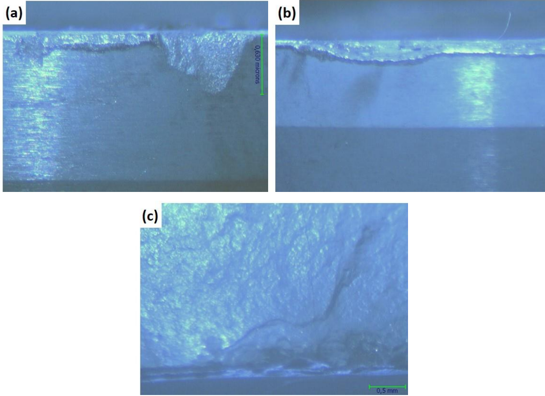
Şekil 1.58. (a) V_c = 250 m/dk, f = 0,15 mm/dev, a_p = 0,1 mm, (b) V_c = 200 m/dk, f = 0,20 mm/dev, a_p = 1,75 mm, (c) V_c = 300 m/dk, f = 0,15 mm/dev, a_p = 1,75 mm kesme koşulları ile test edilen AlZr-%15 nanoZr numunelerinin aşınma profilleri
