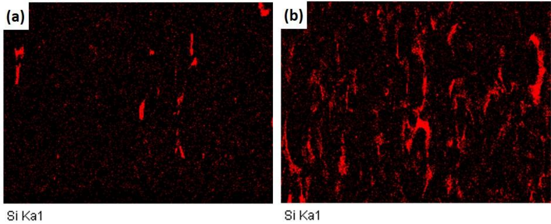
Şekil 1.96. 250 dev/dk dönme hızında (a) 1 dk, (b) 30 dk süreyle karıştırılan AlZr-%10 uBeZr numunelerinin EDX haritalama tekniği ile elde edilen Si elementel haritaları
