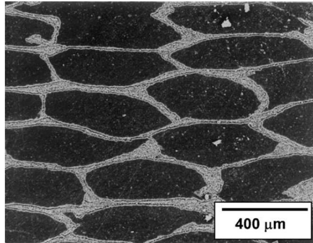
Şekil 1.24. \text{Si}_3\text{N}_4 / BN fibröz monolitinin temsili SEM kesit görüntüsü [66]
