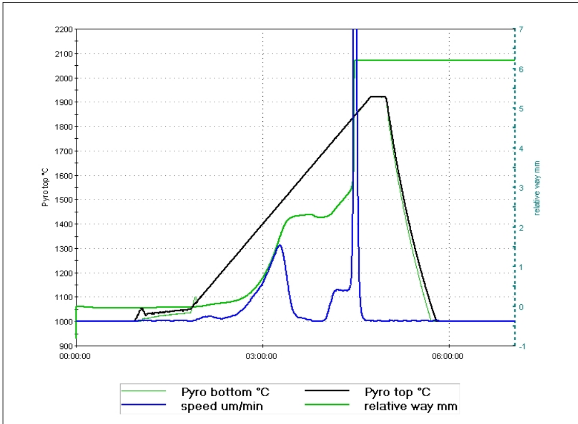
Şekil 3.1. Hacimce %3 nano \text{Si}_3\text{N}_4 içeren nano kompozit numunesine ait dilatometre eğrisi
