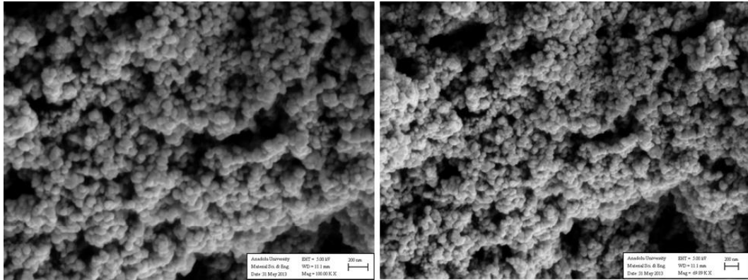
Şekil 1.35. ZrO 2 tozunun SE modunda alınmış SEM görüntüleri
