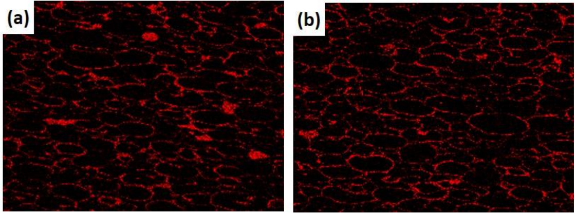
Şekil 1.65. (a) Yalnızca su, (b) su-PEG karışımı ile üretilen SL500-%15 Zr numunelerine ait Zr haritaları
