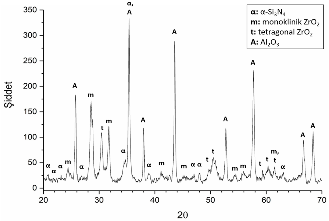
Şekil 1.28. CF1 kodlu fibröz monolit kesici uca ait XRD paterni
