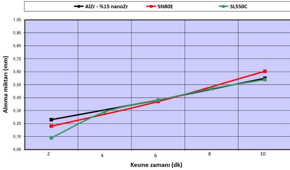
Şekil 1.59. GGG 40 malzemesinin işlenmesi sonucu ölçülen aşınma miktarlarının kesme zamanına göre değişimi
