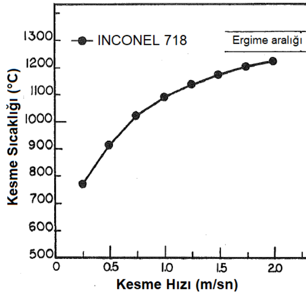
Şekil 1.10. Inconel 718 parçanın Al_2O_3 - TiC kesici uçla işlenmesinde kesme hızının kesme sıcaklığına etkisi (0,1 mm/dev ilerleme, 1 mm kesme derinliği) [43]
