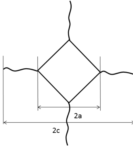
Şekil 1.41. Vickers sertlik ucunun numune yüzeyinde oluşturduğu iz ve çatlakların şematik gösterimi
