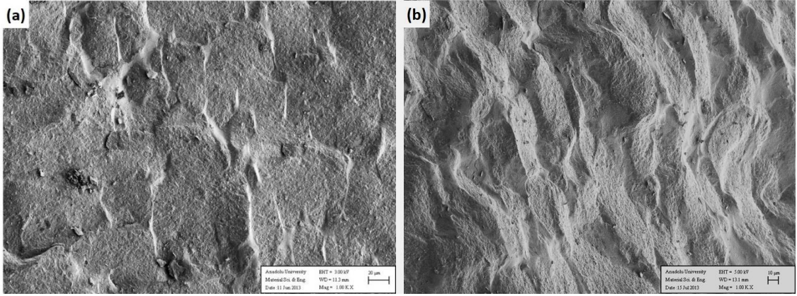
Şekil 1.51. SN80 granüllerinin (a) hacimce %10, (b) hacimce %20 \text{Si}_3\text{N}_4\text{-ZrO}_2 kaplanmasıyla üretilen numunelerin kırık yüzey SE-SEM görüntüleri
