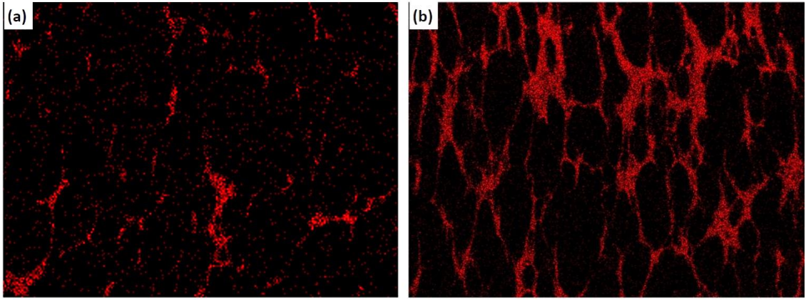
Şekil 1.50. SN80 granüllerinin (a) hacimce %10, (b) hacimce %20 \text{Si}_3\text{N}_4\text{-ZrO}_2 kaplanmasıyla üretilen numunelerin EDX haritalama yöntemiyle elde edilen Si elementel harita görüntüleri
