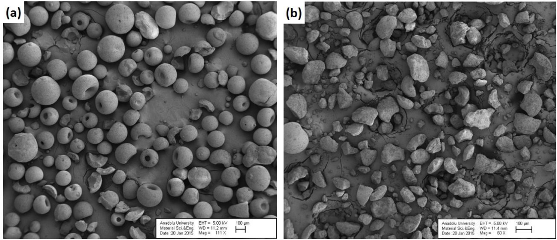
Şekil 1.95. 250 dev/dk dönme hızında (a) 1 dk, (b) 30 dk süreyle karıştırılan AlZr-%10 uBeZr granüllerinin SE-SEM görüntüleri
