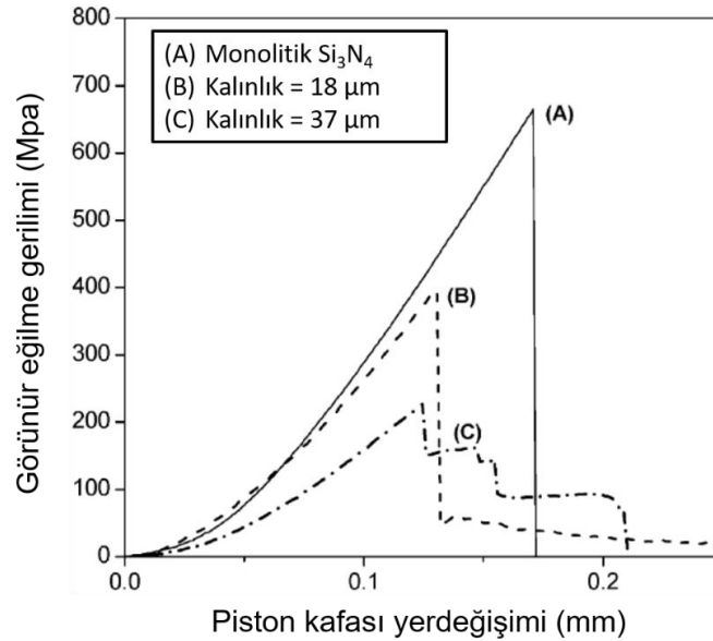
Şekil 1.25. (A) Monolitik, (B) 18 \mu\text{m} , (C) 37 \mu\text{m} hücre sınırı kalınlığına sahip numunelerin eğilme tepkisi [66]
