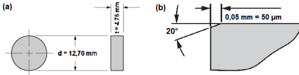
Şekil 1.42. (a) Kesici ucun geometrisi, (b) pah açısı ve uzunluğu
