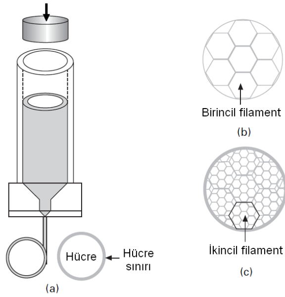
Şekil 1.19. Fibröz monolitlerin üretimi için kullanılan "ortak ekstrüzyon ile mikro üretim" yönteminin şematik gösterimi: (a) ortak ekstrüzyon, (b) birincil filamentin birleştirilmesi, (c) ikinci ortak ekstrüzyon sonrası filament [54]
