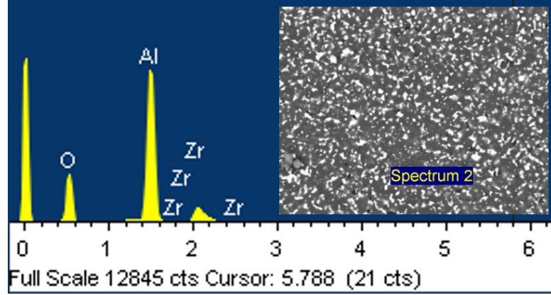
Şekil 1.30. CF1 kodlu fibröz monolit kesici ucun hücre içerisinde alınmış EDX analizi sonucu
