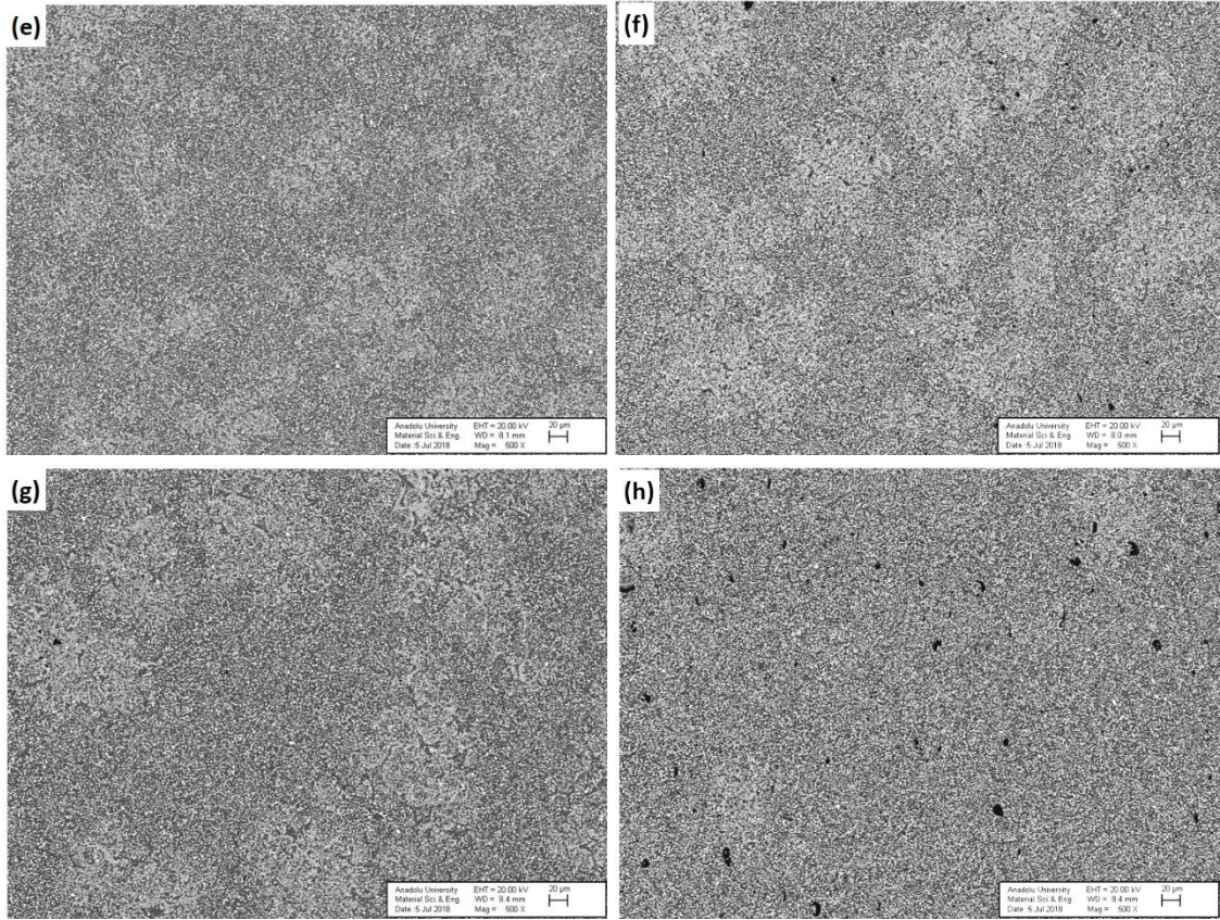
Şekil 3.7 (Devam) Siklonlarla yapılan ve hacimce %5 UBE \text{Si}_3\text{N}_4\text{-ZrO}_2 içerip (a) GPS ile üretilen, (b) PLS ile üretilen, granüllerle yapılan ve hacimce %5 UBE \text{Si}_3\text{N}_4\text{-ZrO}_2 içerip (c) GPS ile üretilen, (d) PLS ile üretilen, siklonlarla yapılan ve hacimce %10 UBE \text{Si}_3\text{N}_4\text{-ZrO}_2 içerip (e) GPS ile üretilen, (f) PLS ile üretilen, granüllerle yapılan ve hacimce %10 UBE \text{Si}_3\text{N}_4\text{-ZrO}_2 içerip (g) GPS ile üretilen, (h) PLS ile üretilen numunelere ait BSE-SEM görüntüleri
