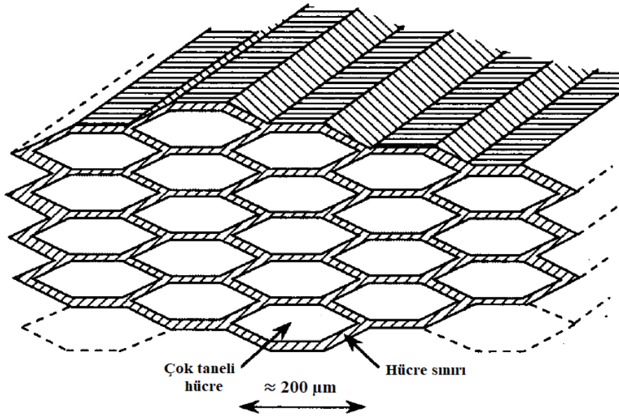
Şekil 1.17. Güçlü hücre ile zayıf hücre sınırını içeren fibröz monolitik yapının şematik gösterimi [24]
