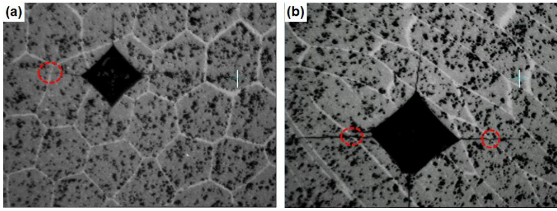
Şekil 1.34. Fibröz monolit kesici ucun parlatılmış kesitine Vickers indent ucu ile (a) 5 kg, (b) 10 kg yük uygulandığında oluşan indent izleri ve çatlak ilerlemesi
