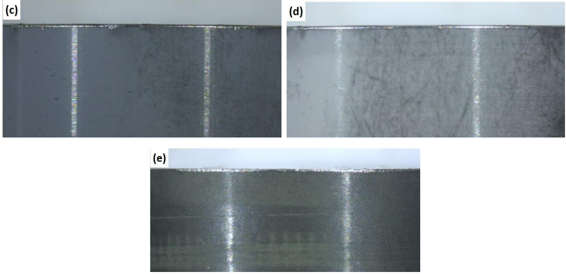
Şekil 2.9. (Devam) Test edilen (a) hacimce %1, (b) hacimce %3, (c) hacimce %5 nano \text{Si}_3\text{N}_4 içeren nano kompozitlerin ve (d) \text{AlZr} matris, (e) \text{Al}_2\text{O}_3\text{--SiC}_v kesici uçların aşınma profilleri
