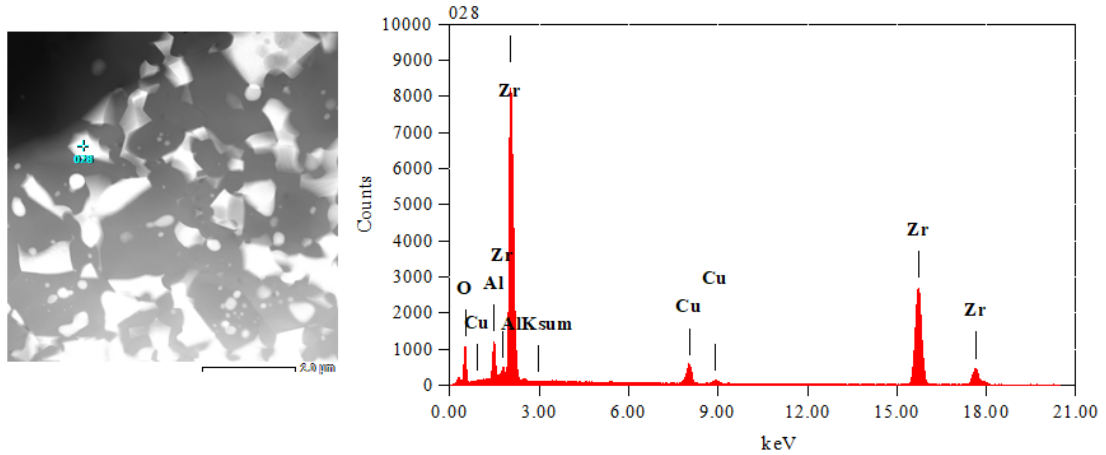
Şekil 1.33. ZrO 2 tanesine yapılan TEM-EDX analizi sonuçları
