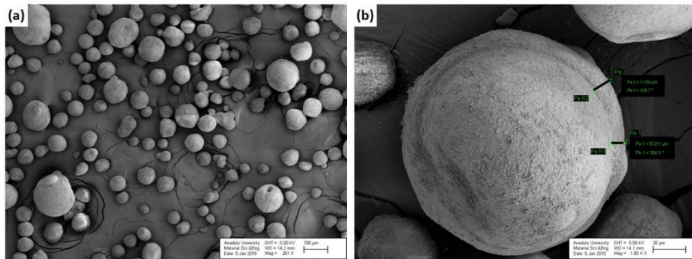
Şekil 1.72. Şiddetli karıştırıcı 1000 dev/dk hızda 30 dk süre ile yapılan SL500 - %15 ubeZr numunesine ait granüllerinin SE-SEM görüntüleri (a) 261x, (b) 1800x
