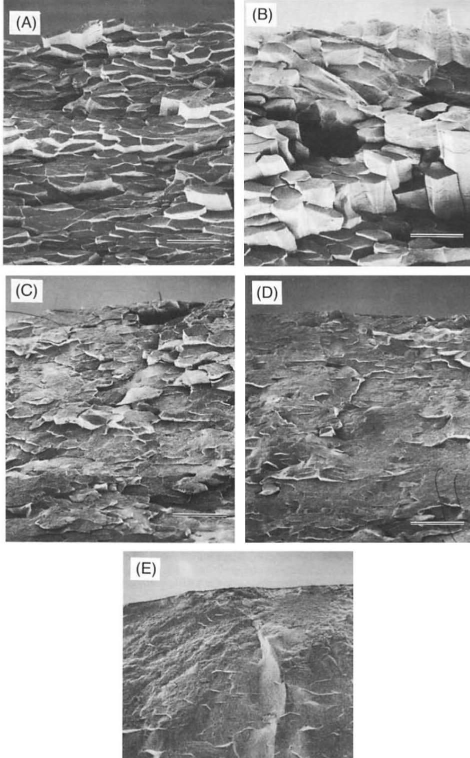
Şekil 1.20. Hücre sınırı (A) %100, (B) %80, (C) %60, (D) %40, (E) %20 grafit içeren SiC esaslı fibröz monolitlerin kırık yüzeyleri [58]
