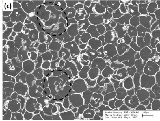
Şekil 1.68. (Devam) SL500 - %15 Zr numunesinin (a) 1000 dev/dk, (b) 1500 dev/dk, (c) 3000 dev/dk dönme hızıyla yapılan denemelerine ait numunelerin BSE-SEM görüntüleri
