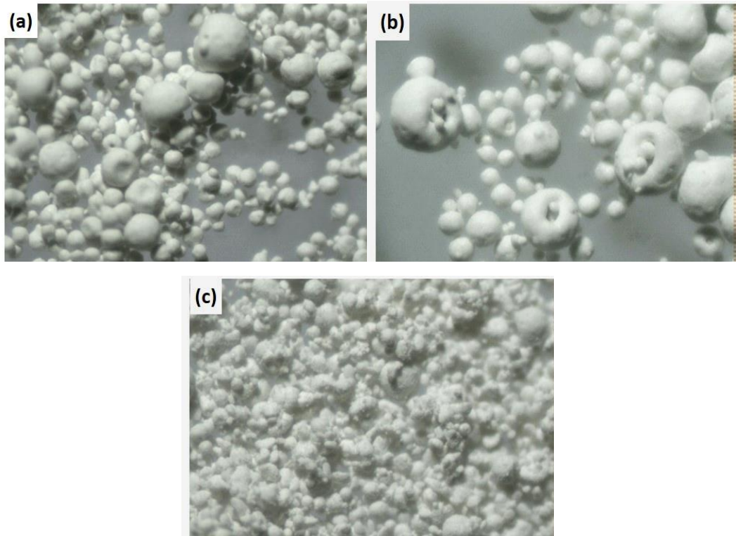
Şekil 1.69. SL500 - %15 Zr numunesinin 5 dk süre ile (a) 1000 dev/dk, (b) 1500 dev/dk, (c) 3000 dev/dk dönme hızıyla yapılan denemelere ait granüllerin stereo mikroskop görüntüleri
