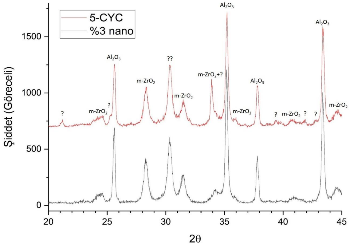
Şekil 3.4. Hacimce %5 nano \text{Si}_3\text{N}_4 içeren numune ile siklonlara hacimce %5 \text{Si}_3\text{N}_4 - \text{ZrO}_2 kaplanarak elde edilen numunenin XRD analizleri
