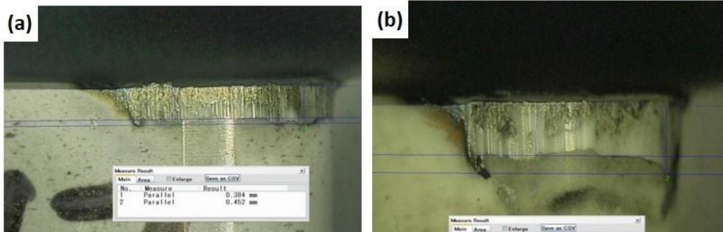
Şekil 1.60. GGG 40 malzemesinin işlenmesi sonucu oluşan aşınma profilleri (a) AlZr-%15 nanoZr, (b) SN80E, (c) SL550C
