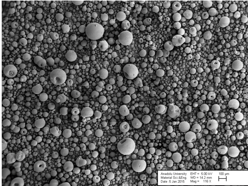
Şekil 1.66. SL500 granüllerinin SE-SEM görüntüsü
