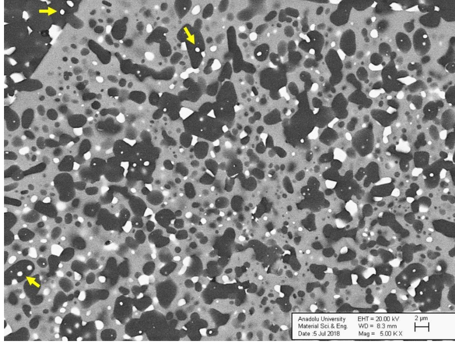
Şekil 3.8. Siklonlarla yapılan ve hacimce %5 UBE \text{Si}_3\text{N}_4\text{-ZrO}_2 içerip GPS ile üretilen numunenin \text{Si}_3\text{N}_4\text{-ZrO}_2 bölgesinden 5000x büyütmede alınan BSE-SEM görüntüsü. Düşük boyutlu ve mükemmel şekilde yuvarlak olan \text{ZrO}_2 taneleri oklarla gösterilmiştir.
