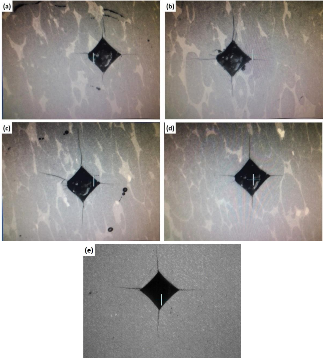
Şekil 1.46. (a) AlZr-%15 ubeZr, (b) yağ ilaveli AlZr-%15 ubeZr, (c) AlZr-%15 nanoZr, (d) yağ ilaveli AlZr-%15 nanoZr, (e) AlZr matris numunelerine ait Vickers indent izi ve oluşan çatlaklar
