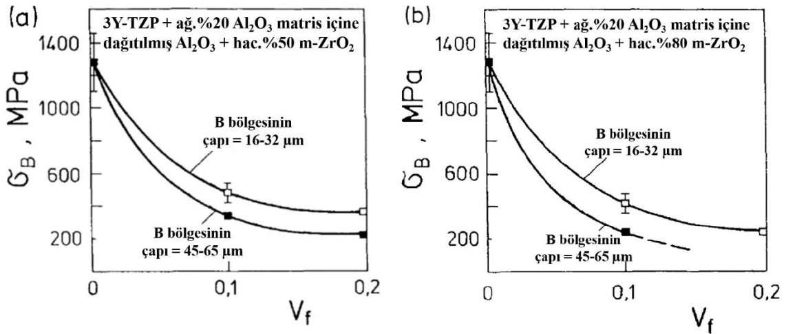
Şekil 1.12. 3Y-TZP + ağ.%20 Al 2 O 3 matris içine dağıtılmış (a) Al 2 O 3 + hac.%50 m-ZrO 2 , (b) Al 2 O 3 + hac.%80 m-ZrO 2 dubleks seramiklerin mukavemeti [53]
