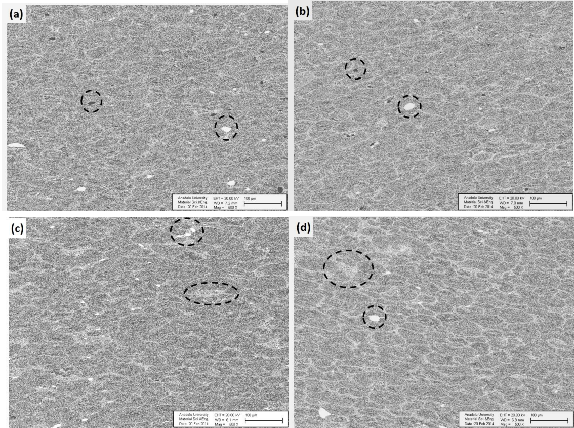
Şekil 1.56. (a) AlZr-%15 ubeZr, (b) yağ ilaveli AlZr-%15 ubeZr, (c) AlZr-%15 nanoZr, (d) yağ ilaveli AlZr-%15 nanoZr numunelerinin BSE-SEM görüntüleri. \text{Si}_3\text{N}_4 ve \text{ZrO}_2 topakları dairelerle gösterilmiştir.
