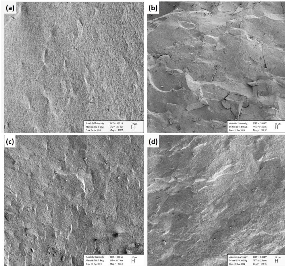
Şekil 1.53. Bilyalı değirmende yapılan (a) yağ ilavesiz, (b) 2 sa yağ ile karıştırılan SN80-%15 ubeZr numunelerinin ve (c) yağ ilavesiz, (d) 2 sa yağ ile karıştırılan SN80-%15 nanoZr numunelerinin kırık yüzey SE-SEM görüntüleri
