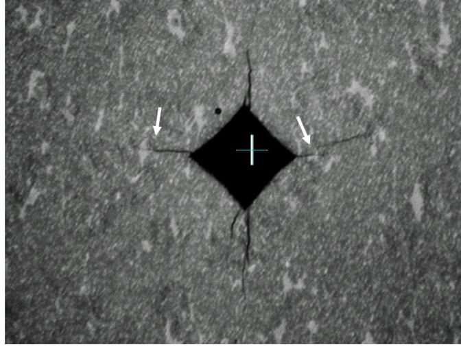
Şekil 1.97. Dondurarak kurutma yöntemiyle üretilen AlZr - \%10\ ubeZr numunesine ait Vickers indent izi ve oluşan çatlakların optik mikroskop görüntüsü. çatlakların heterojen bölgelerle etkileşimi oklarla gösterilmiştir.
