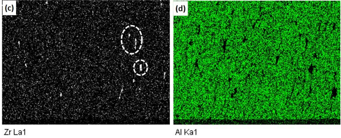
Şekil 1.84. (Devam) Toz ağırlığının 1,5 katı kadar bilye ile karıştırılmış \text{Si}_3\text{N}_4\text{-ZrO}_2 tozunun \text{Al}_2\text{O}_3\text{-ZrO}_2 granülleri etrafına kaplanmasıyla elde edilen numunenin (a) BSE-SEM görüntüsü ve aynı yerden yapılan EDX haritalama analizi ile elde edilen (b) Si, (c) Zr, (d) Al elementel haritaları. Si bölgeleri oklarla, Zr bölgeleri dairelerle gösterilmiştir.
