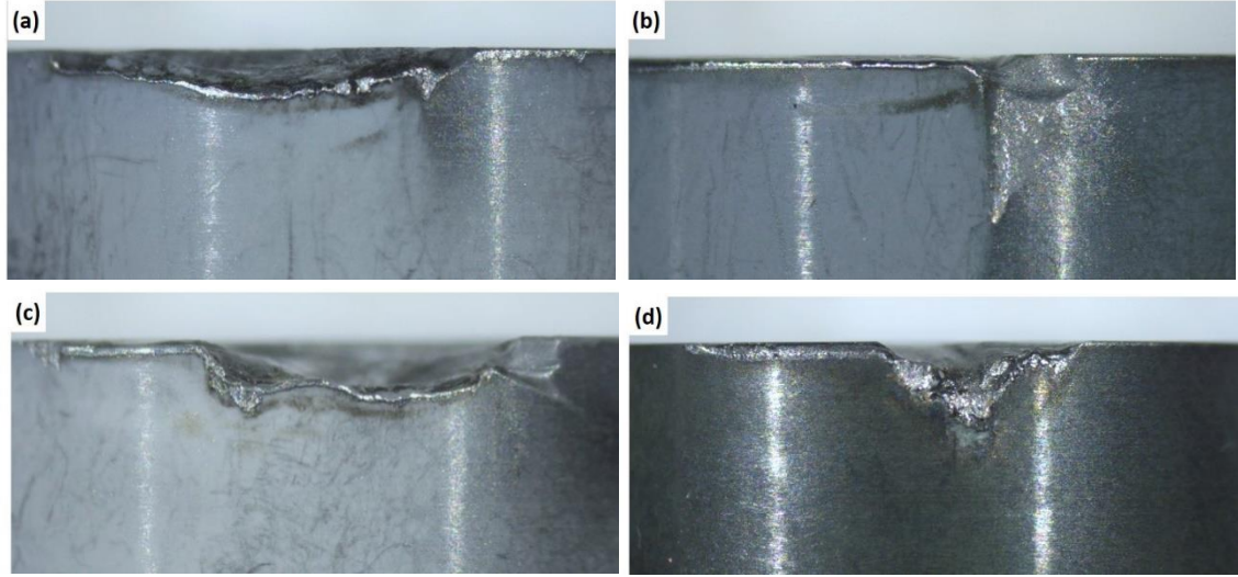
Şekil 2.8. Test edilen (a) hacimce %1, (b) hacimce %3 nano \text{Si}_3\text{N}_4 içeren nano kompozitlerin ve (c) \text{AlZr} matris, (d) \text{Al}_2\text{O}_3\text{--SiC}_v kesici uçların aşınma profilleri
