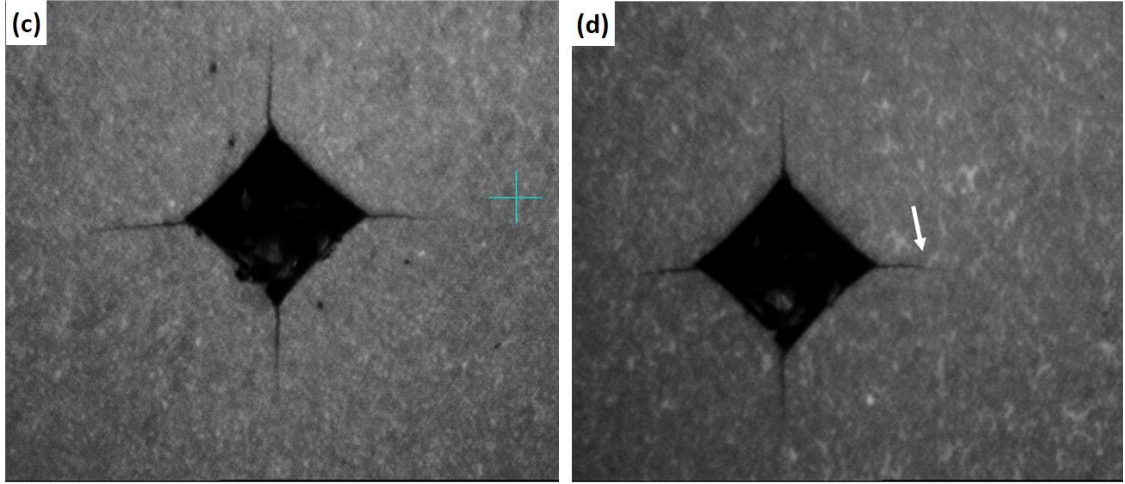
Şekil 1.98. (Devam) Düşük boyutlu \text{Al}_2\text{O}_3\text{-ZrO}_2 granülleri ile (a) hacimce %5, (b) hacimce %10 ve siklonlarla (c) hacimce %5, (d) hacimce %10 olacak şekilde dondurarak kurutma yöntemiyle yapılan denemelere ait numunelerin Vickers indent izi ve oluşan çatlaklar. Çatlakların heterojen bölgelerle etkileşimi şekil üzerinde ok ile gösterilmiştir.
