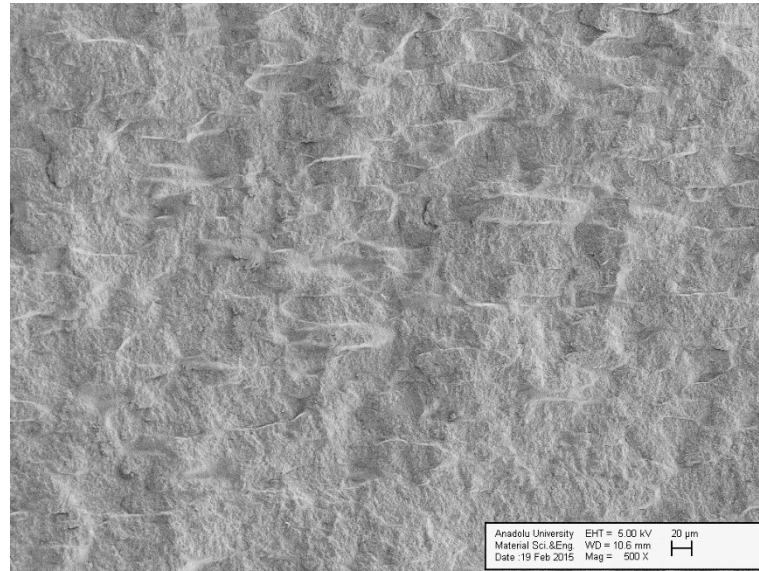
Şekil 1.86. Ağırlıkça %5 su-PEG karışımı içeren AlZr-%10 nanoSN numunesinin kırık yüzeyine ait SE-SEM görüntüsü
