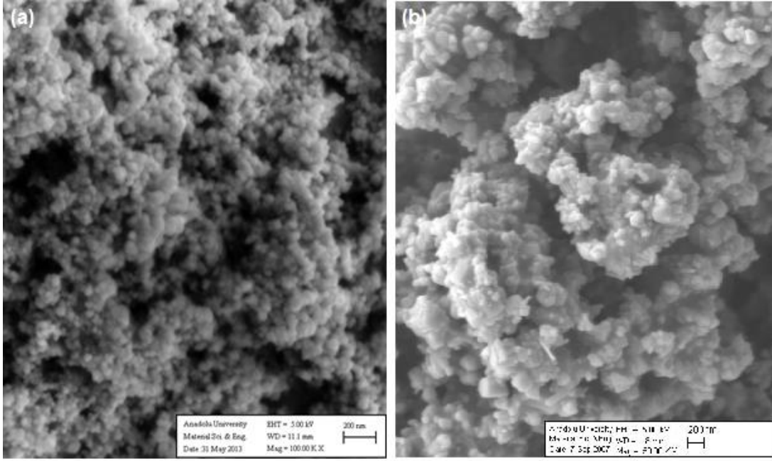
Şekil 1.36. (a) Grade C, (b) SN-E10 \text{Si}_3\text{N}_4 tozlarının ikincil elektron modunda alınmış SEM görüntüleri
