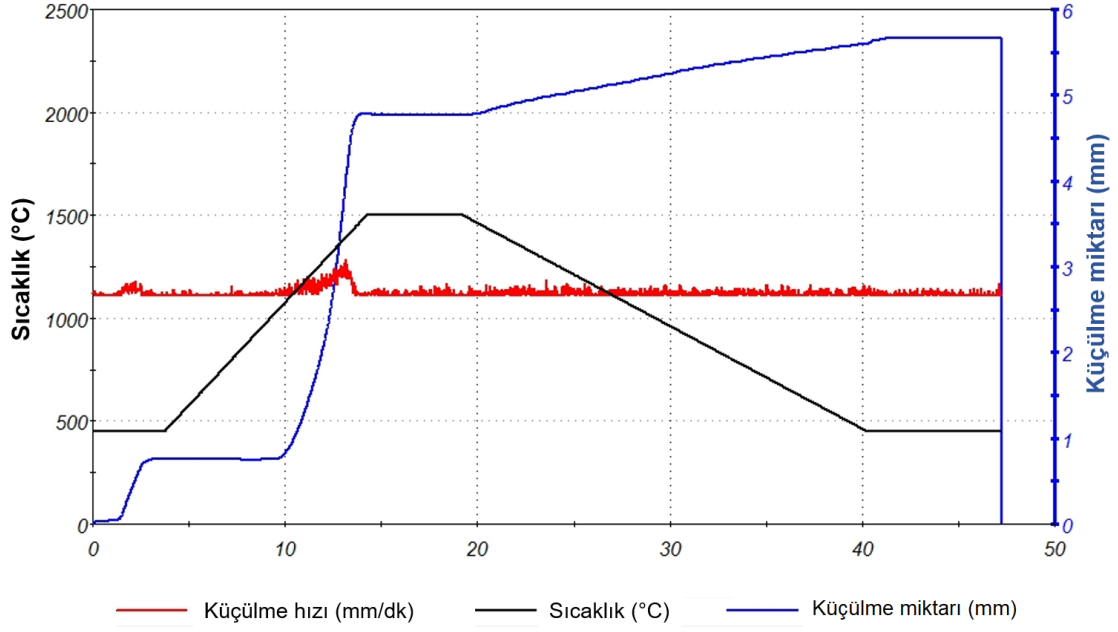
Şekil 1.40. SPS ile sinterleme sırasında kayıtları edilen parametrelerin değışimini gösteren grafik
