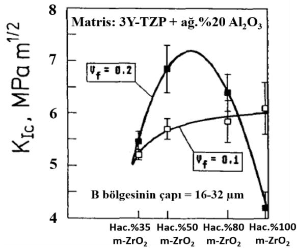
Şekil 1.15. Farklı basınç bölgesi miktarlarına sahip dubleks seramiklerin kırılma tokluğu [53]
