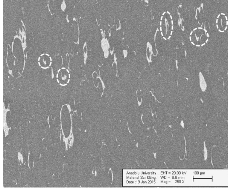
Şekil 1.91. 20 dk süreyle karıştırılan SL500 - %10 ubeZr numunesine ait BSE-SEM görüntüsü. Beyaz ZrO 2 bölgeleri dairelerle gösterilmiştir.
