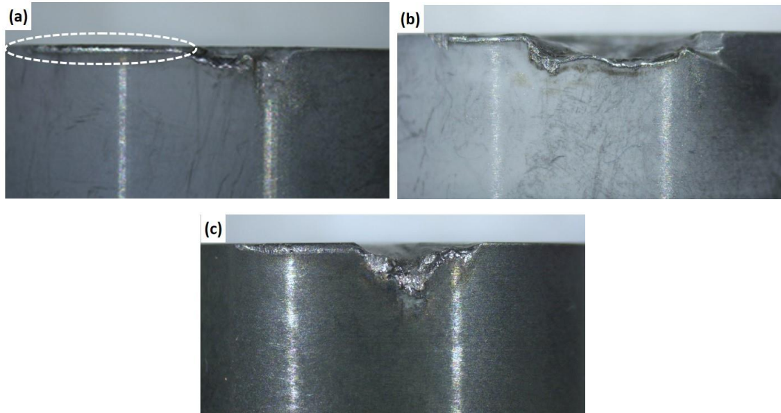
Şekil 1.110. Test edilen (a) AlZr-%5 ubeZr, (b) AlZr matris, (c) Al 2 O 3 -SiC v kesici uçların aşınma profilleri. Yanıl aşınma bölgesi daire ile gösterilmiştir.
