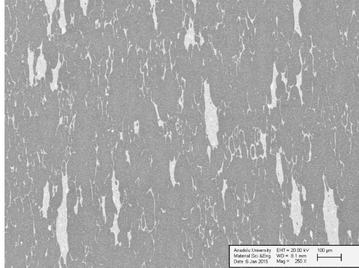
Şekil 1.73. Şiddetli karıştırıcıda 215 dev/dk hızda 30 dk süre ile yapılan SL500 - %15 ubeZr numunesine ait BSE-SEM görüntüsü
