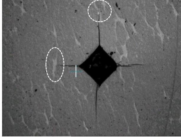
Şekil 1.44. SN80-%10 nanoZr numunesine ait Vickers indent izi ve oluşan çatlaklar. Çatlakların heterojen bölgelerle etkileşimi dairelerle gösterilmiştir.
