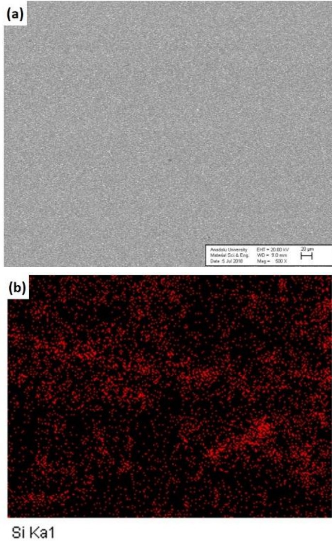
Şekil 2.6. 500 dev/dk dönme hızıyla üretilen ve hacimce %3 nano \text{Si}_3\text{N}_4 içeren nano kompozitin (a) BSE-SEM görüntüsü, (b) EDX haritalama analizi ile elde edilen Si elementel haritası
