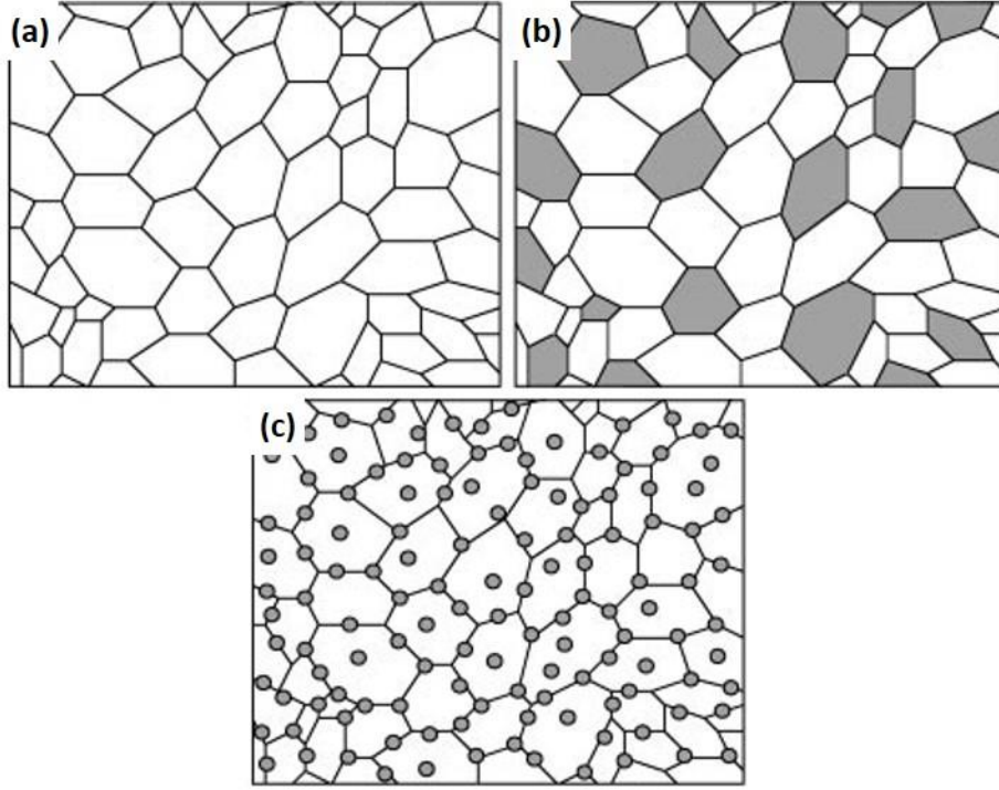
Şekil 2.1. Nano-seramiklerin temel tipleri: (a) hepsi nano, tek faz, (b) hepsi nano, iki faz, (c) mikro/nano, iki faz: Nano faz tanelere ve tane sınırlarına dağılmış [100]
