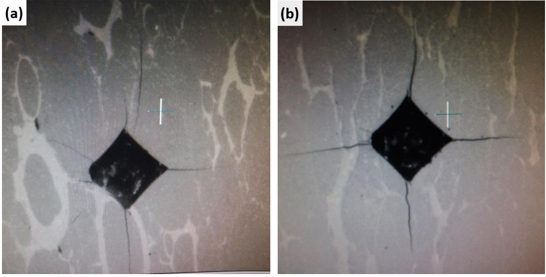
Şekil 1.45. (a) SN80-%10 ubeZr, (b) SN80-%10 nanoZr numunelerine ait Vickers indent izleri ve oluşan çatlaklar
