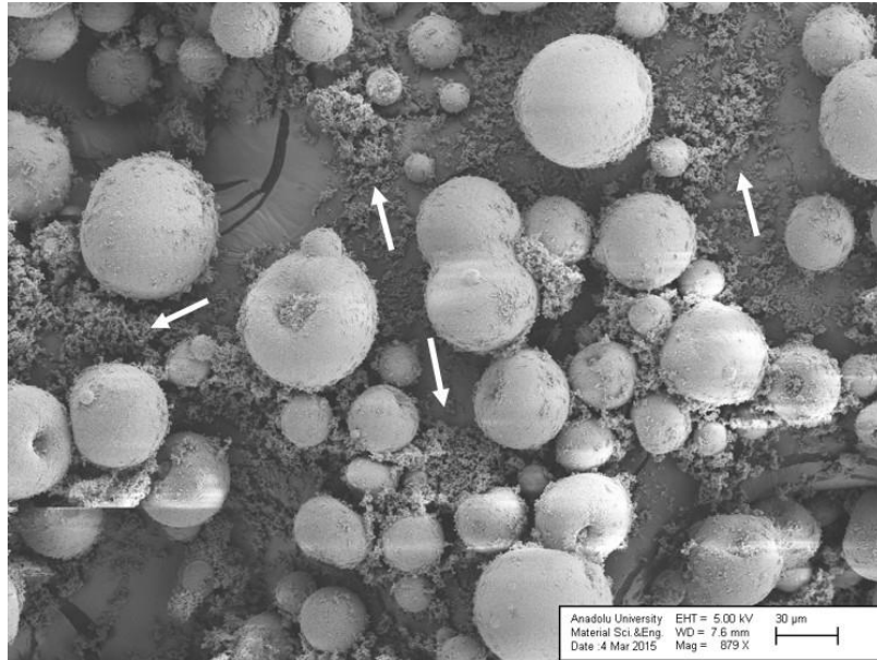
Şekil 1.99. Dondurarak kurutma yöntemiyle üretilen \text{AlZr}\text{-}\%10\text{ ubeZr} granüllerine ait SE-SEM görüntüsü. kaplanmadan kalan tozlar oklarla gösterilmiştir.
