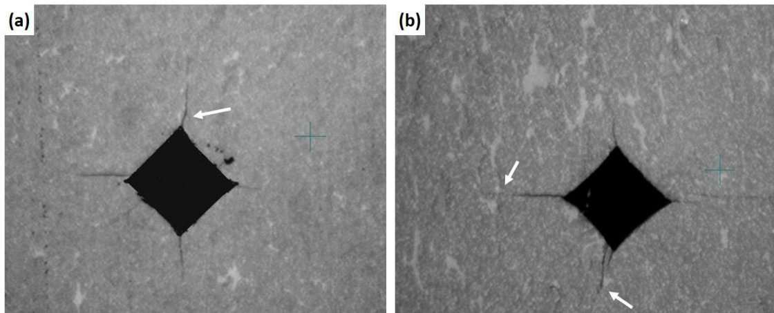
Şekil 1.98. Düşük boyutlu \text{Al}_2\text{O}_3\text{--ZrO}_2 granülleri ile (a) hacimce %5, (b) hacimce %10 ve siklonlarla (c) hacimce %5, (d) hacimce %10 olacak şekilde dondurarak kurutma yöntemiyle yapılan denemelere ait numunelerin Vickers indent izi ve oluşan çatlaklar. Çatlakların heterojen bölgelerle etkileşimi şekil üzerinde ok ile gösterilmiştir.
