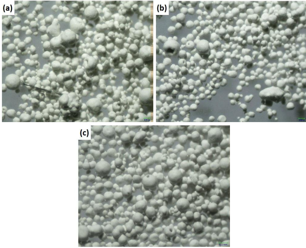
Şekil 1.71. SL500 - %15 ubeZr numunesinin şiddetli karıştırıcıda 1000 dev/dk dönme hızı ile (a) 5 dk, (b) 15dk, (c) 30 dk süreyle yapılan denemelere ait granüllerin stereo mikroskop görüntüleri
