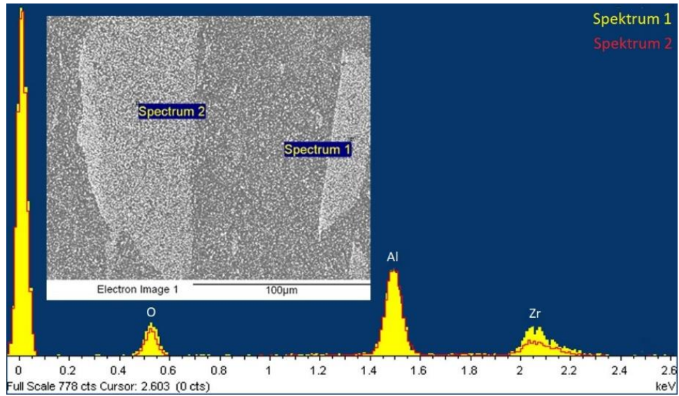
Şekil 3.13. Hacimce %1 nano \text{Si}_3\text{N}_4 içeren ve GPS ile üretilen numunenin EDX analizi
