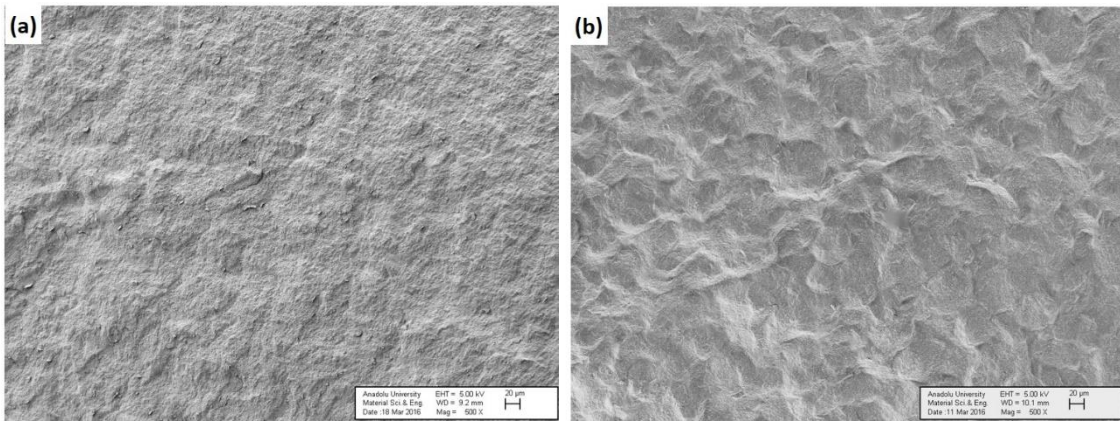
Şekil 1.107. Düşük boyutlu Al_2O_3-ZrO_2 granülleri ile (a) hacimce %5 ve (b) hacimce %10 olacak şekilde dondurarak kurutma yöntemiyle yapılan denemelere ait numunelerin kırık yüzeyinden 500x büyütmede alınan SE-SEM görüntüleri
