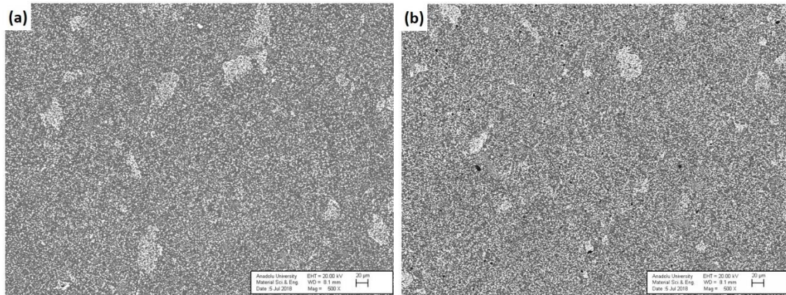
Şekil 3.12. Hacimce %1 nano \text{Si}_3\text{N}_4 içerip (a) GPS ile üretilen, (b) PLS ile üretilen, hacimce %3 nano \text{Si}_3\text{N}_4 içerip (c) GPS ile üretilen, (d) PLS ile üretilen numunelere ait BSE-SEM görüntüleri
