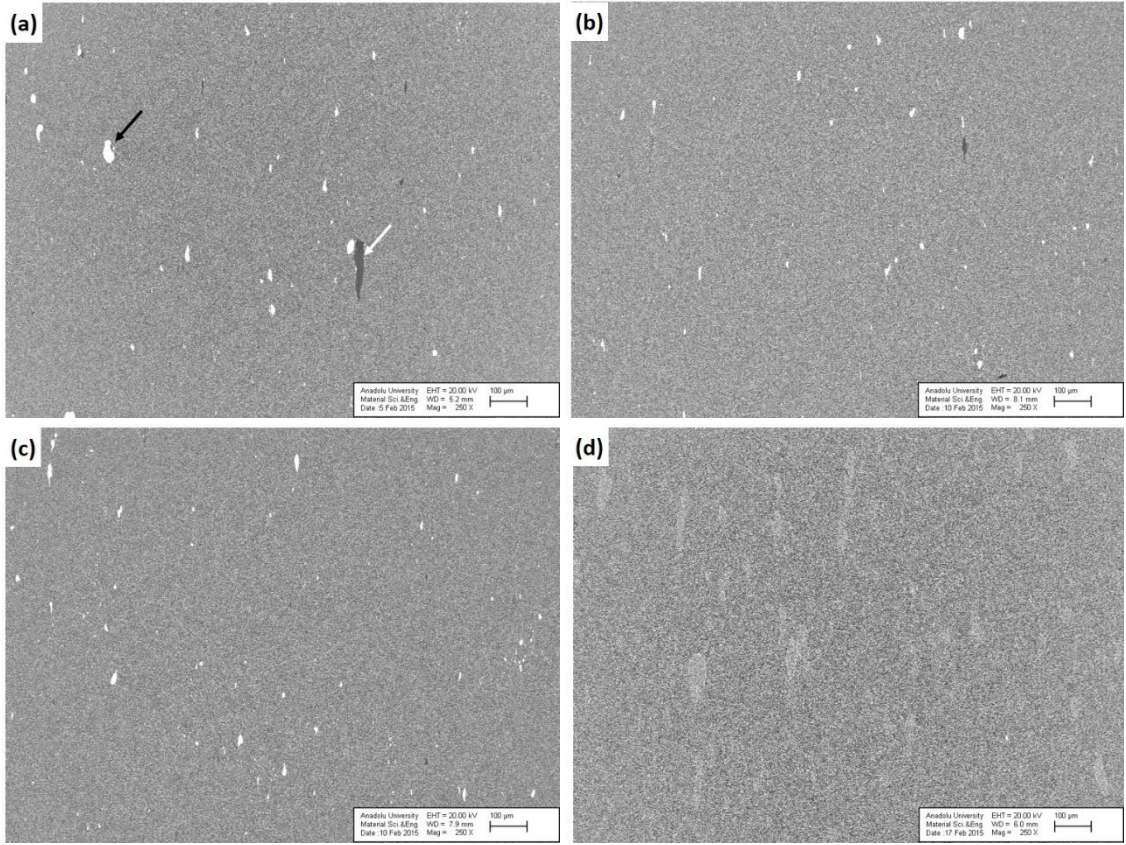
Şekil 1.82. (a) 3 adet bilyeyle 7 saat, (b) 3 adet bilyeyle 24 saat, (c) toz ağırlığının 1,5 katı kadar bilyeyle 24 saat, (d) toz ağırlığının 2,5 katı kadar bilyeyle 24 saat karıştırılan nano \text{Si}_3\text{N}_4\text{-ZrO}_2 toz karışımı ile yapılan denemelere ait numunelerin BSE-SEM görüntüleri. Heterojen \text{Si}_3\text{N}_4 ve \text{ZrO}_2 bölgeleri oklarla gösterilmiştir.
