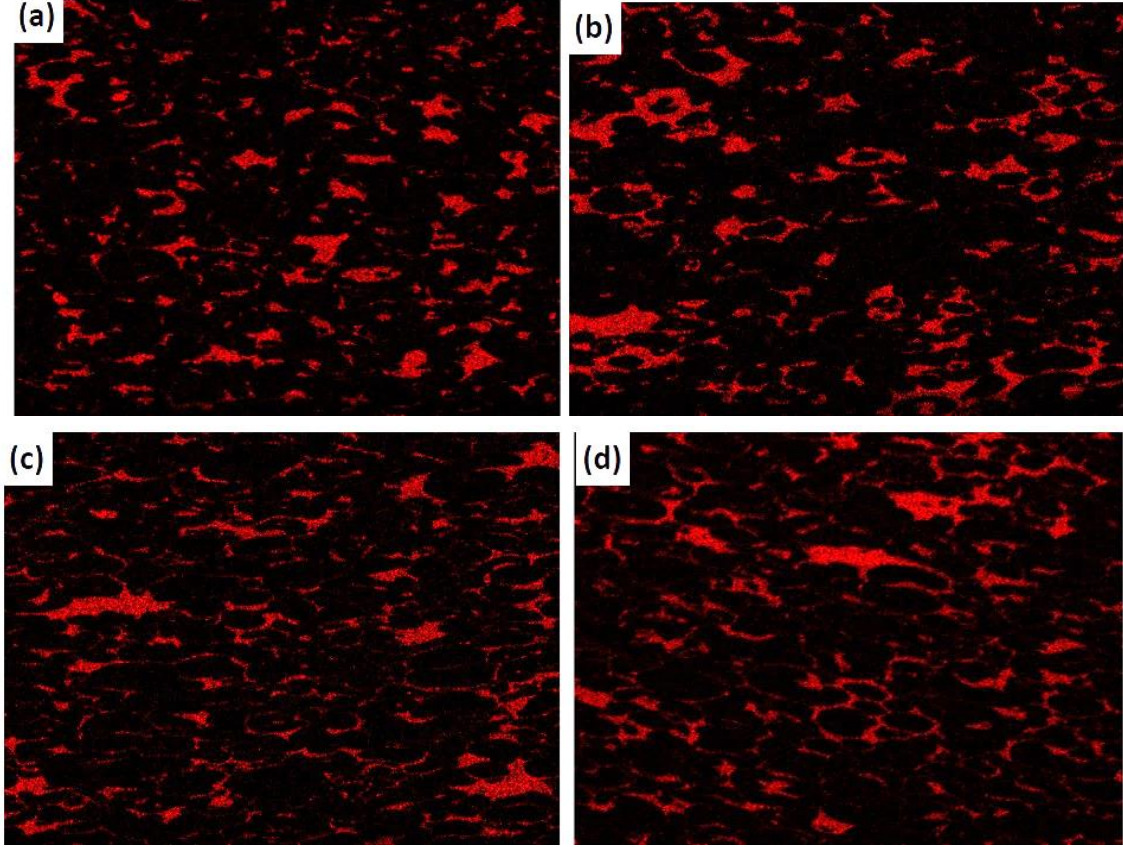
Şekil 1.57. (a) AlZr-%15 ubeZr, (b) yağ ilaveli AlZr-%15 ubeZr, (c) AlZr-%15 nanoZr, (d) yağ ilaveli AlZr-%15 nanoZr numunelerinin EDX haritalama yöntemiyle elde edilen Si elementel harita görüntüleri
