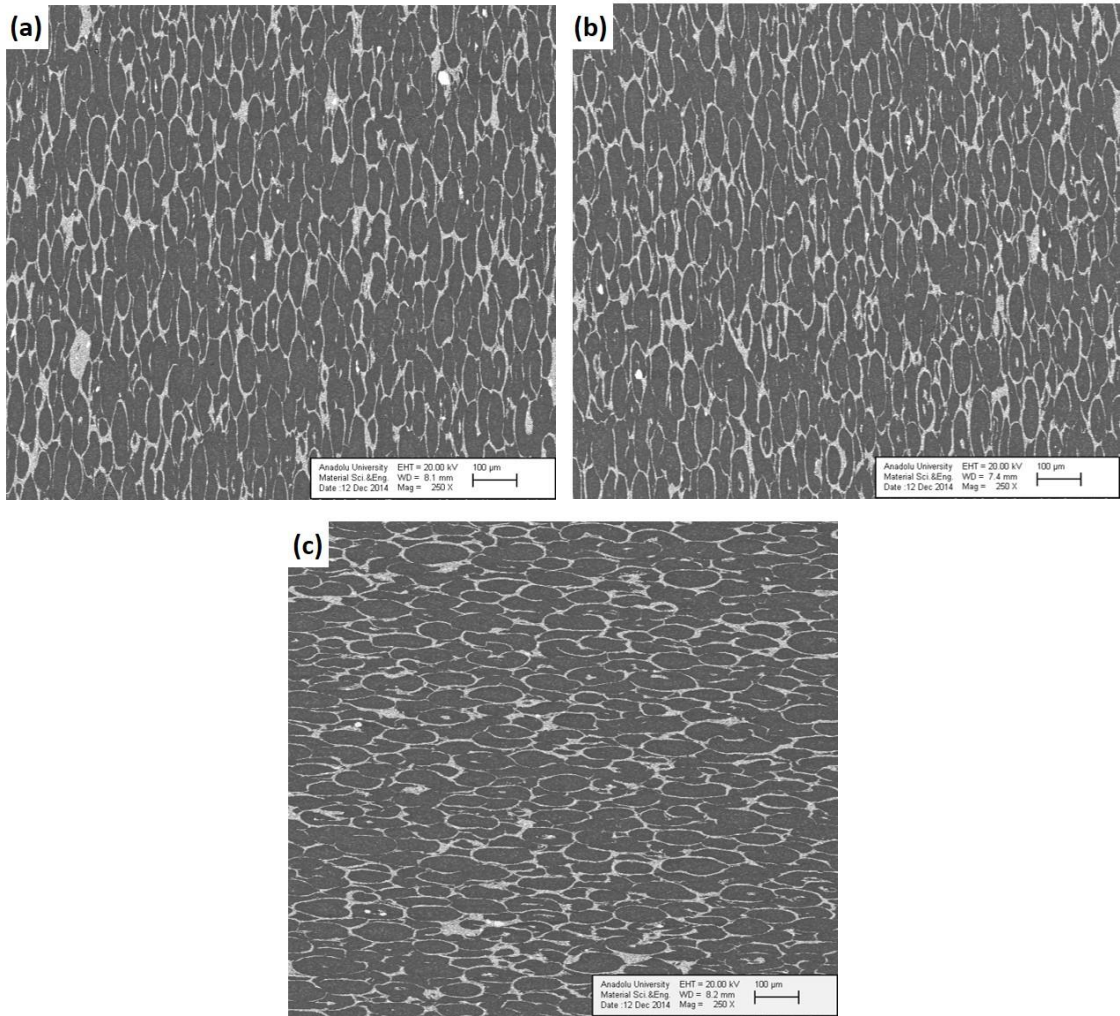
Şekil 1.70. SL500 - %15 ubeZr numunesinin şiddetli karıştırıcıda 1000 dev/dk dönme hızı ile (a) 5 dk, (b) 15dk, (c) 30 dk süreyle yapılan denemelere ait numunelerin BSE-SEM görüntüleri
