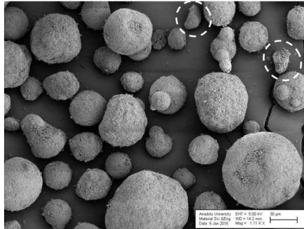
Şekil 1.74. Şiddetli karıştırıcıda 215 dev/dk hızda 30 dk süre ile yapılan SL500 - %15 ubeZr numunesine ait granüllerin SE-SEM görüntüsü. Granüllerden kopan parçalar dairelerle ile gösterilmiştir.
