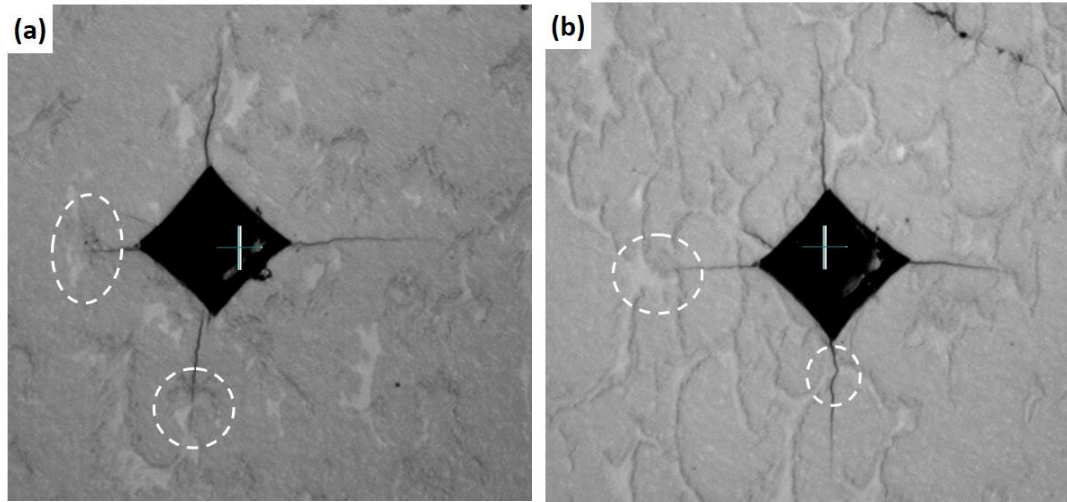
Şekil 1.62. Dondurarak kurutma yöntemiyle elde edilen \text{Si}_3\text{N}_4\text{-ZrO}_2 tozlarının \text{Al}_2\text{O}_3\text{-ZrO}_2 granüllerinin etrafına kaplanmasıyla elde edilen numunelerin Vickers indent izi ve oluşan çatlaklar
