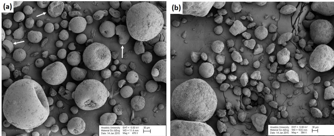
Şekil 1.90. (a) 10 dk, (b) 20 dk süreyle karıştırılan SL500 - %10 ubeZr numunesine ait granüllerin SE-SEM görüntüleri. Paralanan granüllerden kopan paralar oklarla gösterilmiştir.
