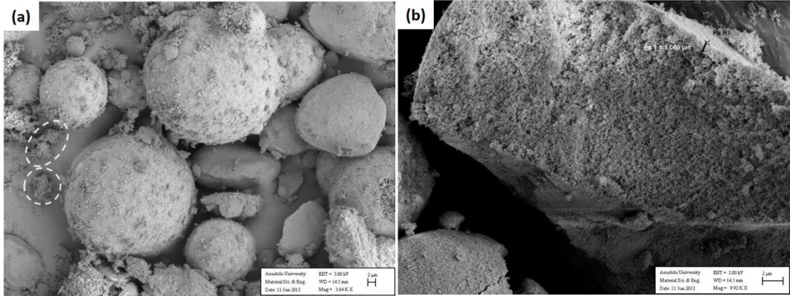
Şekil 1.48. Hacimce %10 \text{Si}_3\text{N}_4\text{-ZrO}_2 kaplanan SN 80 granüllerinin SE-SEM görüntüleri. (a)3640x, (b) 9920x. Kaplanmadan kalan tozlar dairelerle gösterilmiştir.
