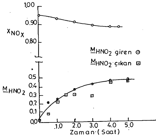
Şekil 3.11. Delikli üç tepsi içeren bir kolonda, toplam \text{NO}_x dönüşümü ve sıvı fazdaki \text{HNO}_2 değişiminin yatışkın duruma erişmesi (Counce and Perona, 1979a, 1980)
