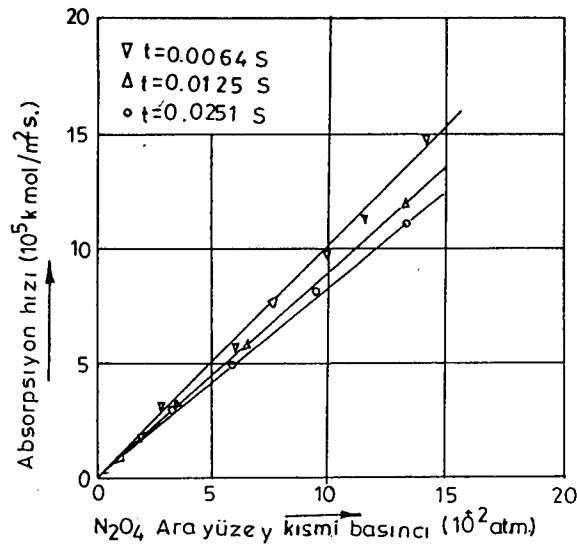
Şekli 3.6. 20 °C'da, laminer bir jet absorplayicisinde absorpsiyon hızının \text{N}_2\text{O}_4 arayüzey kısmi basıncına bağımlılığı (Kramers, et al., 1961).
