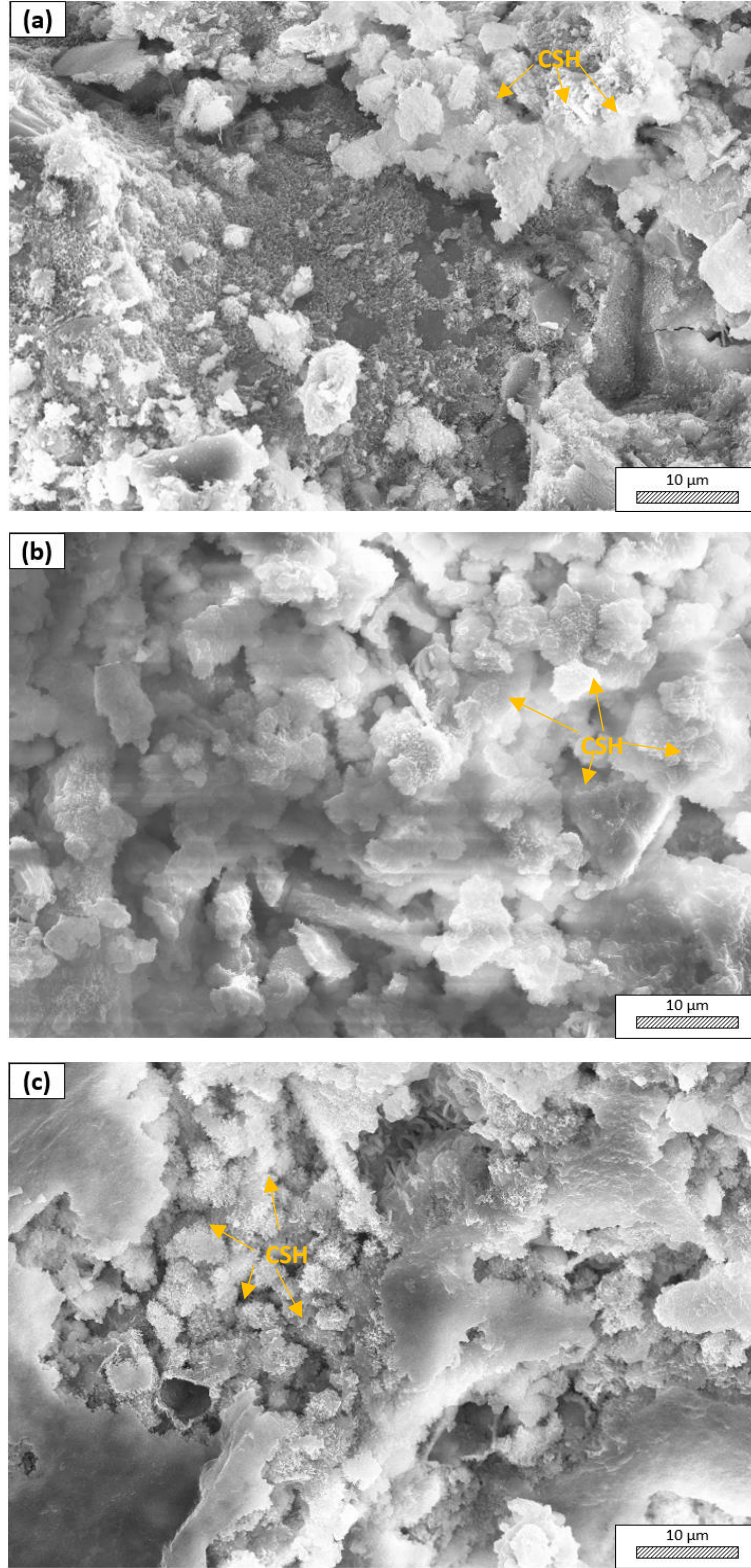
Şekil 3. 34. Eşit büyütmelerde (5.000x) alınmış mikroyapı görüntüleri; a) %5-600-FS-1s-suda – 7 gün, b) %15-600-FS-1s -suda – 7 gün c) %25-600-FS-1s -suda- 7 gün
