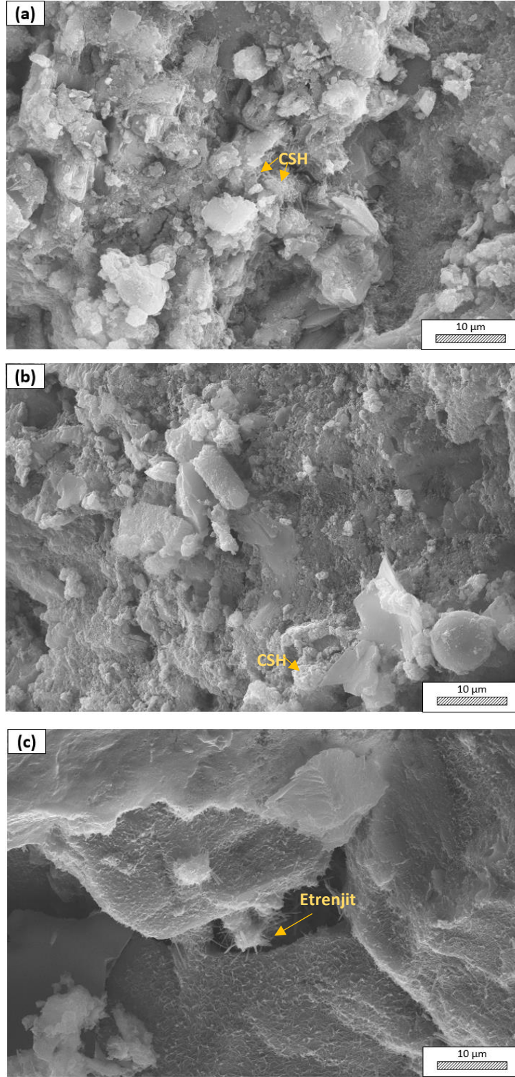
Şekil 3. 33. Eşit büyütmelelerde (5.000x) alınmış mikroyapı görüntüleri; a) Referans-suda – 7 gün, b) Referans-suda – 28 gün c) Referans-suda – 90 gün
