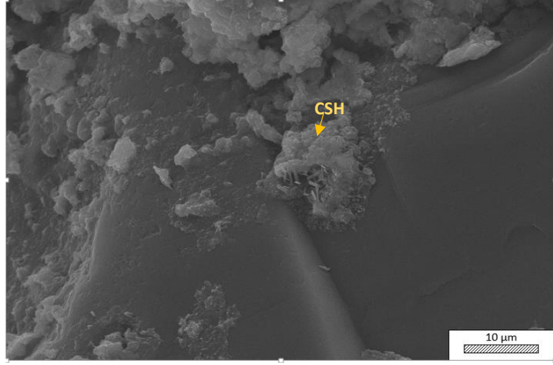
Şekil 3. 18. Eşit büyütmelerde (5.000x) alınmış mikroyapı görüntüleri; %15-400-AS-1s numunesi – 28 gün
