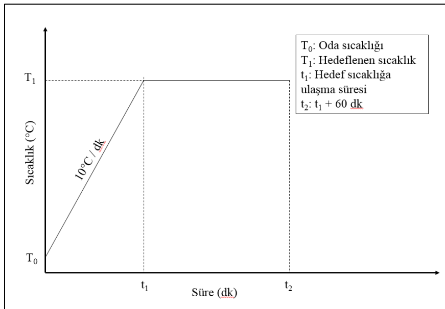
Şekil 2. 2. Bir saat ısıtma işlem uygulandıktan sonra ani soğutma (AS-1s) işlemine ait ısıtma işlem detayı
