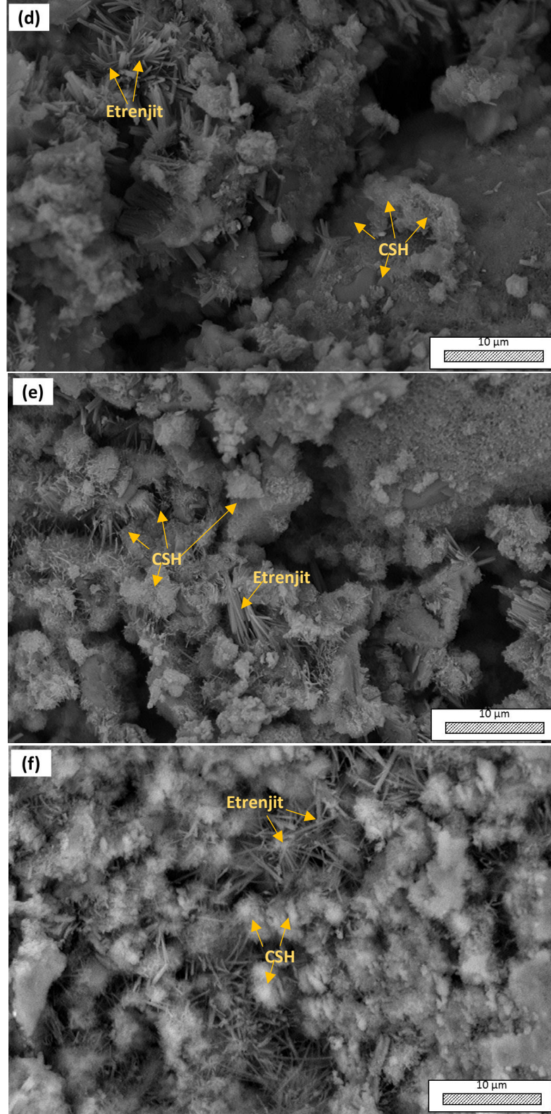
Şekil 3.15. (devam) 90 gün sonra dayanımları ölçülmüş numunelerden eşit büyütme (5.000x) alınmış mikroyapı görüntüleri; a) %15-400-FS-1s, b) %15-500-FS-1s, c) %15-600-FS-1s, d) %15-700-FS-1s, e) %15-800-FS-1s, f) %15-900-FS-1s
