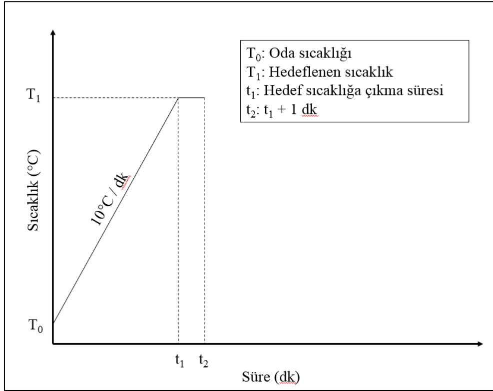
Şekil 2. 3. Bir dakika ısıt işlem uygulandıktan sonra ani soğutma (AS-1d) işlemine ait ısıt işlem detayı
