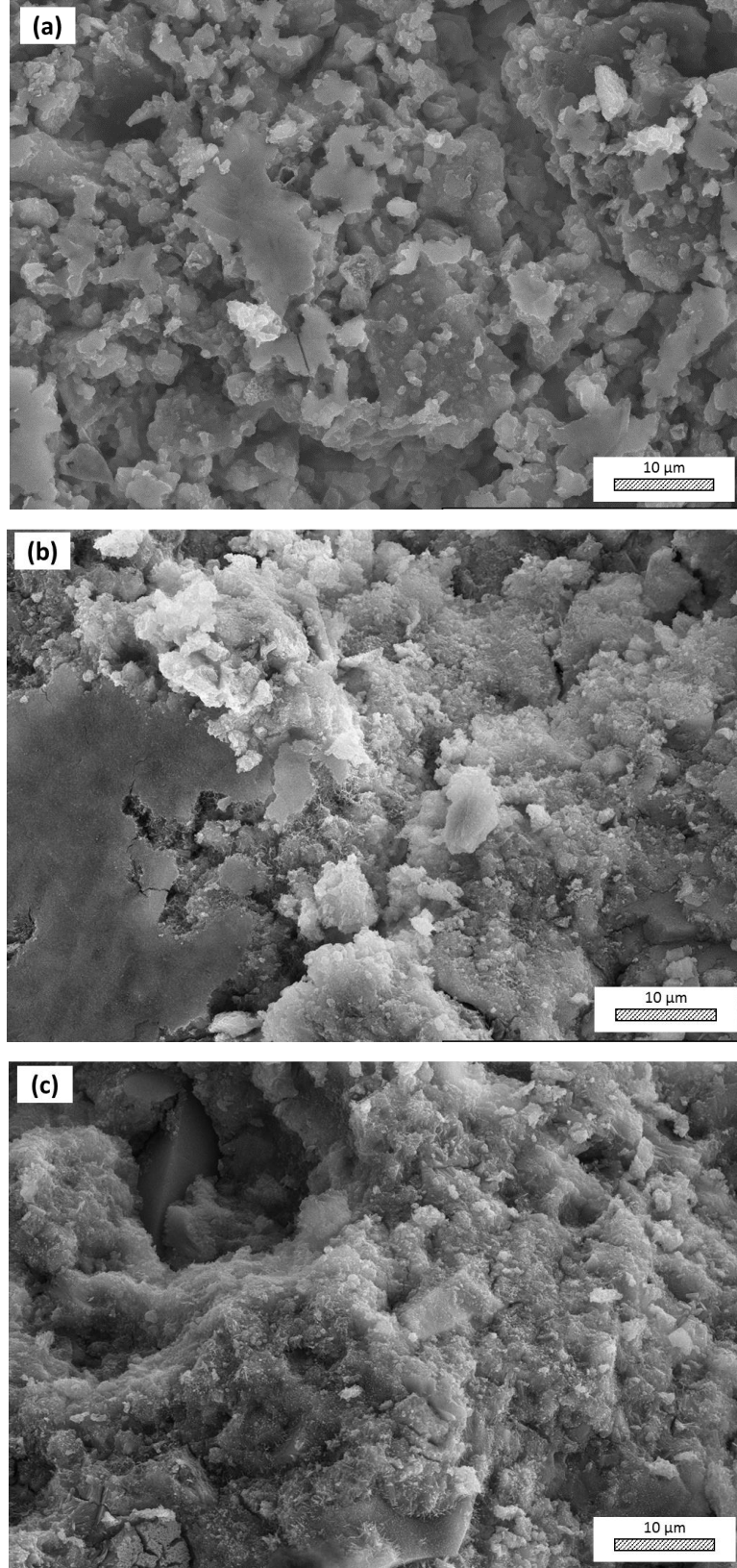
Şekil 3. 22. 28 gün sonra dayanımları ölçülmüş numunelerden eşit büyütmelerde (5.000x) alınmış mikroyapı görüntüleri a) %15-750-AS-1d, b) %15-780-AS-1d, c) %15-800-AS-1d
