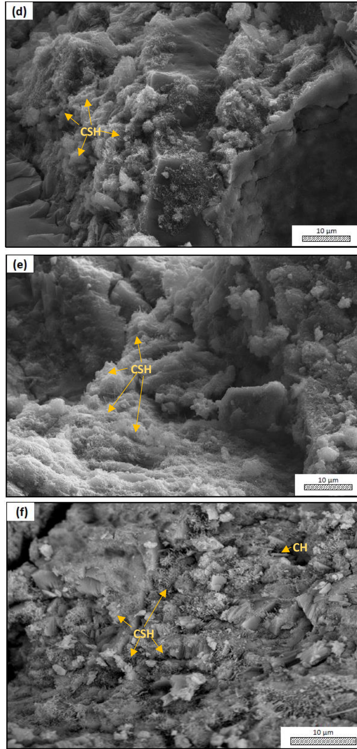
Şekil 3.14. (devam) 28 gün sonra dayanımları ölçülmüş numunelerden eşit büyütmelerde (5.000x) alınmış mikroyapı görüntüleri; a) %15-400-FS-1s, b) %15-500-FS-1s, c) %15-600-FS-1s, d) %15-700-FS-1s, e) %15-800-FS-1s, f) %15-900-FS-1s
