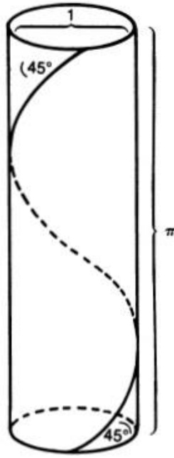
Şekil 2.5. Dairenin yuvarlanması (Rucker, 2005.)
