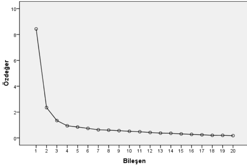
ÇizeneK 5: Açımlayıcı faktör analizine konu olan tüm bileşenlere ilişkin yamaç-birikinti grafiği
