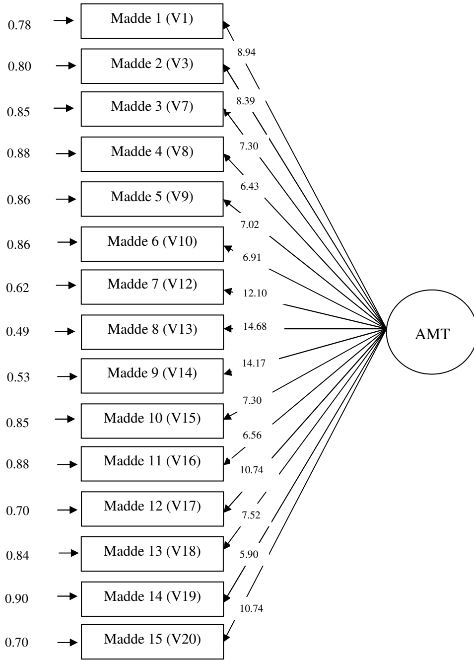
Çizene 6: AMT Ölçeği doğrulayıcı faktör analizi
