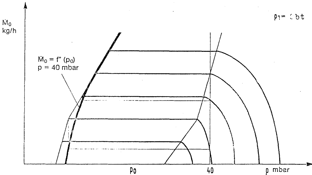
Şekil 3.10. M_o = f(P_o) P = sbt eğrisi
