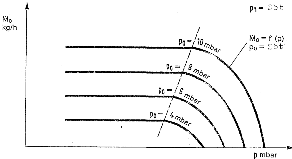
Şekil 3.8. M_0 = f(D) , P_0 = \text{sbt} eğrileri
