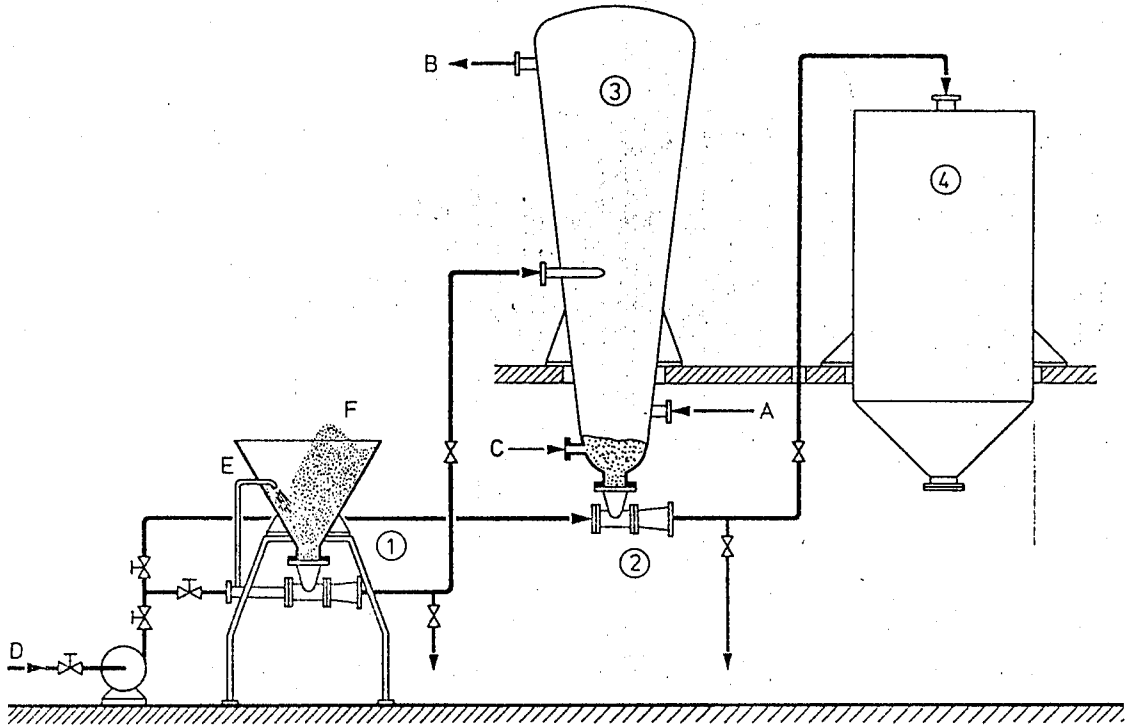
Şekil 2.4. Su jetli katı pompa (Wiegand, 1986)
