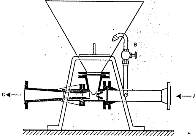
Şekil 2.4. Su jetli katı pompa (Wiegand, 1986)
