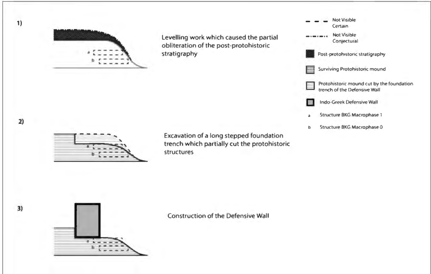
Resim 5. Bazira Sur Duvarı, Yapım Aşamaları ve Stratigrafisi (Iori, a.g.k. , 2018, 35, Fig. 1.14).
