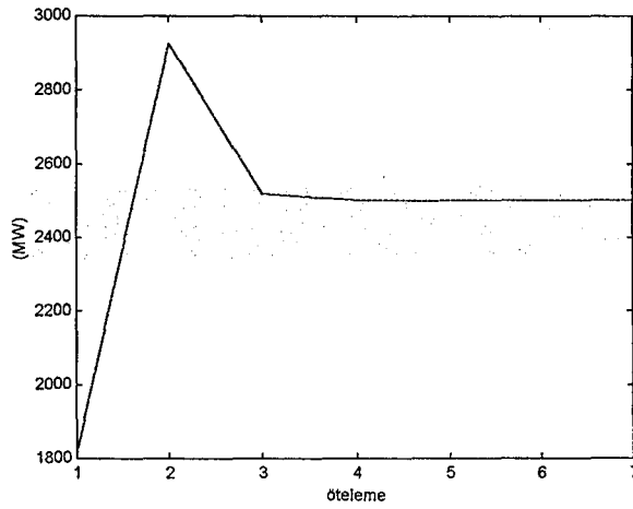
Şekil 5.38 Sistemdeki Toplam Güç Miktarının Öteleme Sayısına Göre Değişimi
