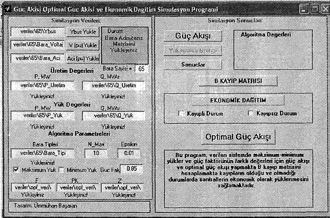
Şekil 5. 44 Güç Akışı, Optimal Güç Akışı ,Ekonomik Dağıtım Programlarının Arayüzü
