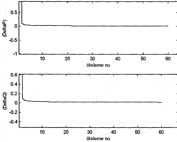
Şekil 5.14 \Delta P ve \Delta Q Değerlerinin Yakınsama Grafiği
