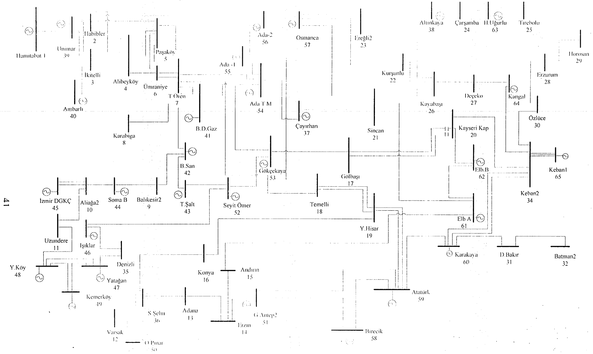
Şekil 5.10 Türkiye'deki 380 kV'luk 65 Baralı Sistem Şeması
