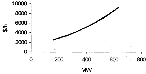
Şekil 5.29 Kemerköy Termik Santralinin Maliyet Eğrisi
