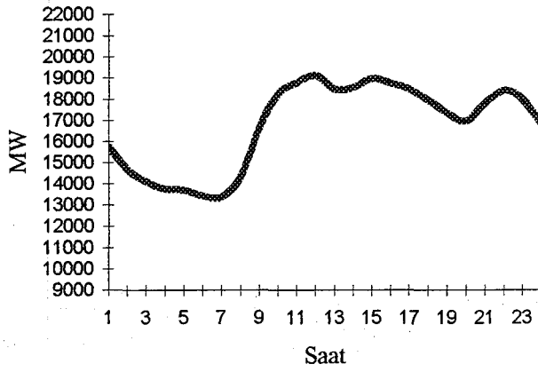
Şekil 2.2 Tüketici Bölgesinin Örnek Bir Günlük Yük Eğrisi (16.07.2003) [7]
