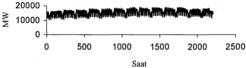
Şekil 5.4 Yaz Mevsiminde Yük Eğrisi
