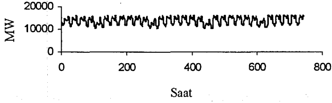
Şekil 5.2 Aylık Yük Eğrisi (Mayıs)
