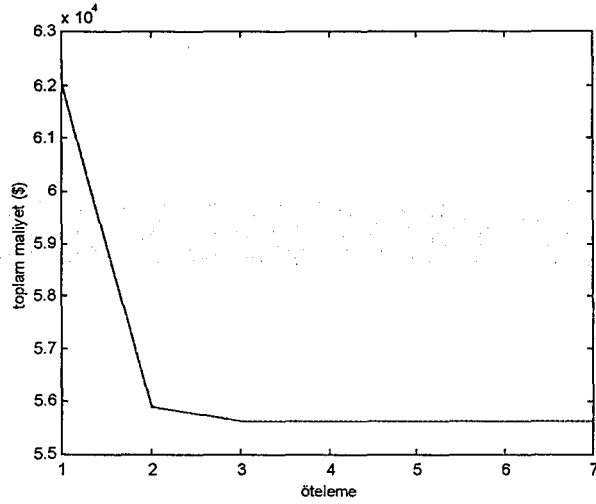
Şekil 5.40 Sistemin Toplam Maliyetinin Öteleme Sayısına Göre Değişimi Santrallerin çıkış güçleri aşağıda gösterilmiştir:
