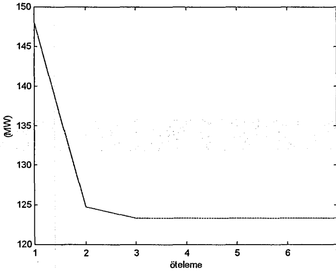
Şekil 5.32 Sistemdeki Kayıp Miktarının Öteleme Sayısına Göre Değişimi
