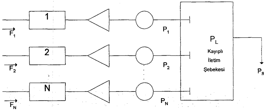
Şekil 4.3 P_R Yükünü Besleyen N Tane Termal Üretim Birimi
