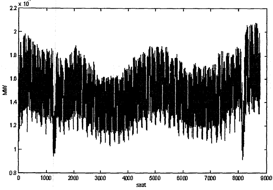
Şekil 5.7 Türkiye'de 2002 Yılı Yük Eğrisi
