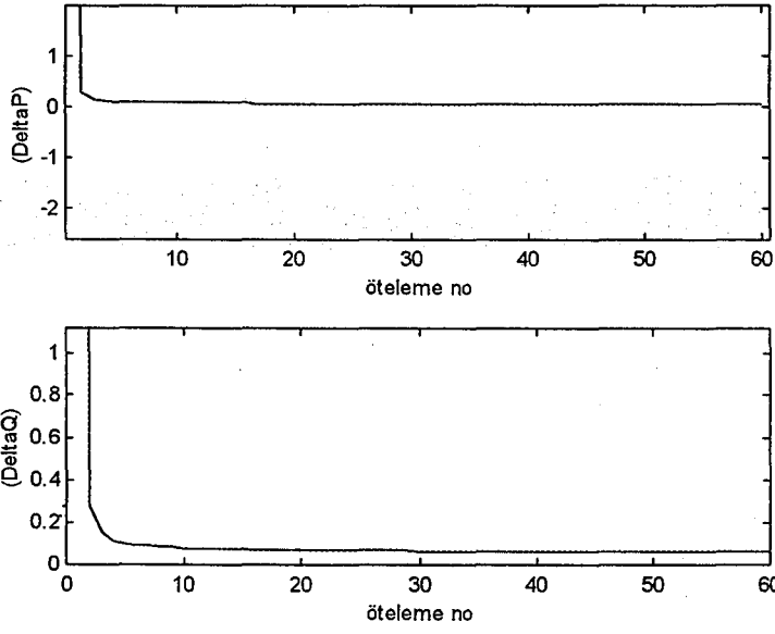
Şekil 5.16 \Delta P ve \Delta Q değerlerinin yakınsama grafiği
