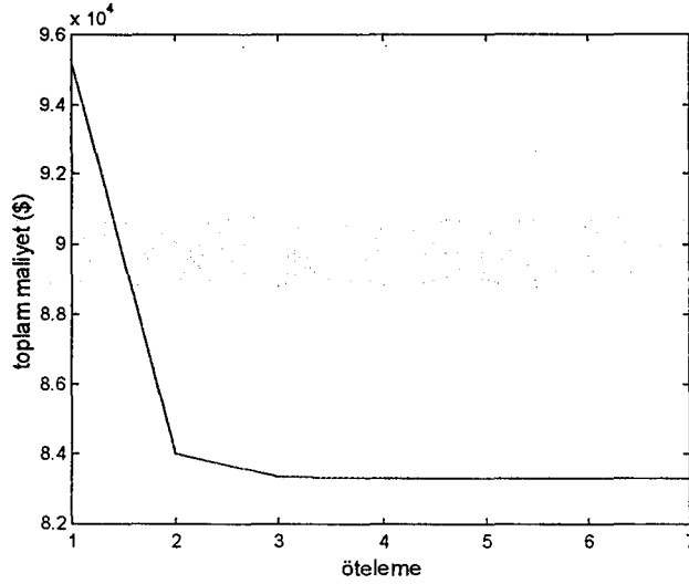
Şekil 5.35 Sistemin Toplam Maliyetinin Öteleme Sayısına Göre Değişimi Santrallerin çıkış güçleri aşağıda gösterilmiştir:
