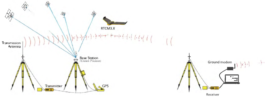
Şekil 3.5. RTK İHA platformları çalışma şekli ( http-24 )
