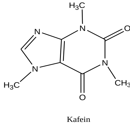
Şekil 4.1. Kafein molekülü
