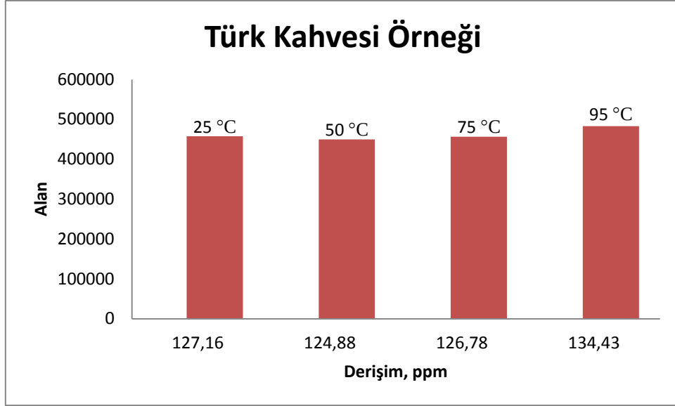
Şekil 5.10. Türk Kahve örneğindeki kafein miktarının sıcaklıkla değişimi
