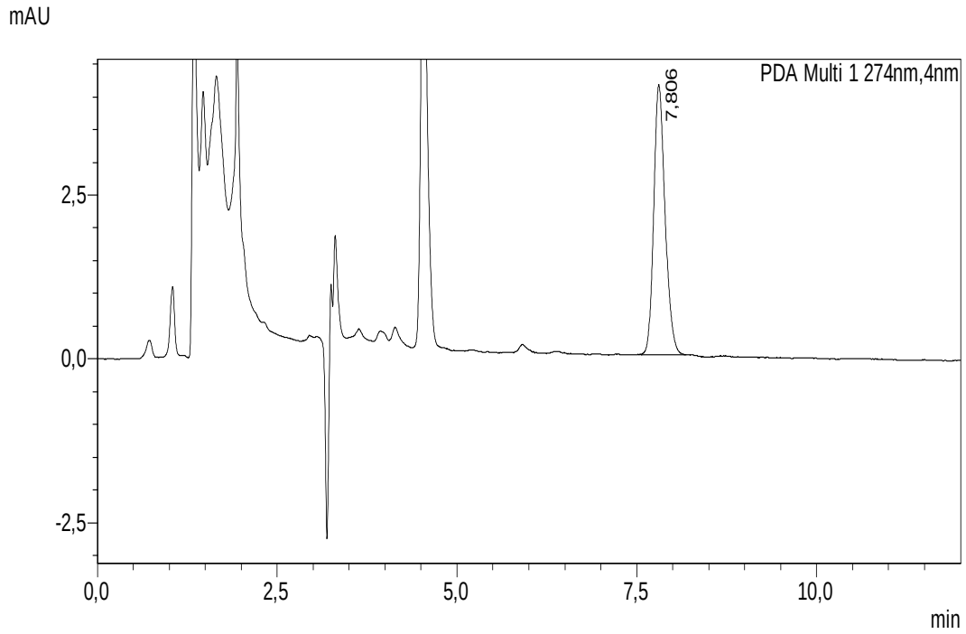
Şekil 5.3. 3 ü 1 arada kahve numunesinden elde edilen kromatogram
