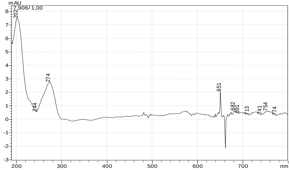
Şekil 5.1. 80 ppm derişime sahip kafein ile elde edilen DAD spektrumu
