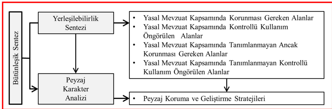
Şekil 5.1. Bütünsel sentez
