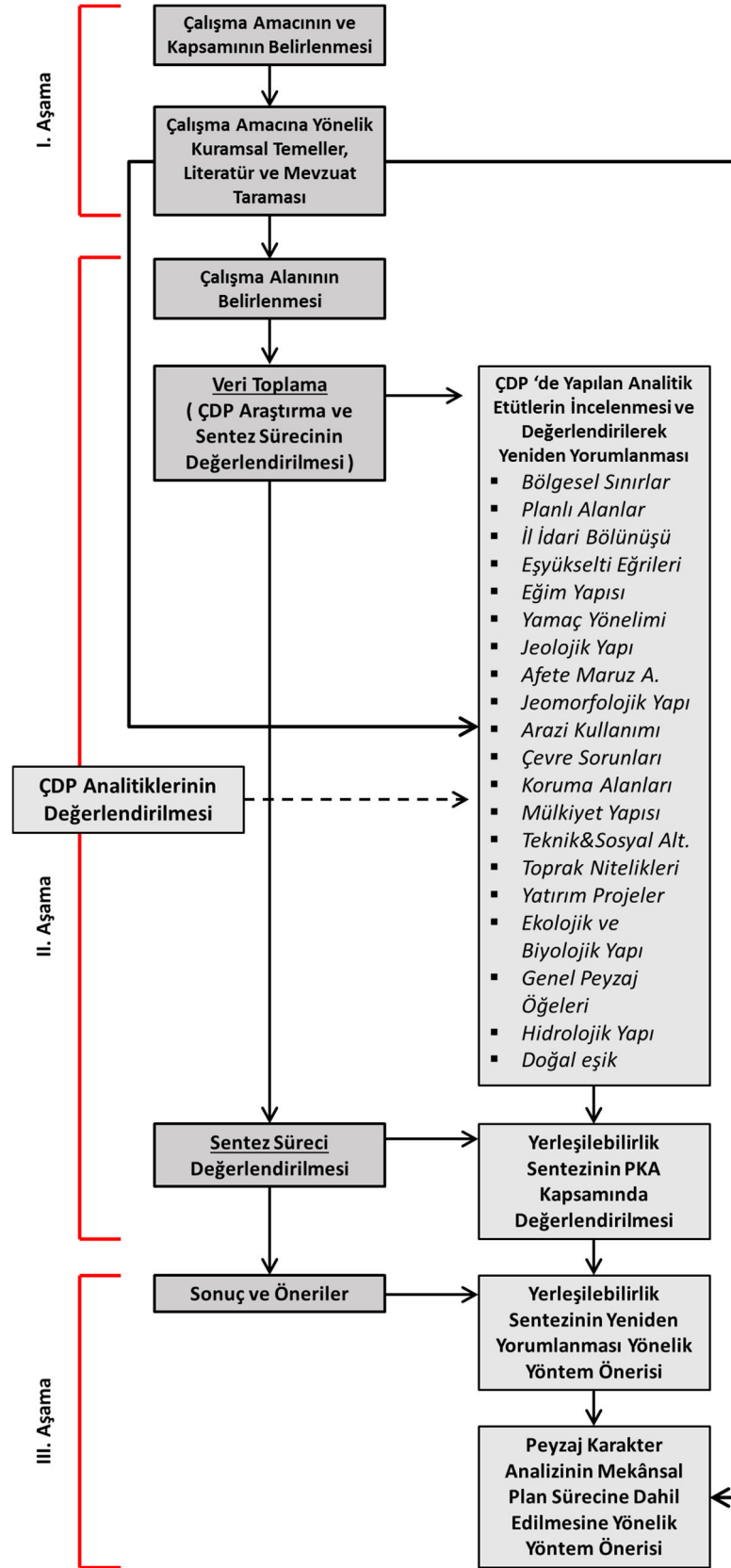
Şekil 3.1. Çalışmanın yöntemi
