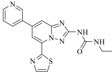
Şekil 2.20. 1-Etil-3-[7-(piridin-3-il)-5-(tiyazol-2-il)-[1,2,4]triazolo[1,5-a]piridin-2-il]üre
