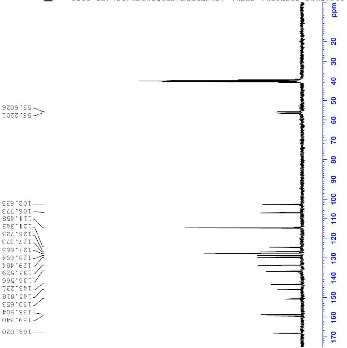
Şekil 5.31. Bileşik 4g'ye ait 13 CNMR spektrumu
