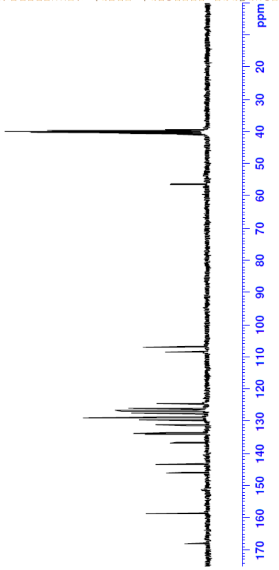
Şekil 5.55. Bileşik 4m'ye ait 13 CNMR spektrumu
