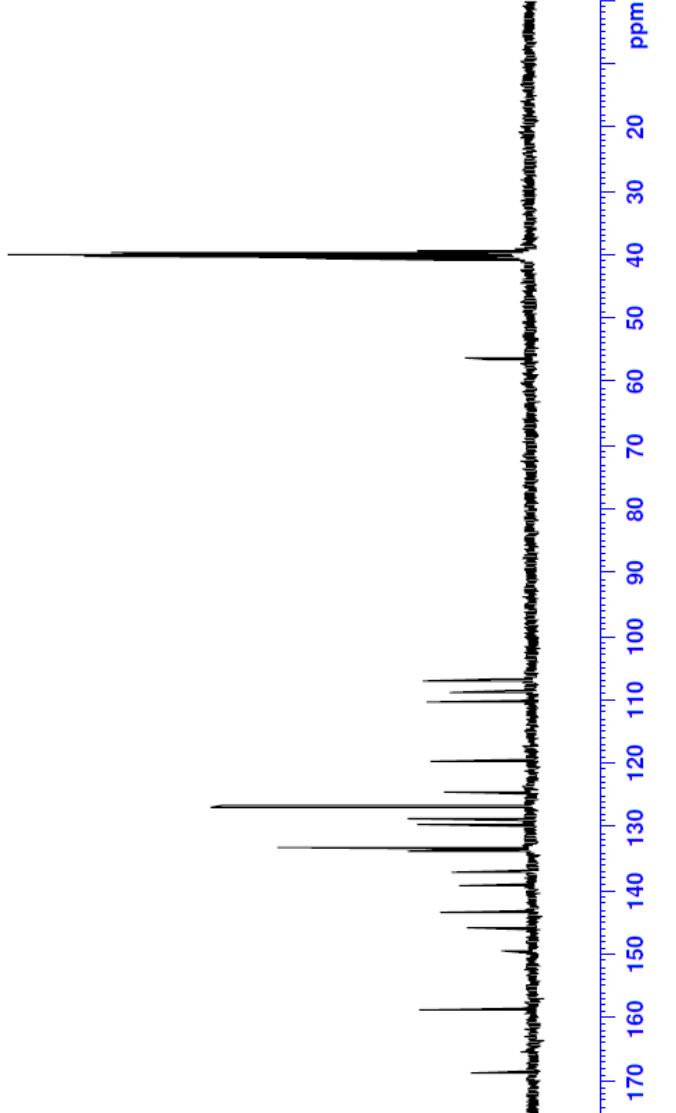
Şekil 5.23. Bileşik 4e'ye ait 13 CNMR spektrumu
