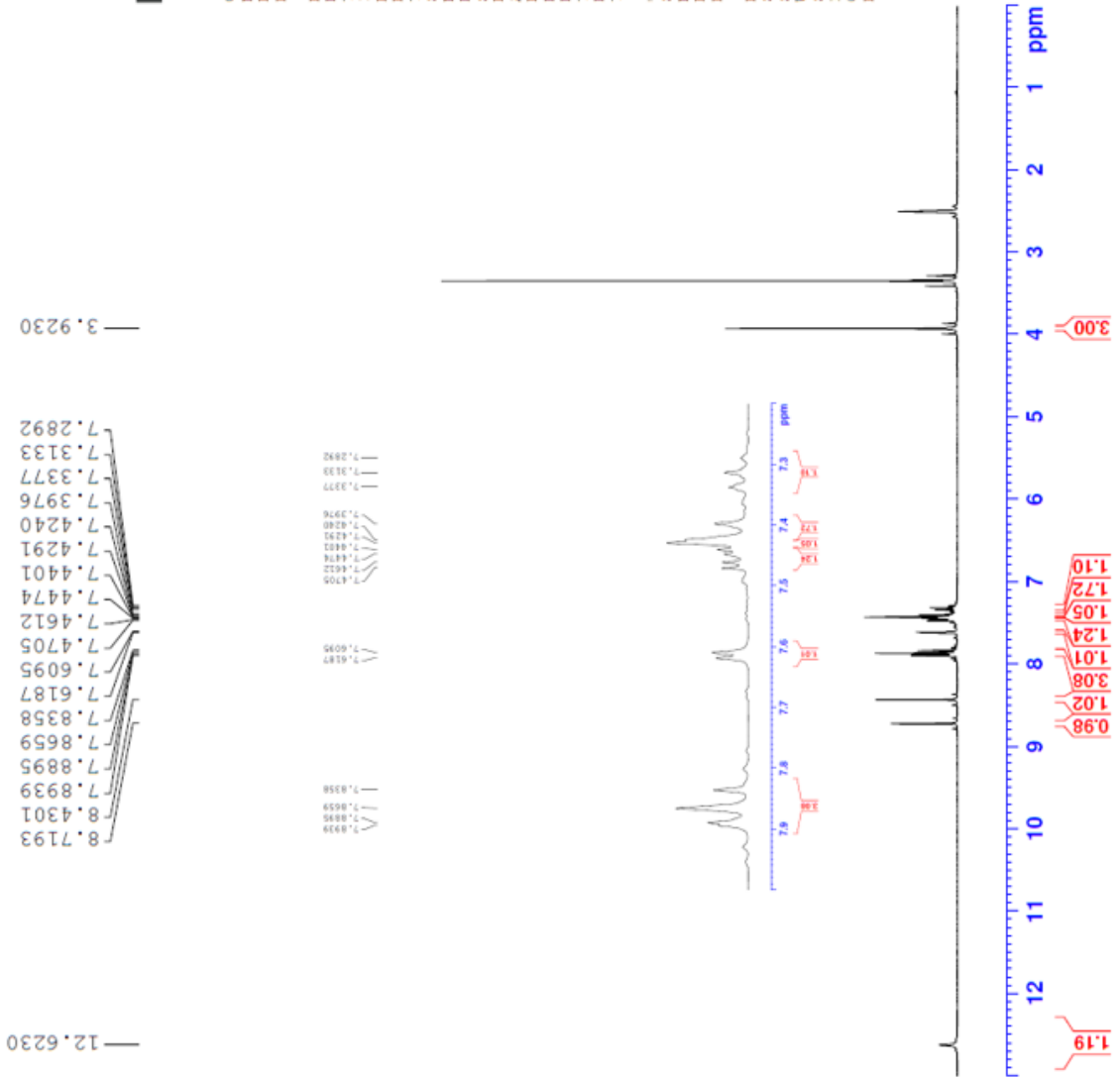
Şekil 5.18. Bileşik 4d'ye ait 1 H NMR spektrumu
