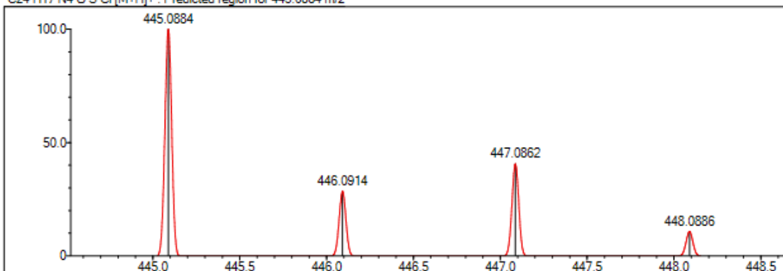
Şekil 5.56. Bileşik 4m'ye ait kütle spektrumu
