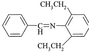
Şekil 50: Benziliden-2,6-dietilanilin
