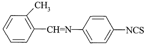
Şekil 24: N-(2-metilbenziliden)-4-tiyosiyanatoanilin
