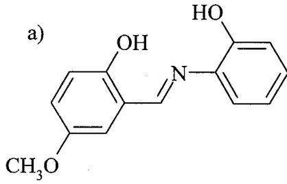
Şekil 79: a) N-(o-hidroksifenil)-5-metoksisalisilaldimin
