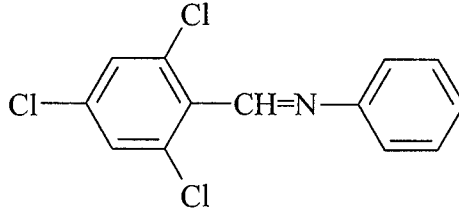
Şekil 10: 2,4,6-triklorobenzilidenanilin
