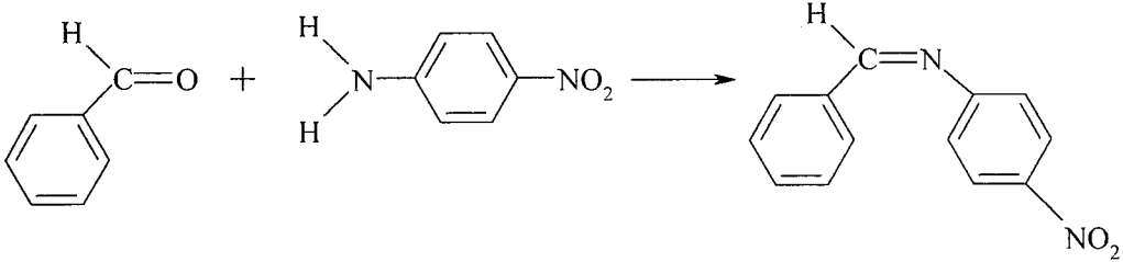
Şekil 60: Benziliden-p-nitroanilin eldesi
