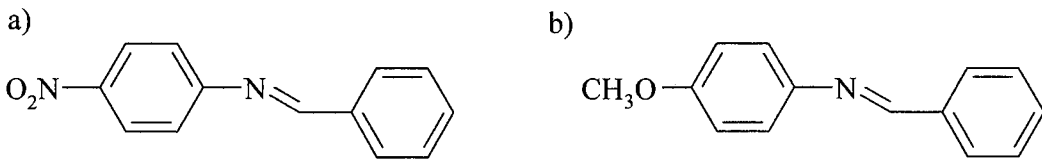
Şekil 44: a) N-benziliden-4-nitroanilin
