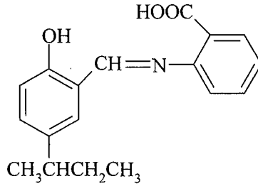
Şekil 73: 2-[2-hidroksi-5-(2-butilbenzilidenamino)]benzoikasit
