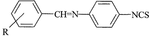
Şekil 20: Sübstitüe benzilidenanilin-4-tiyosiyanatoanilin
