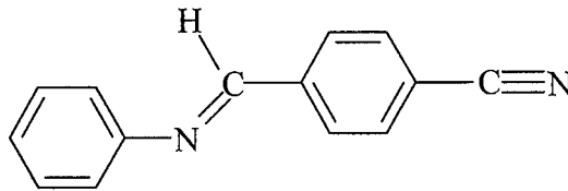
Şekil 74: N-(4-Siyanobenziliden)anilin
