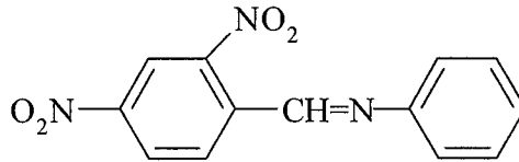
Şekil 6: 2,4-dinitrobenzilidenanilin
