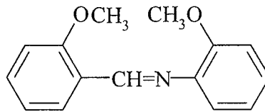
Şekil 23: o-anisiliden-o-anisidin
