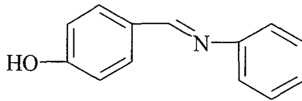
Şekil 8: 4-hidroksibenzilidenanilin
