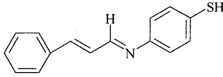
Şekil 82: N-sinnamiliden-2-merkaptanilin
