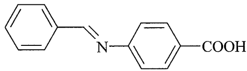
Şekil 29: 4-(N-benzilidenamino)benzoikasit
