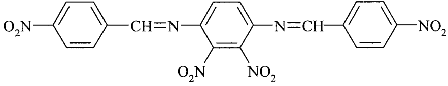
Şekil 14: N,N'-(4-nitrobenziliden)bis(2-nitroanilin)
