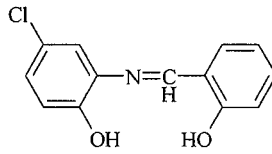
Şekil 75: N-(2-hidroksi-5-klorofenil) salisilaldimin
