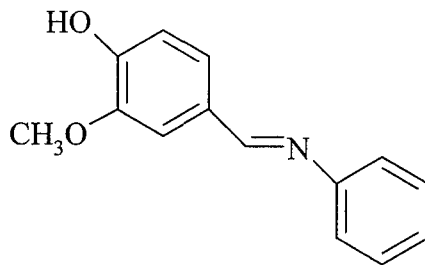
Şekil 31: 3-metoksi-4-hidroksibenzalanilin
