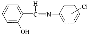
Şekil 85: N-süstitüe klorofenilsalisilaldimin
