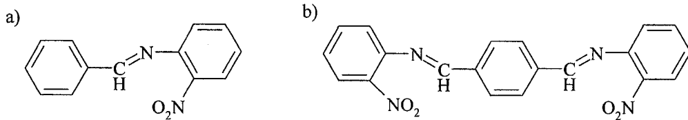
Şekil 21: a) N-benziliden-o-nitroanilin
