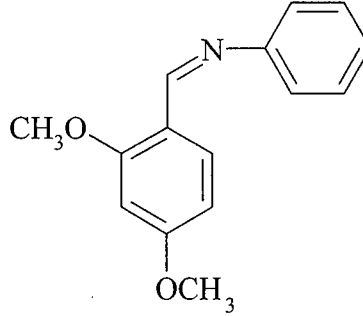
Şekil 56: 2,4-dimetoksibenzilidenanilin
