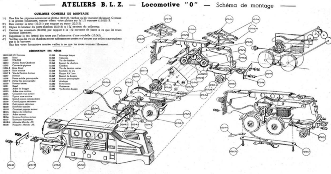
Görsel 3.24 Oyuncak bir lokomotifin montaj şeması. ( http-3 )
