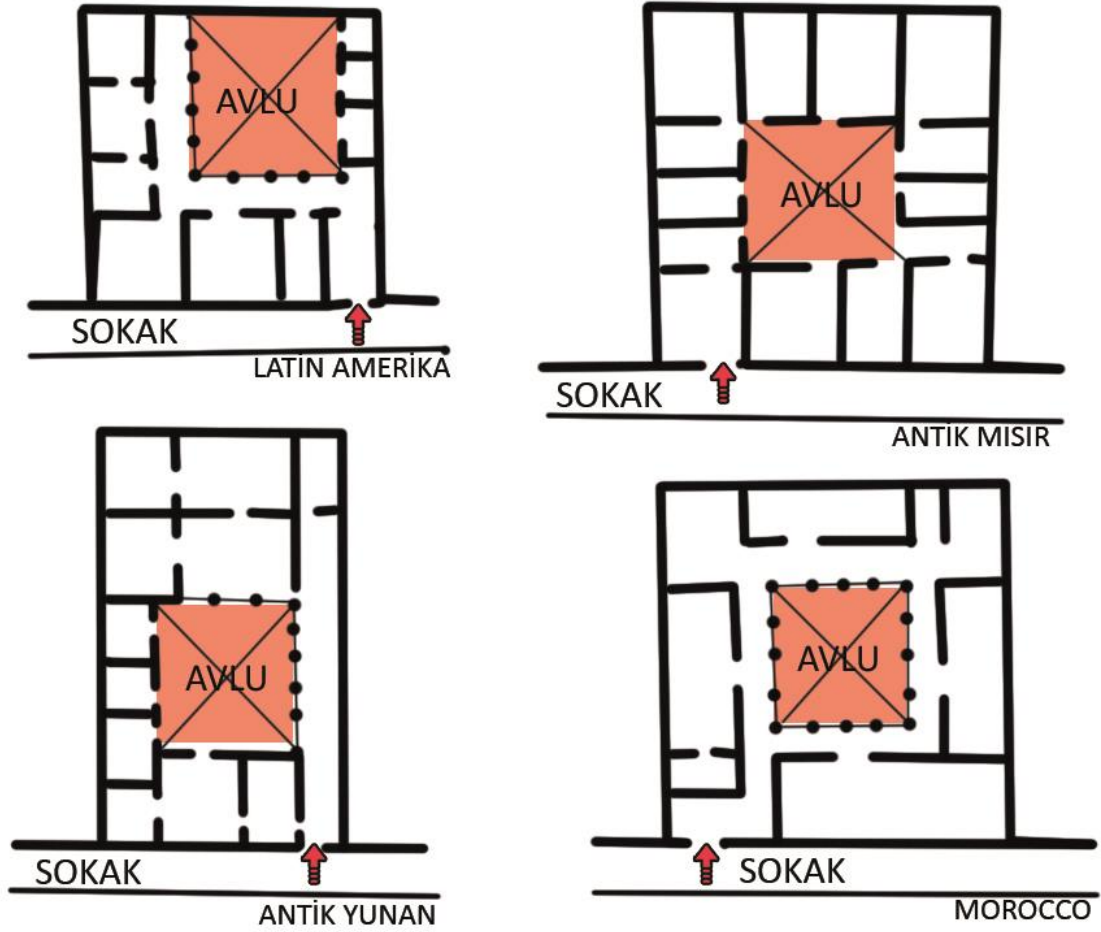
Şekil 4. 10. Dört farklı bölgeye ait benzer prensipler ile tasarlanan avlu örnekleri (Rapoport, 1969'dan faydalanılarak hazırlanmıştır.)
