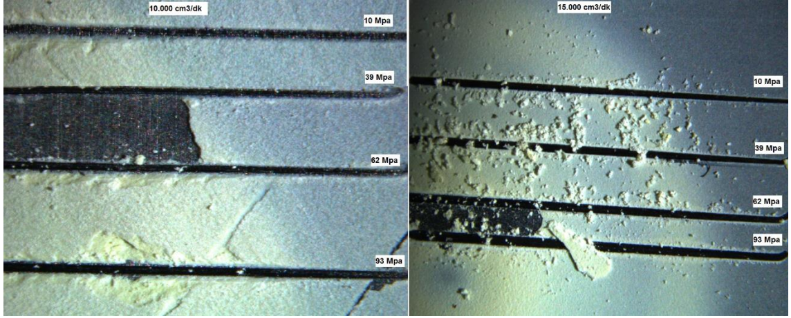
Şekil 3.28. Farklı gaz akışında ( 1.000, 5.000, 10.000, 15.000 \text{ cm}^3/\text{dk} ) yapılan kaplamaların çizik test optik görüntüleri
