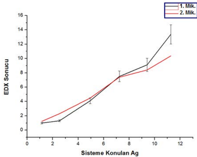
Şekil 2.23. Başlangıç Ag miktarı ile karakterizasyon sonrası okunan Ag miktarlarının karşılaştırılması
