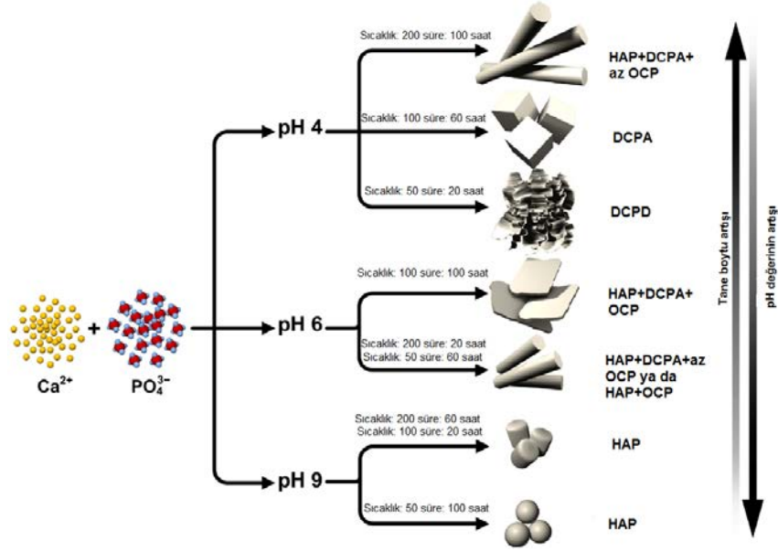
Şekil 2.6. Sıcaklığın, pH'ın ve hidrotermal sürenin CaP tozunun faz, morfoloji ve tane boyutuna etkisi
