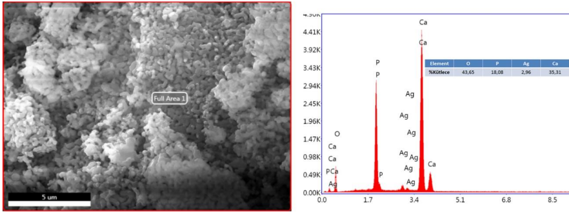
Şekil 2.25. Son pH değeri 8.5 olarak sentezlenen tozun a) kalsinasyon öncesi b) kalsinasyon sonrası kimyasal analiz sonucu
