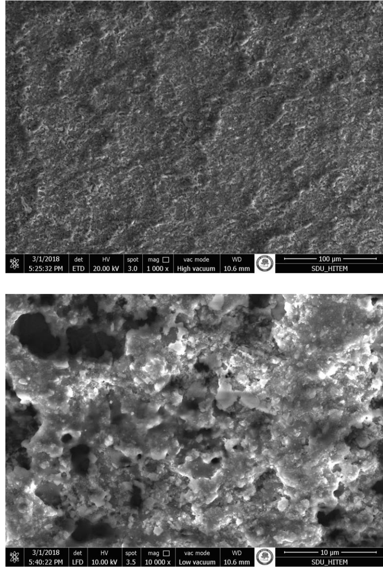
Şekil 4.15. Isıl işlem sonrası metal implant yüzeyinde bulunan kaplamanın mikro yapısı
