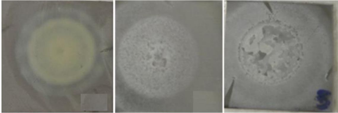
Şekil 3.5. 3 farklı toz ile kaplanan altlıkların görüntüleri ( 0,06\ \mu\text{m} , 0,2\ \mu\text{m} ve 0,8\ \mu\text{m} )
