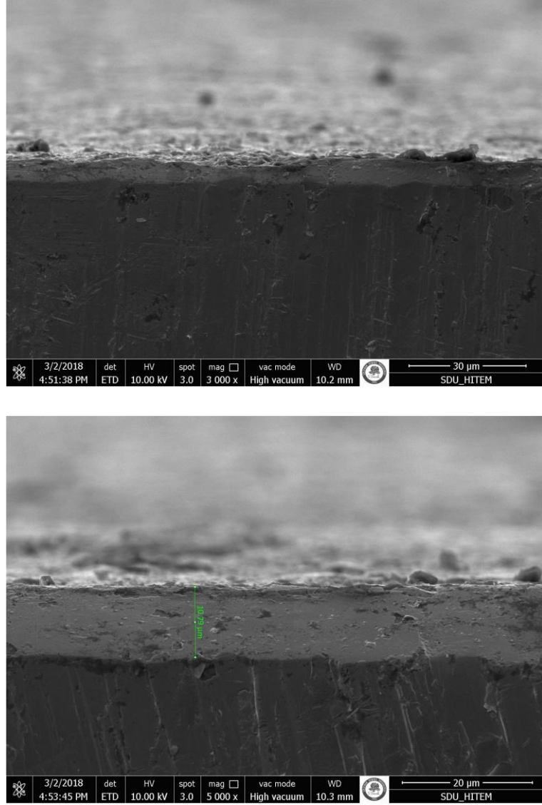
Şekil 4.16. Metal implantın ve kaplamanın ara yüzeyinden alınan SEM görüntüleri
