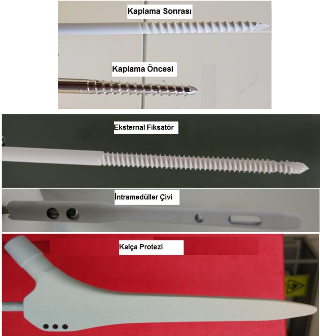
Şekil 4.6. Elektro spreyl yöntemi ile kaplanan metal implantların görüntüsü
