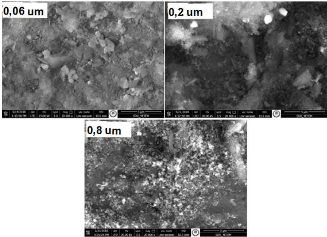
Şekil 3.7. 0,06-0,2 ve 0,8 µm tane boyutuna sahip tozlar ile yapılan kaplamaların mikro yapı görüntüleri
