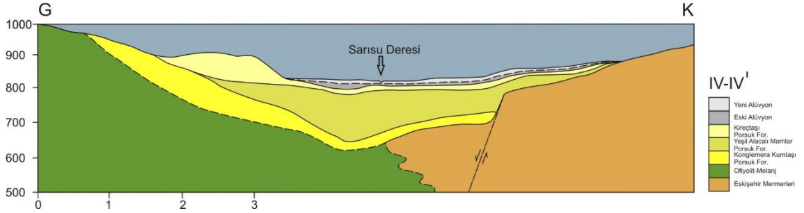
Şekil 3.8. IV-IV' - GGD-KKB kesiti (DSİ, 1976'dan geliştirilmiştir, Güney vd., 2014)
