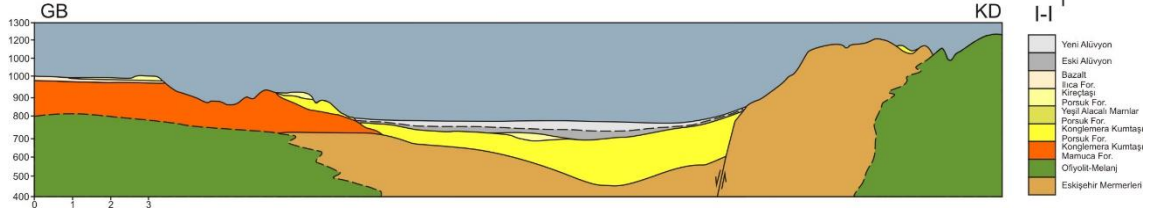
Şekil 3.5. I-I' - GB-KD kesiti (DSİ, 1976'dan geliştirilmiştir, Güney vd., 2014)
