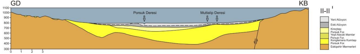
Şekil 3.6. II-II' - GD-KB kesiti (DSİ, 1976'dan geliştirilmiştir, Güney vd., 2014)
