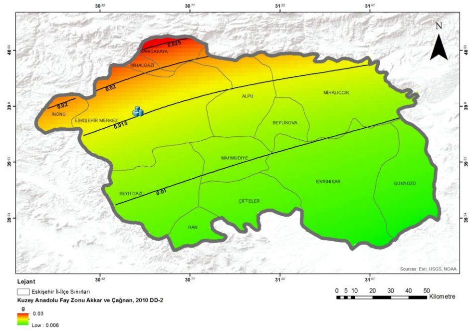
Şekil 6.25. KAFZ Akkar ve Çağnan, (2010) azalım ilişkisi STA haritası (DD-2, 50 yılda %10 aşılma olasılığı ve 475 yıllık tekrarlanma periyodu)
