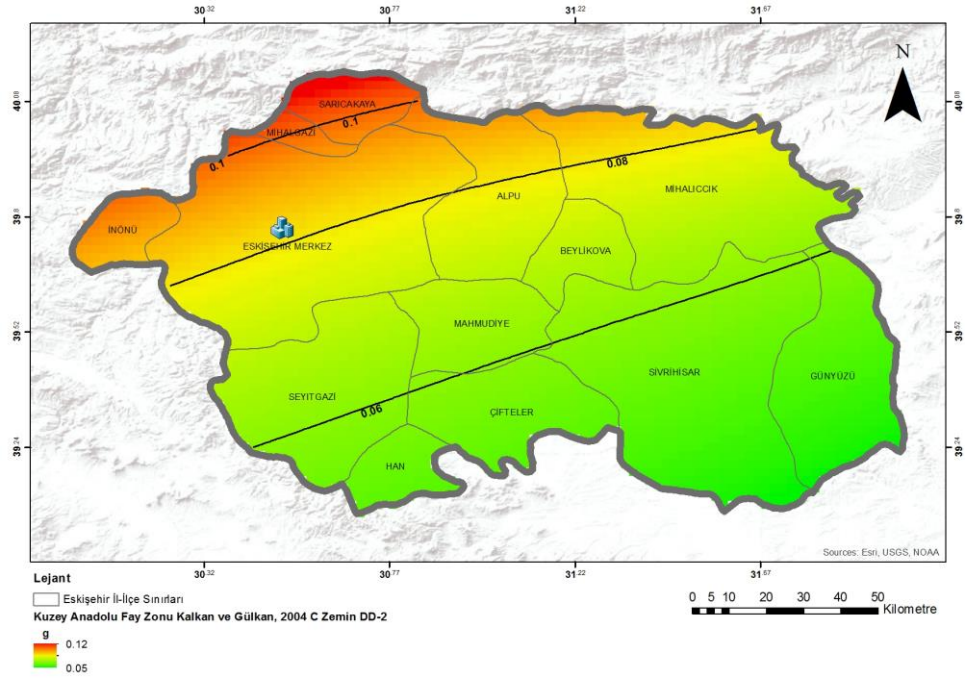
Şekil 6.14. KAFZ Kalkan ve Gülkan, (2004) azalım ilişkisi C zemin sınıfına göre STA haritası (DD-2, 50 yılda %10 aşılma olasılığı ve 475 yıllık tekrarlanma periyodu)
