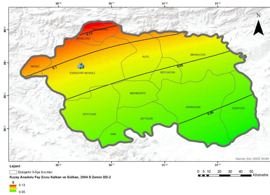
Şekil 6.15. KAFZ Kalkan ve Gülkan, (2004) azalım ilişkisi D zemin sınıfına göre STA haritası (DD-2, 50 yılda %10 aşılma olasılığı ve 475 yıllık tekrarlanma periyodu)
