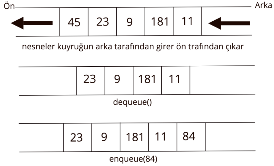
Şekil 3. 7. Kuyruk veri yapısı
