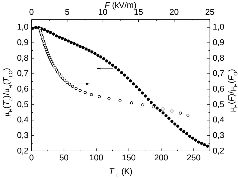
Şekil 4.4. \text{Al}_{0,25}\text{Ga}_{0,75}\text{N}/\text{AlN}/\text{GaN} heteroeklem örnekte sıcaklığa ve elektrik alana bağlı normalize edilmiş mobilitelerin karşılaştırılması. İçi dolu daireler normalize edilmiş mobilitenin sıcaklıkla değişimi ve içi boş daireler normalize edilmiş mobilitenin uygulanan elektrik alan ile değişimidir.
