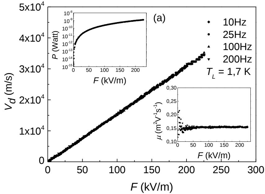
Şekil 4.15. \text{Ga}_{0,7}\text{In}_{0,3}\text{N}_{0,004}\text{As}_{0,996}/\text{GaAs} kuantum kuyu örnekte sürüklenme hızının, mobilitenin ve elektron başına güç kaybının elektrik alanla değişimlerinin a)1,7 K, b)50 K, c)100 K, d)150 K, e)200 K, f)250 K, g)300 K'deki uygulanan voltajın frekansına bağlı değişimleri
