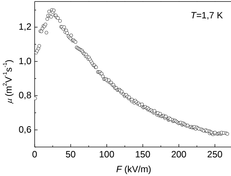
Şekil 4.10. \text{Al}_{0.83}\text{In}_{0.17}\text{N}/\text{AlN}/\text{GaN} heteroeklem örnekte mobilitenin uygulanan elektrik alan ile değişimi ( T=1,7 K)
